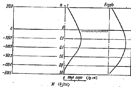
図-15 M (kg/cm)
