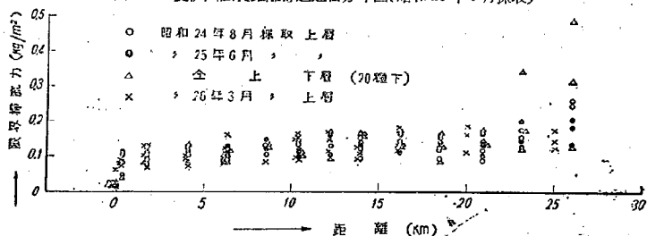
図—14 限界掃流力変化図
