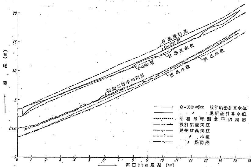
図一18 斐伊川縦断面図
