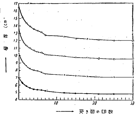
図-5 突き固メ回数と層厚との関係
