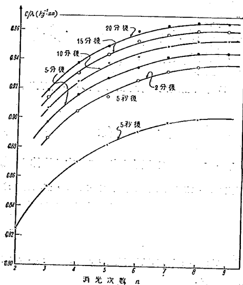
附図-1 フェノライトの光弾性感度に対する消光次数 n の影響
