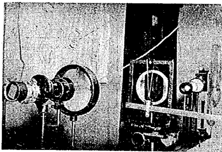
附写真-1 試験片形状および測定装置
