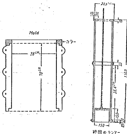
図-2 モールド並びに突き固め用ランマー
