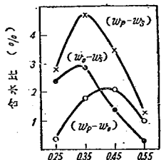
図-11 (w_0 - w_p) , (w_p - w_s) , (w_0 - w_s) と n の間の関係
