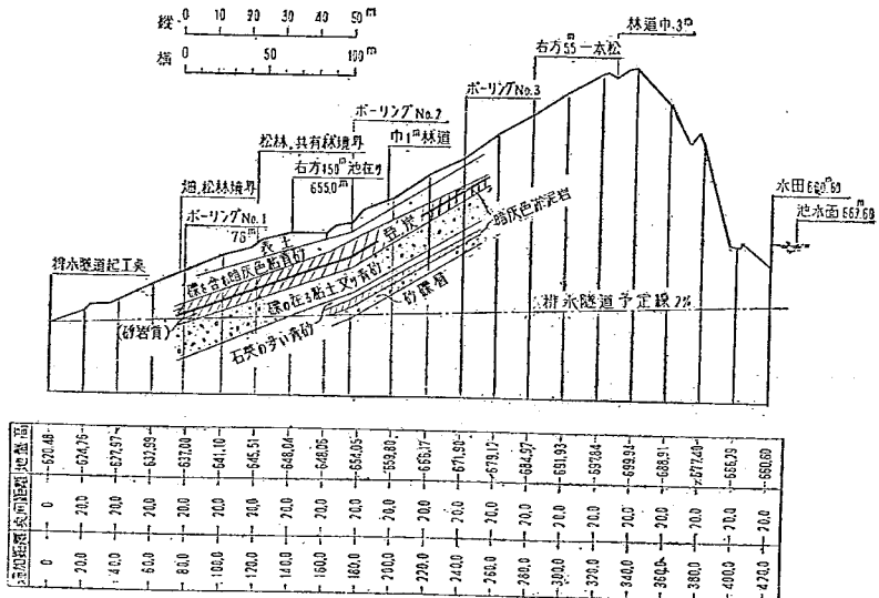
図-5 有旅側頂上排水トンネル縦断地質図
