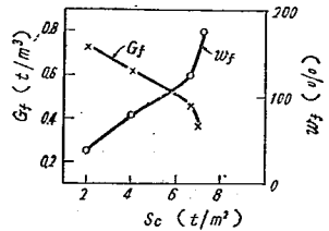
図-9 最適含水比における強度 S_c と細粒部分の乾燥密度 G_0 と並びに含水比 w_f の間の関係
