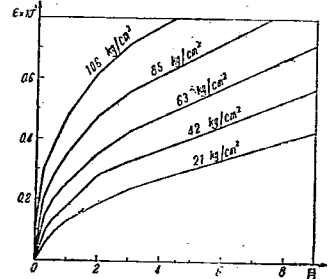
図-8 コンクリート偏屈曲線
