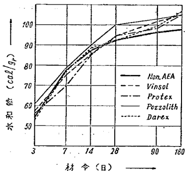
図-1 普通セメント水和熱
