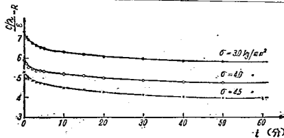
図-7 光弾性感度と歪に対する負荷時間の影響
