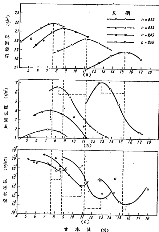
図-6 軽メ固メの含水比と乾燥密度、圧縮強度、透水性係数の関係
