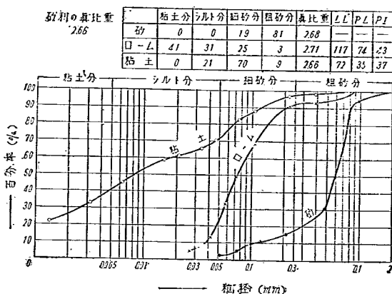
図-1B 原材料の性質
