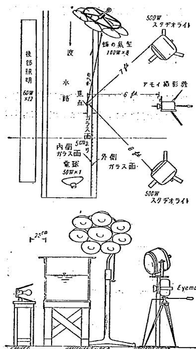
図-2 ライトの配置とカメラの位置
