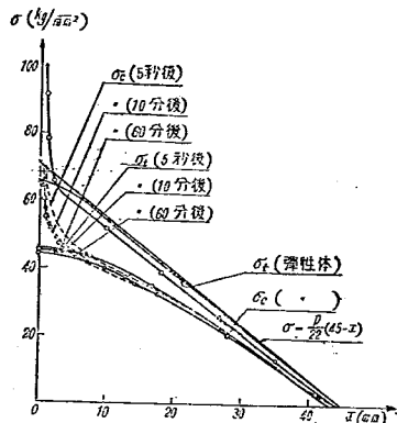
図-9 (b) 弾性体と塑性体（メタクリル酸樹脂）に於ける繰応力
