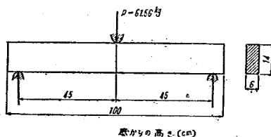
図-9 (a) 供試体寸度と負荷要領
