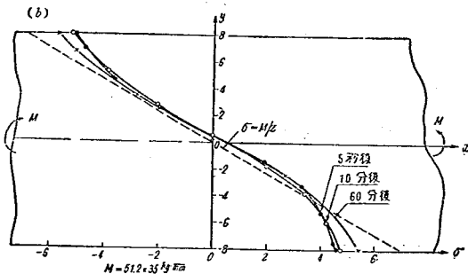
図-10 (b) 矩形梁の純粋曲げの場合
