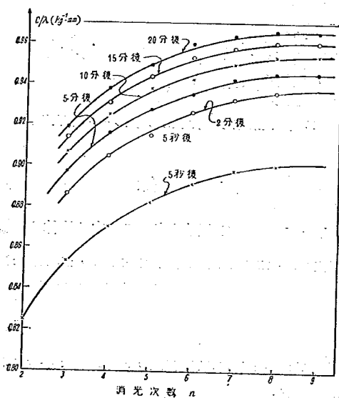
附図一 フェノライトの光弾性感度に対する消光次数 n の影響
