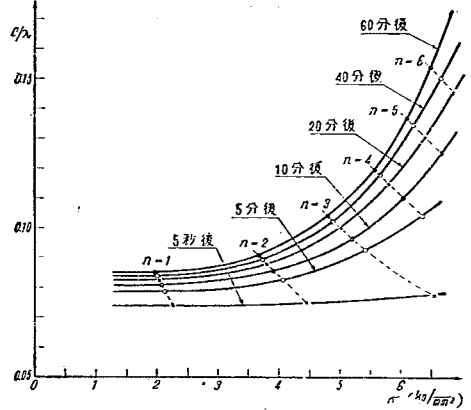
図-5 b. 光弾性感度 c/l に対する圧縮応力と負荷時間の関係 (室温 28^{\circ}\text{C} )
