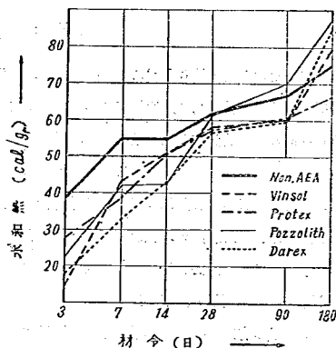
図-5 シリカセメント水和熱
