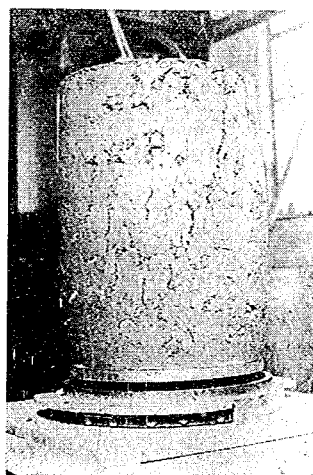
写真-2 圧縮試験終了後の供試体 ( n=0.25 w=17\% )
