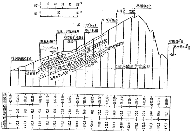
圖一5 有旅側頂上排水隧道縱斷地質圖
