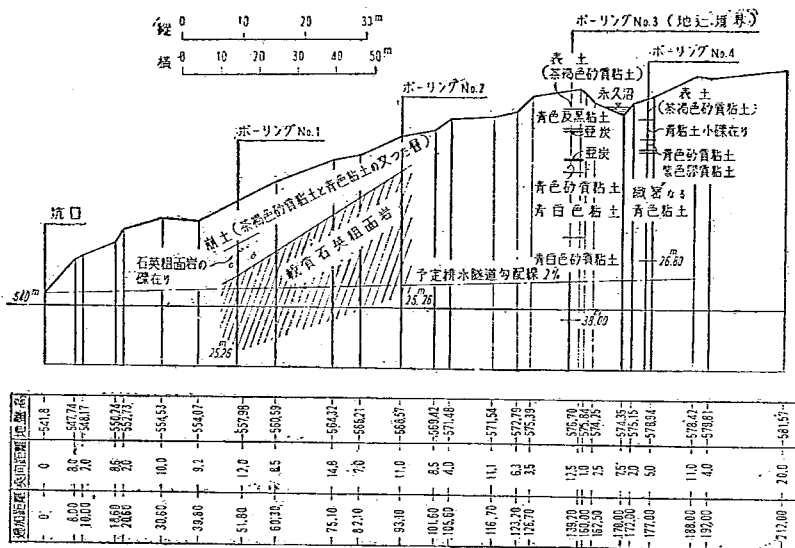
図-3 宇土沢排水隧道地質図
