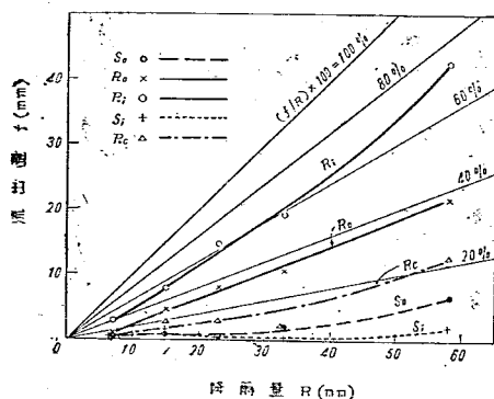
図一20 降雨量と流出量との関係
