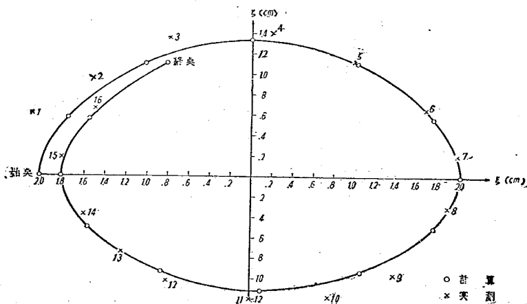
図-5 (c) 実測軌道と理論軌道との比較 (例3)
