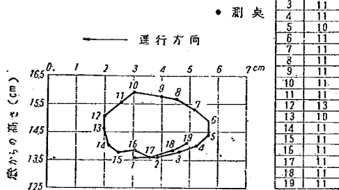
図-4 (a) 水分子軌道実測図 (例 2)
