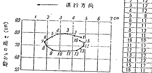
図-6 (a) 水分子軌道実測図 (例 4)
