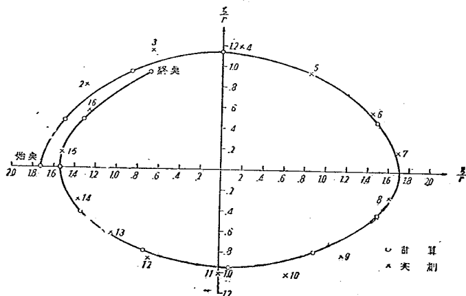
図-5 (b) 実測軌道と理論軌道との比較 (例3)
