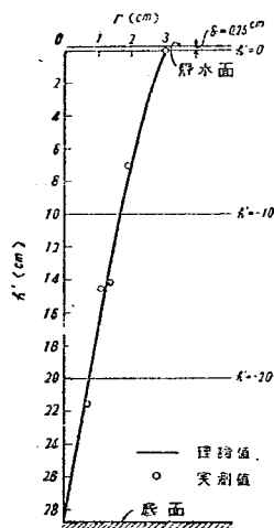
図-7 半波高( r )の実測値と理論値との比較
