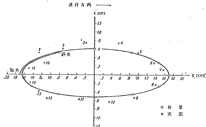
図-6 (b) 実測軌道と理論軌道との比較 (例 4)
