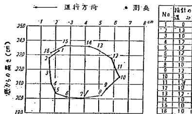
図—3 (a) 水分子軌道実測図 (例 1)
