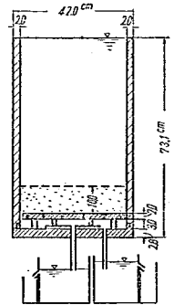
図-4 透水試験装置
