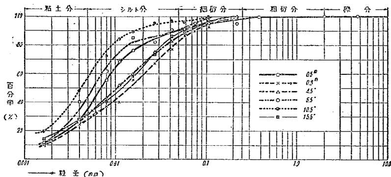
図-2 粒径加積曲線
