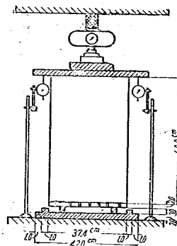
図-3 圧縮試験装置
