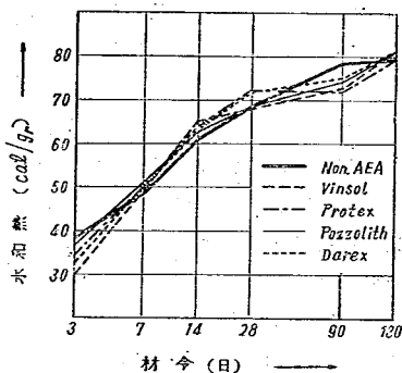
図-3 低熱セメント水和熱
