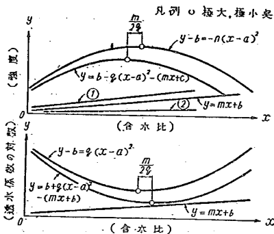
図-12 最大強度、最小透水係数を与える点が最適含水比をあたえる点と一致しないことを示す図
