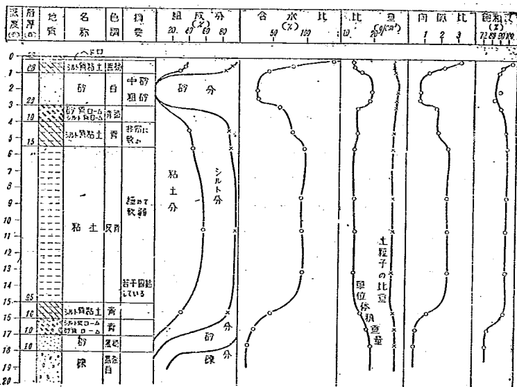
図—10 土質試験成績(0表の土)
