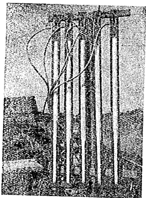
写真—6 間隙水圧計のマノメータ
