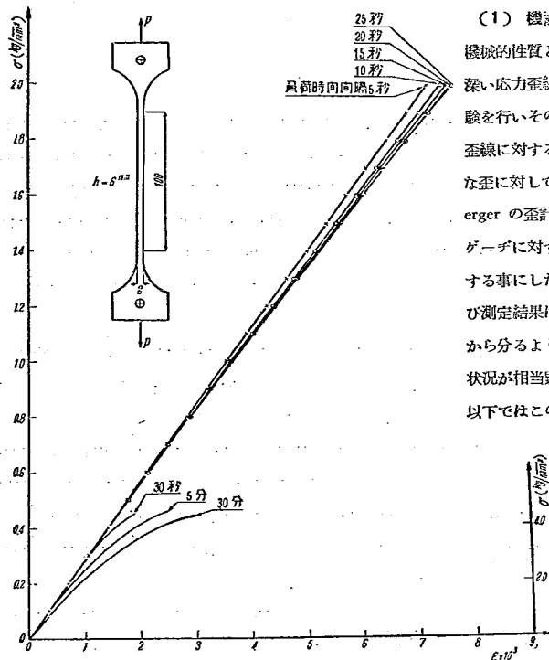
図一 負荷時間々隔の曲線 \sigma \sim \epsilon 曲線に及ぼす影響 (室温 28°C)
