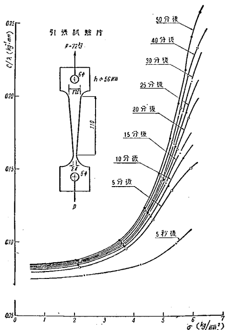
図—3 光弾性感度に対する引張応力と負荷時間の関係 (室温 28°C)
