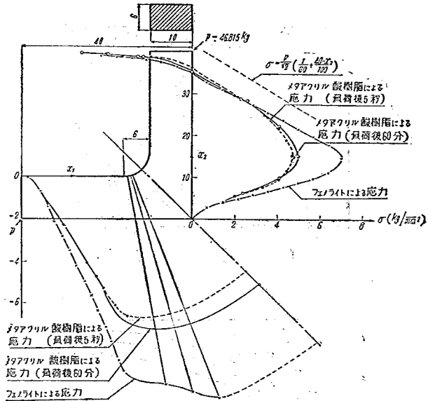
図-13 曲げと圧縮を同時に受ける場合ラメーン隅角部附近の応力
