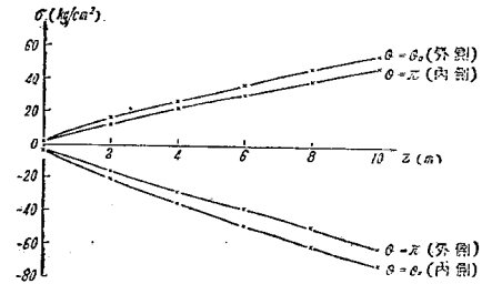
図-7 地盤地み高さ z と橋立応力 \sigma との関係
