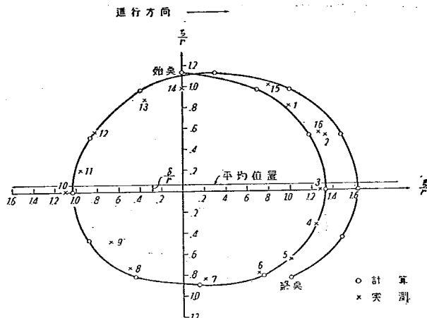
図-3 (b). 実験軌道と理論軌道との比較 (例1)
