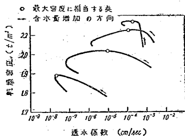
図-8 乾燥密度と透水係数との関係
