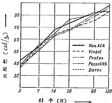
図-2 中庸熱セメント水和熱
