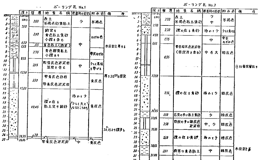
図-3 宇土沢排水隧道地質図
