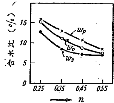
図-10 最適含水比 w_0 , 最大強度を与える含水比 w_c , 最小透水係数を与える含水比 w_p と n との関係
