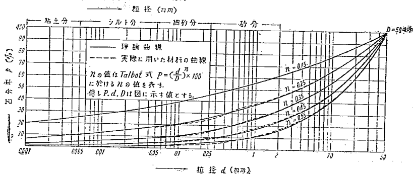
図-1A 試験に用いた材料の粒径加減曲線
