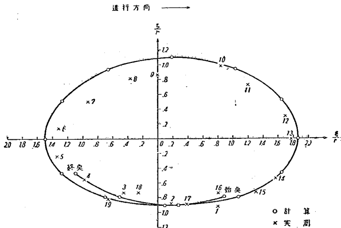
図-4 (b) 実測軌道と理論軌道との比較 (例 2)
