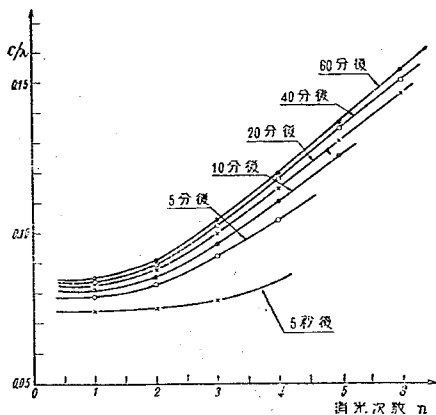
図-6 圧縮時に於ける光弾性感度 c/\lambda に対する消光次数 n および負荷時間の関係 (室温 28^{\circ}\text{C} )
