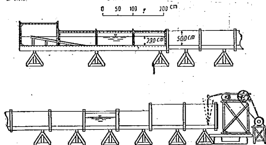
図-1 実験水路
