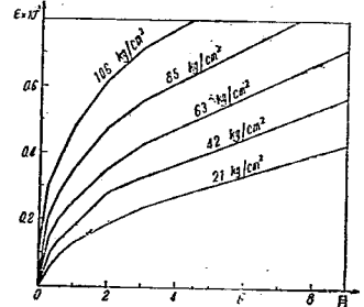
図-8 コンクリート偏屈曲線
