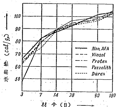
図-4 高熱セメント水和熱
