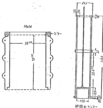
図-2 モールド並びに突き固メ用ランマー
