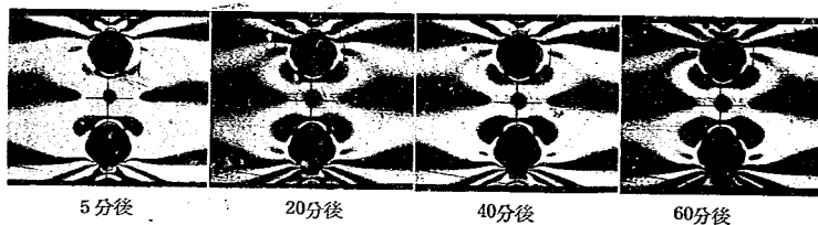
写真-3 2 円孔梁 純粹曲げ
