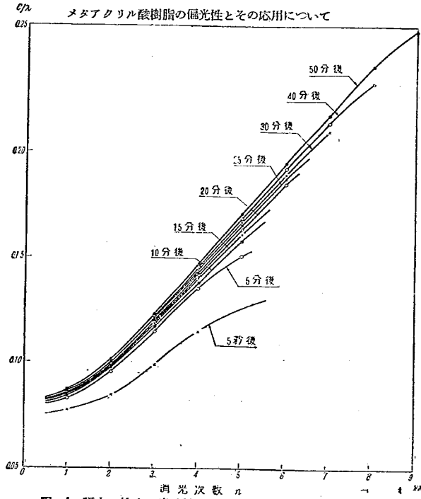
図-4 張力に於ける光弾性感度 c/l に対する消光次数 n および負荷時間の関係 (室温 28^{\circ}\text{C} )
