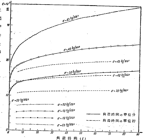
図-2 負荷時間の歪曲に対する影響 (室温 28°C)
