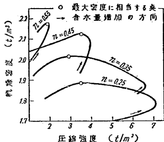
図-7 乾燥密度と圧縮強度との関係
