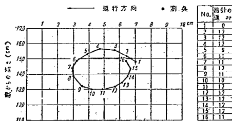
図-5 (a) 水分子軌道実験図 (例3)
