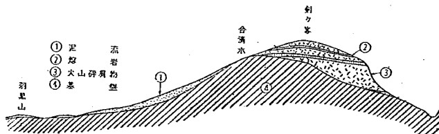
図-2 月山 proper 断面概念図
