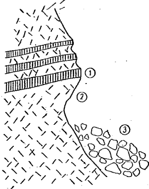
① 熔岩流 ② 火山碎屑物 (熔岩下部でえぐられている) ③ 崖壁 (熔岩破片及び 図-5 碎屑物中の岩片より成る)
