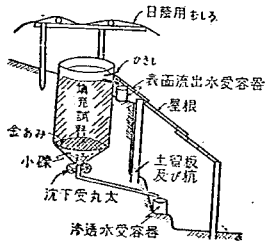
図-16 滲透計設置図
