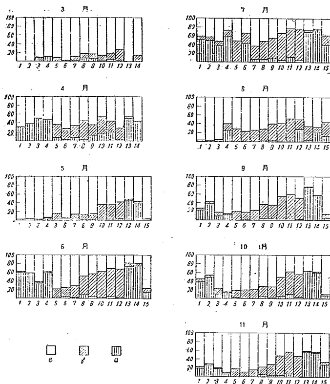
図一七 月別に見た降雨量、表面流出量(f) 滲透量(Q) 蒸発量(e) の関係
