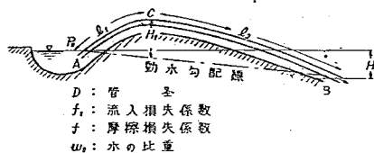
図-9 サイフォン
