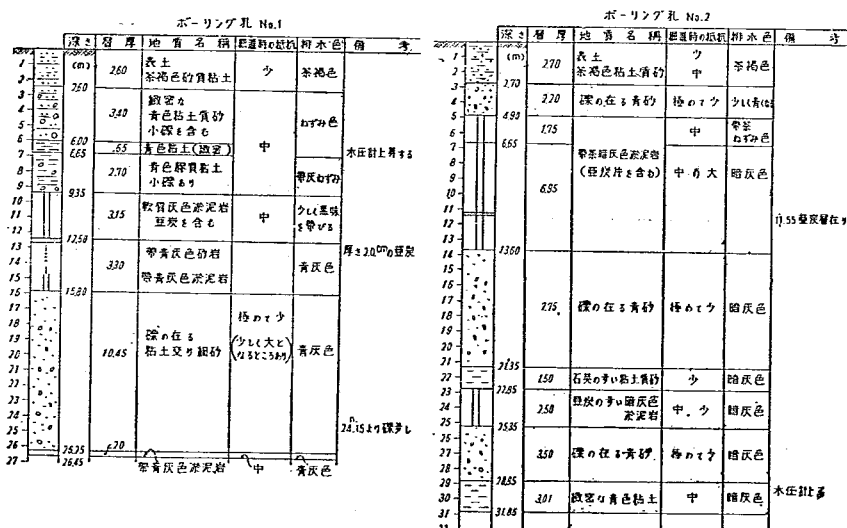
图一3 宇土沢排水隧道路地質図
