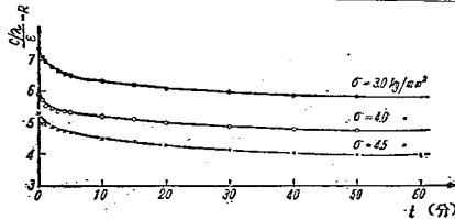
図-7 光弾性感度と歪に対する負荷時間の影響
