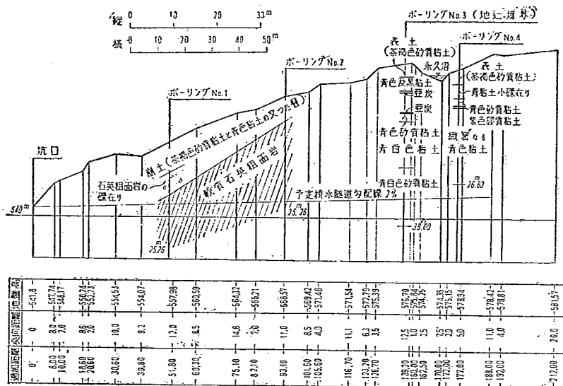
图一3 宇土沢排水隧道路地質図
