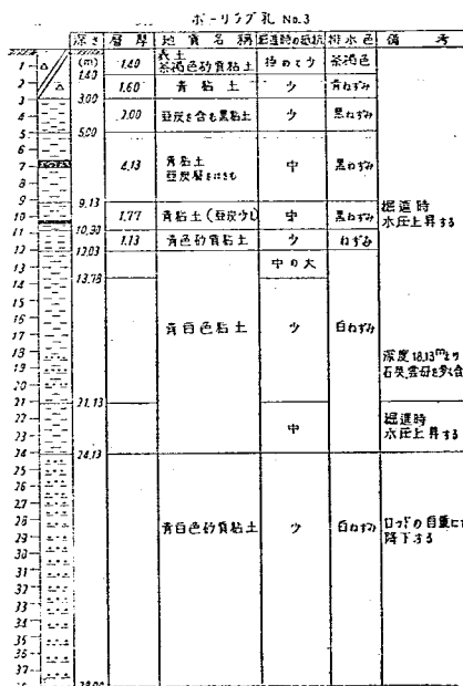
図-2 宇土沢側ボーリング柱状図
