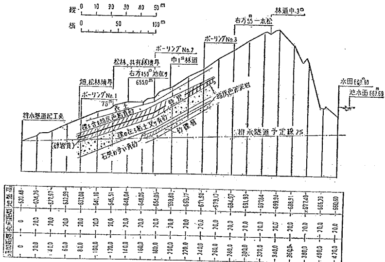
図-5 有旅側頂上排水隧道縦断地質図
