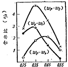
図-11 (w_0 - w_s) , (w_p - w_0) , (w_p - w_s) と n の間の関係
