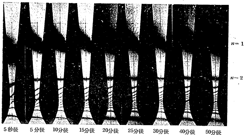
写真-1 引張時に於ける負荷時間の縮戻様に対する影響
