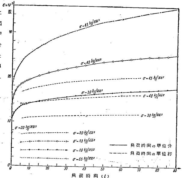
図-2 負荷時間の creep に対する影響 (室温 28°C)
