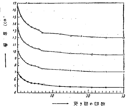
図-5 突キ固メ回数と層厚との関係
