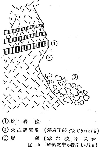
図-5 碎屑物中の岩片より成る
