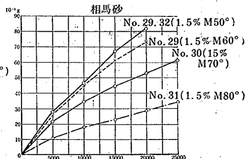
(d) 含水率速度を一定にして削り角をかえた場合
