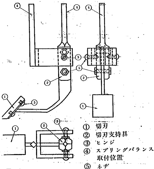
図—4 モーメント測定装置
