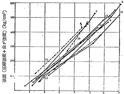
図—16 強度水と熱比と強度の関係
