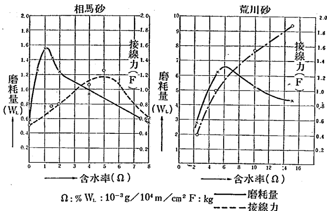
図—17 含水率と磨耗量及び接線力との関係
