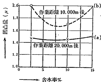
図—19 一定作業距離に於ける表面凹凸量と含水量との関係
