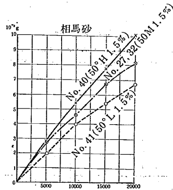
(b) 含水率削り角を一定にして速度をかえた場合
