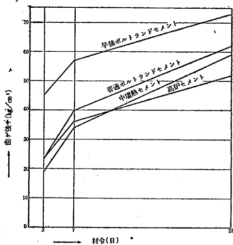
図-3 曲グ強サ
