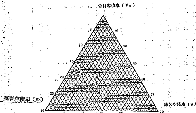
図-7 V_a-v-v 三元系
