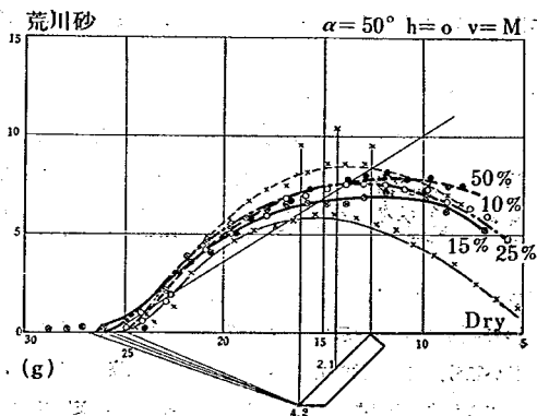
図一〇 切刃面上に於ける砂の流動
