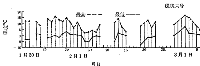
図一1 コンクリート養生室内の温度図
