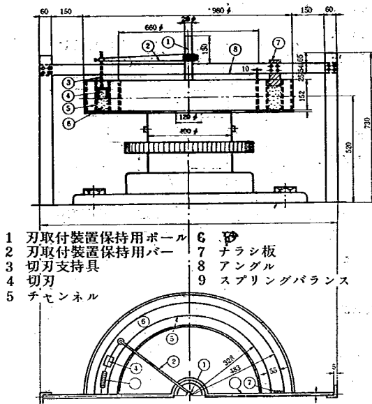
図一 磨耗試験機全図
