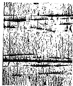
相馬砂 \Omega=1.5\% V=M 磨耗距離 10000m 後ノ 磨耗面 (×100)
