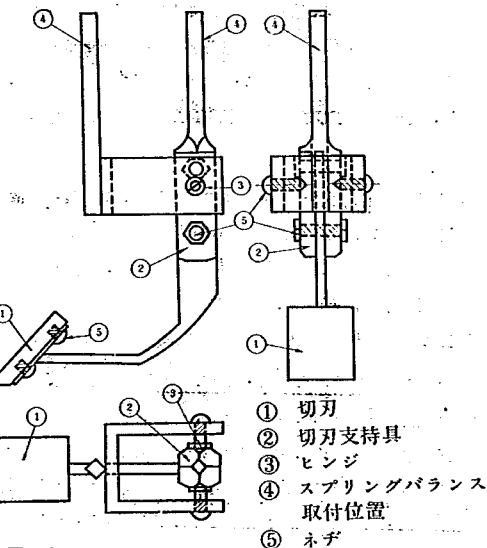
図一4 モーメント測定装置
