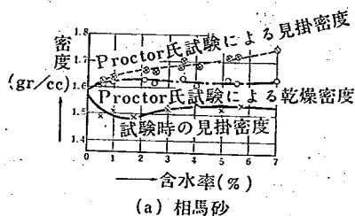
図-13 含水率と密度との関係
