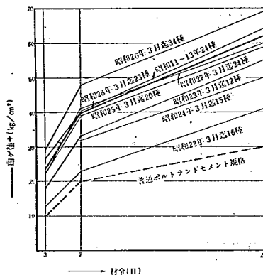
図-2 普通ポルトランドセメント曲げ強サ
