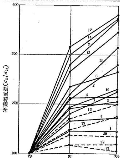
図-18 コンクリート圧縮強度増進率
