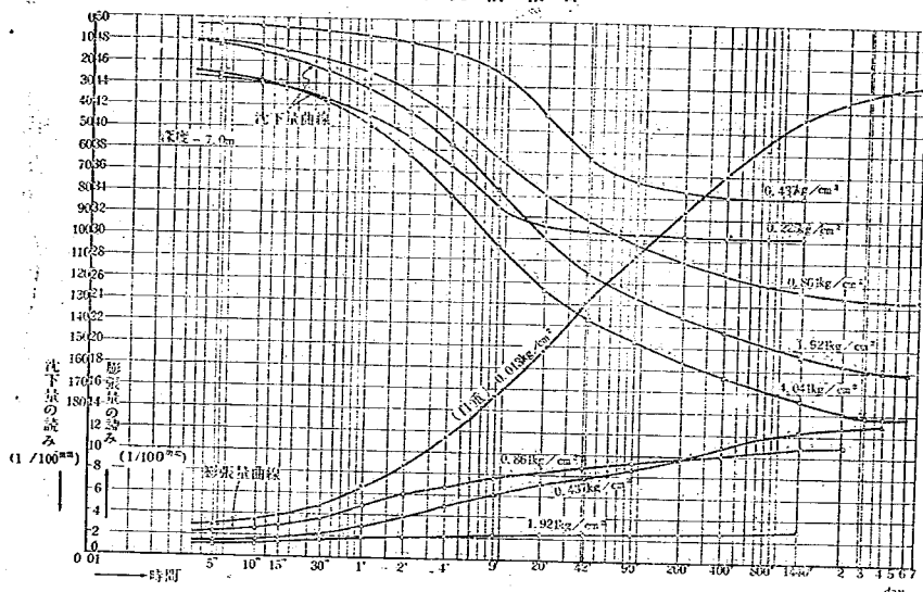
図-17 深度-7.0m
