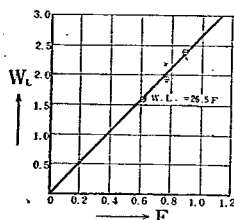
図—21 磨耗量と接線力との関係
