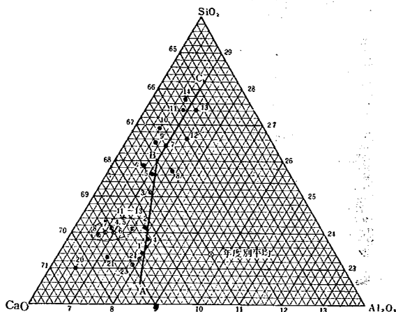
図-3 低発熱型セメントの \text{CaC}-\text{SiO}_2-\text{Al}_2\text{O}_3 三元組成
