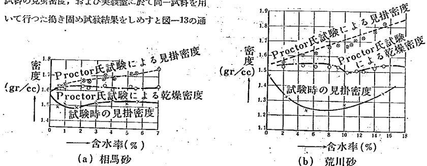
図-13 含水率と密度との関係
