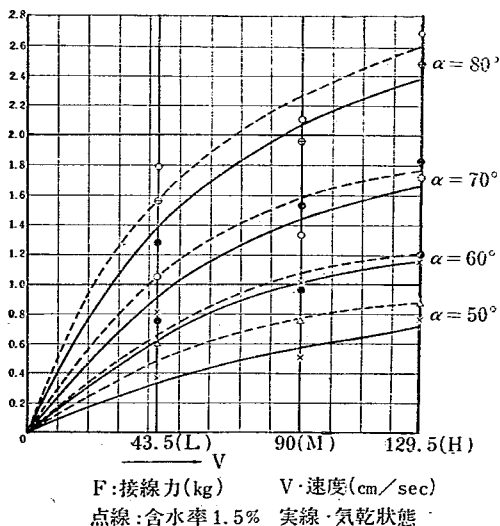
図—22 接線力と速度との関係
