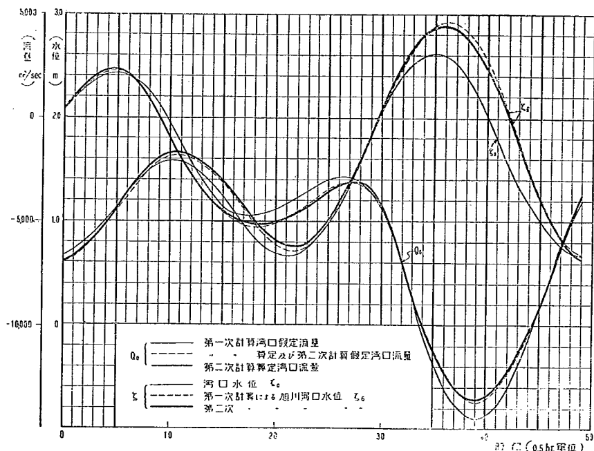
図-12 洪水時締切前の湾口の仮定及び算定流量並びに旭川河口水位
