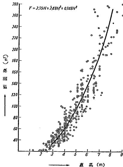
図-6 直高と断面積との関係
