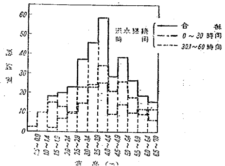
図—18 直高と洪水継続時間との関係
