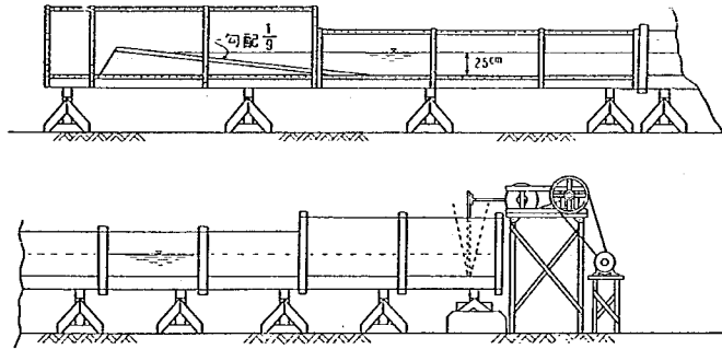
図-2 実験水路
