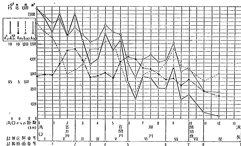
図-7 児島湾有効断面積、有効幅、径深変化
