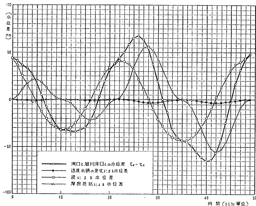
図-14 平水時の締切前の湾口と旭川河口の潮位の水位差の分析
