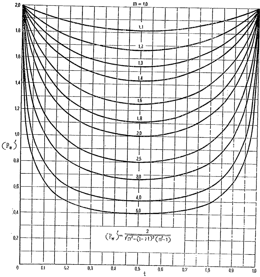
附図-5 (P_*)' \sim t, m 曲線
