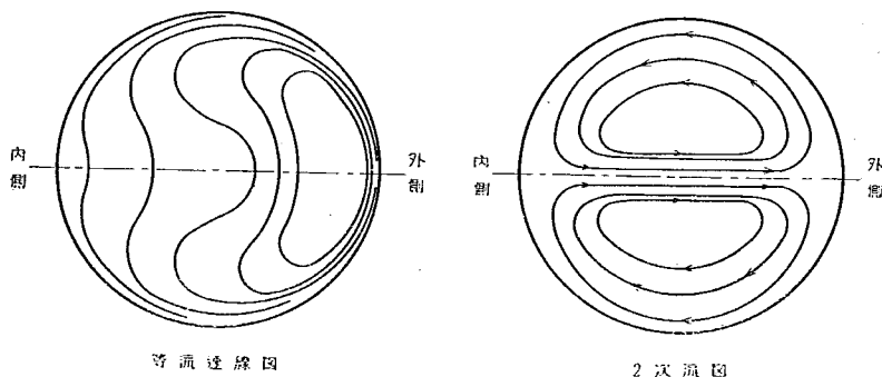
図-15 曲管内の流れ
