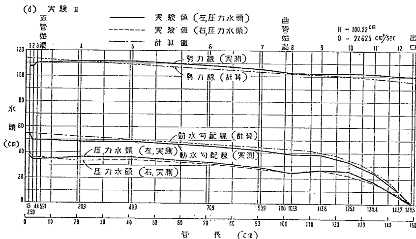
図-11-(d) 勢力線, 動水勾配線, 上下圧力水頭線図
