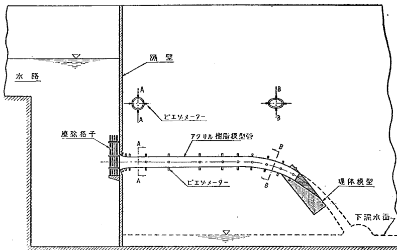
図-5 模型実験装置図
