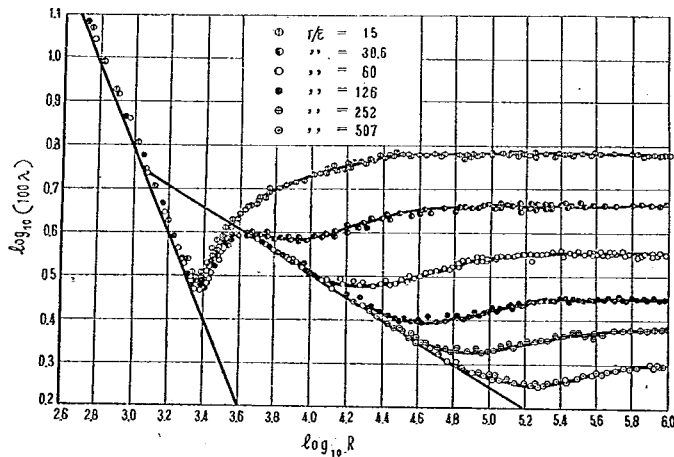
図-13 Reynolds 数と \lambda との関係
