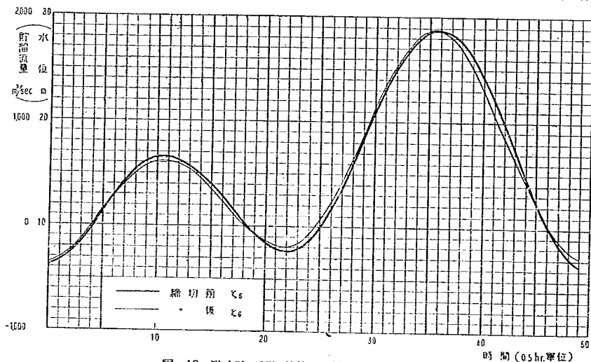
図一16 洪水時の締切前後の旭川河口水位比較
