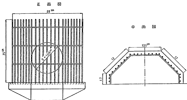
図-10 塵除格子構造図
