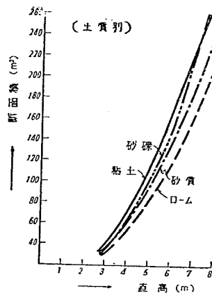
図-16 直高と断面積との関係
