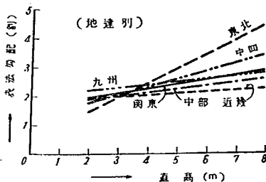
図-7 直高と表法勾配との関係
