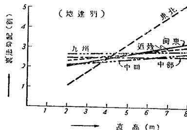
図-8 直高と裏法勾配との関係
