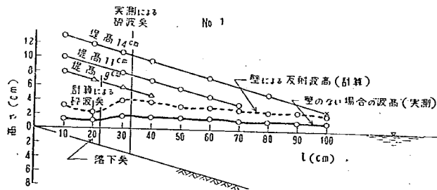
図-4 (a) 堤防の種々なる位置における衝突波の状態
