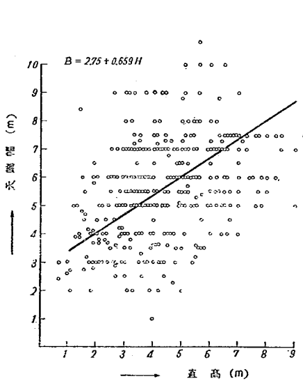
図-4 直高と天端幅との関係
