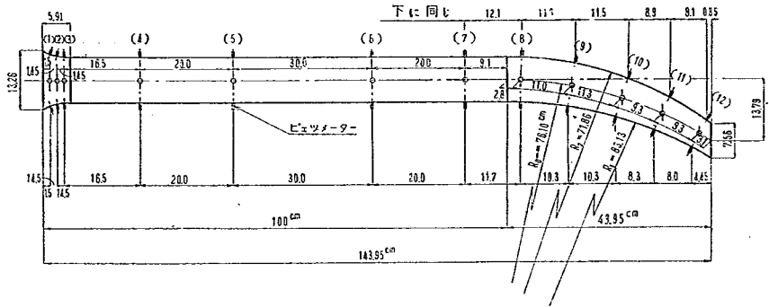
図-6 管水路全体図
