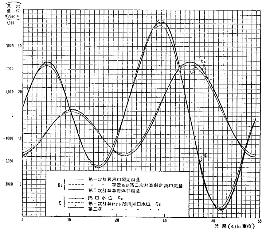
図-9 平時締切前の湾口の仮定及び算定流量並びに旭川河口水位
