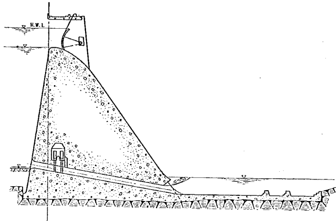
図-4 III型放水管を有する堰堤
