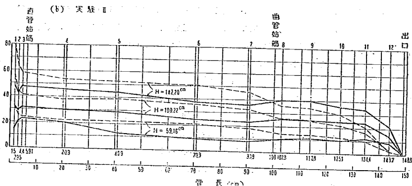
図-16 (b) 上下ピエゾメーターの圧力水頭線
