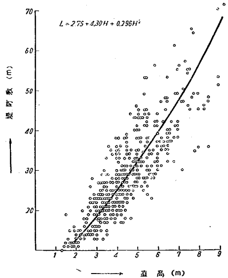
図-5 直高と堤防敷との関係
