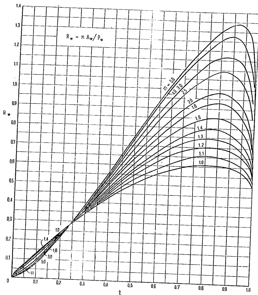
附圖-4 R_* \sim t, m 曲線
