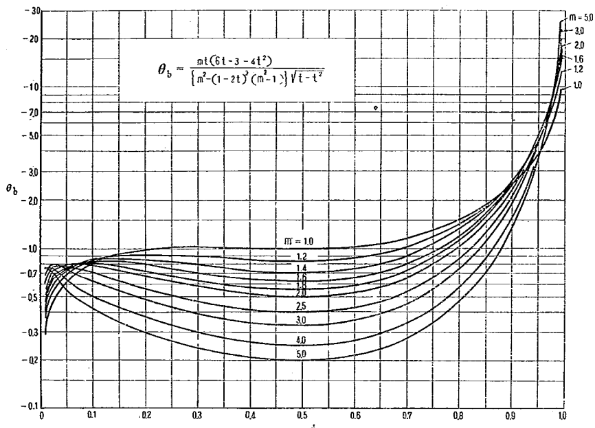
附圖—8 \theta_b \sim t, m 曲線
