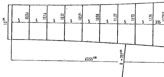
図-8 曲管部平面図
