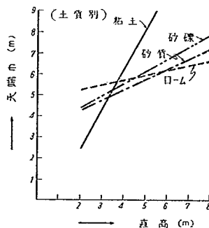
図-14 直高と天端幅との関係
