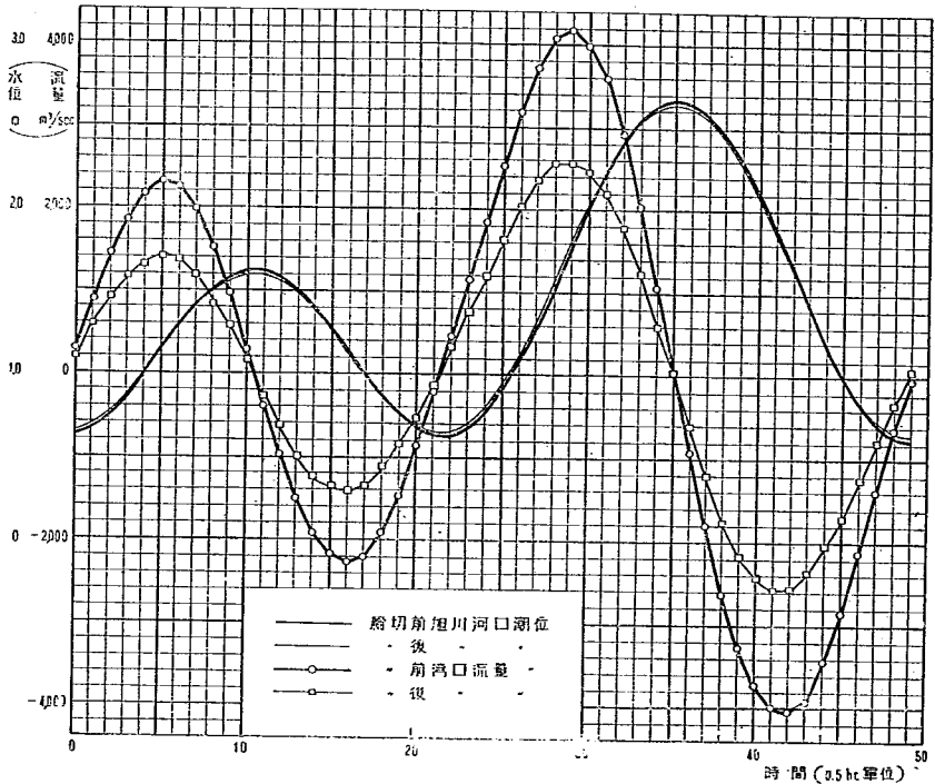
図一11 平時締切前後の湾口流量及び旭川河口潮位の比較
