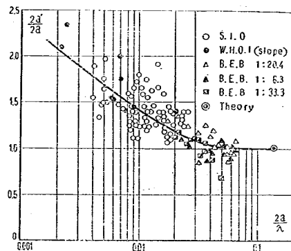
図-13 沖波の尖鋭度の函数としての碎波点の波高と沖波高との比
