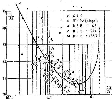
図-14 沖波の尖鋭度の函数としての碎波水深と沖波高との比
