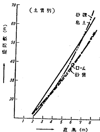
図-15 直高と堤防敷との関係
