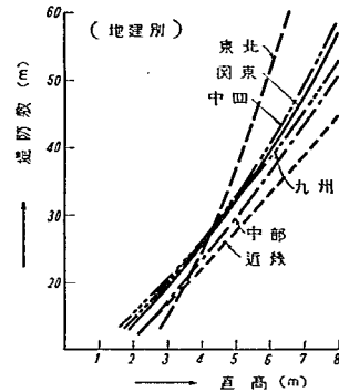
図-10 直高と堤防敷との関係
