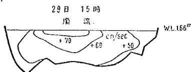
図-3 児島湾口流況
