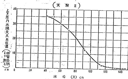
図-17 上下圧力水頭交叉点と水位との関係
