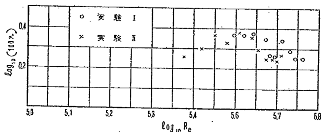
図-14 Reynolds 数と \lambda との関係 (実験値)
