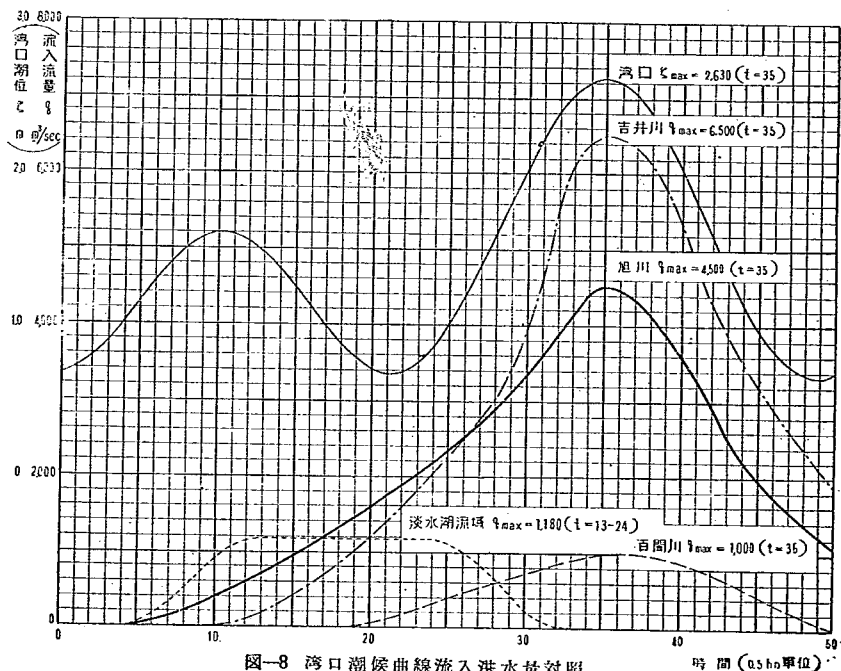
図-8 湾口潮候曲線流入洪水量対照
