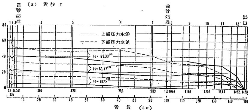
図-16 (a) 上下ピエゾメーターの圧力水頭線
