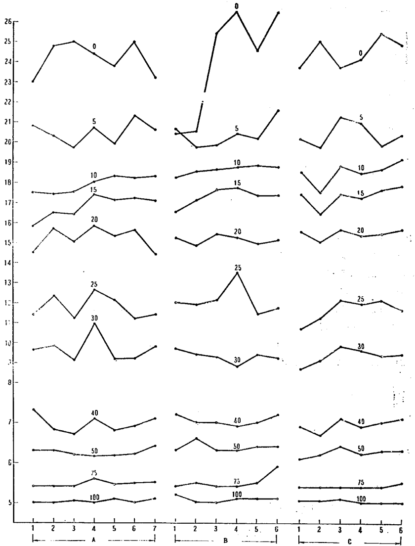
図-8 田沢湖の深度と水温
