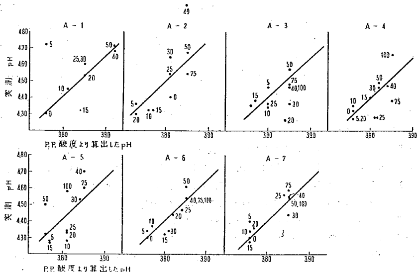
図-10 P.P. 酸度より算出した pH と実測 pH の関係
