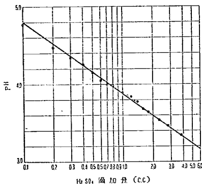
図-15 田沢湖水の滴定線
