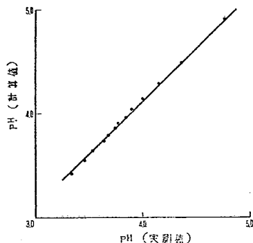
図-16 pHの実測値と計算値(硫酸滴加時)
