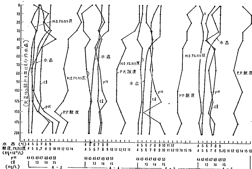
図-13 A断面の pH、水温、酸度、アルカリ度及び塩素含量 (昭29.12.12)
