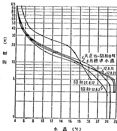
図-7(B) 田沢湖水温の比較(8月)
