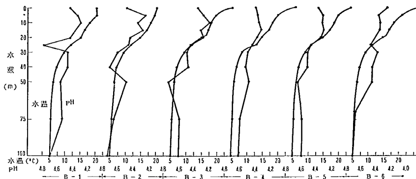
図-4 B断面の pH と水温
