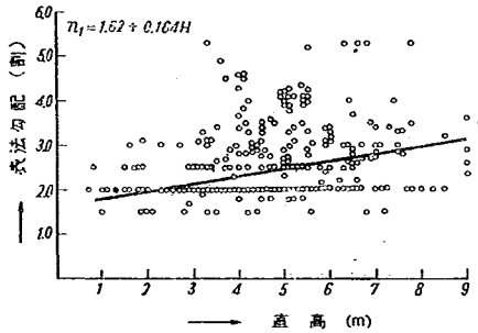
図-2 直高と表法勾配との関係
