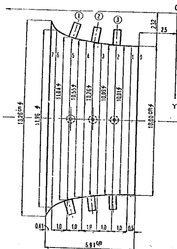
図-9 ベルマウス曲線形
