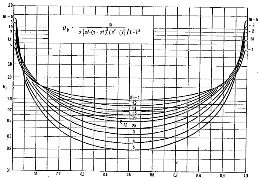
附圖—6 \theta_h \sim t, m 曲線
