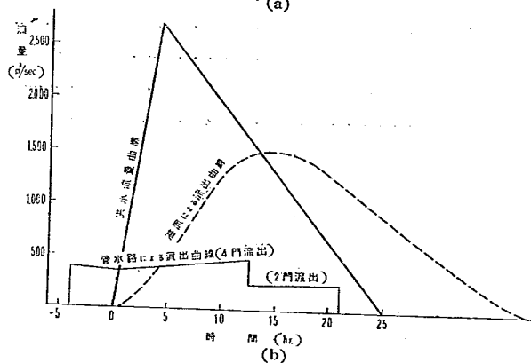
図-1 洪水調節操作方法の例
