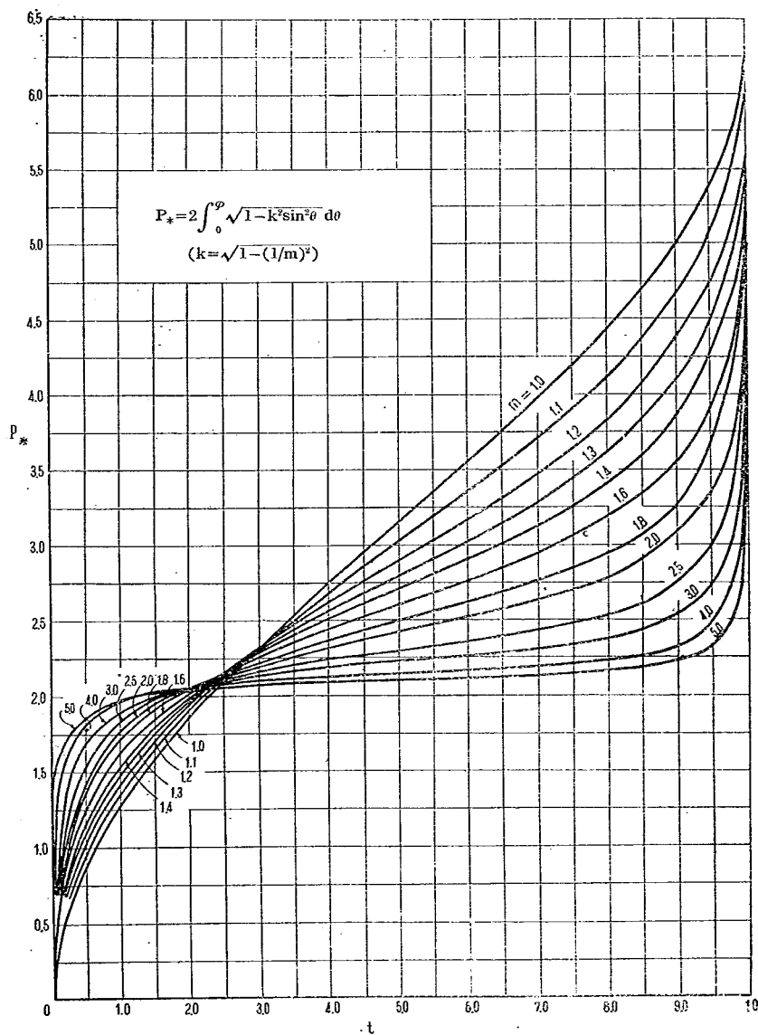
附図-3 P_* \sim t, m 曲線
