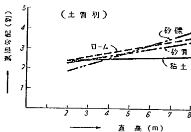
図-13 直高と堤防勾配との関係
