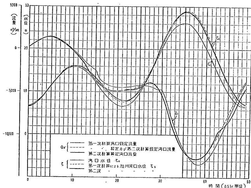
図—13 洪水時締切後の湾口の仮定及び算定流量並でびに旭川河口水位
