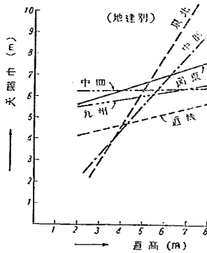
図-9 直高と天端幅との関係
