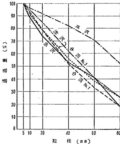
図-3 本沢、赤沢、濁沢及び合流後の粒度曲線
