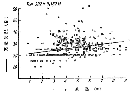
図-3 直高と裏法勾配との関係
