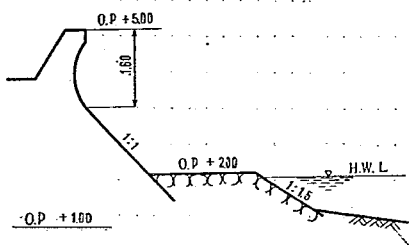
図-1 (a) 泉南郡樽井地先 護岸標準断面 (単位:m)
