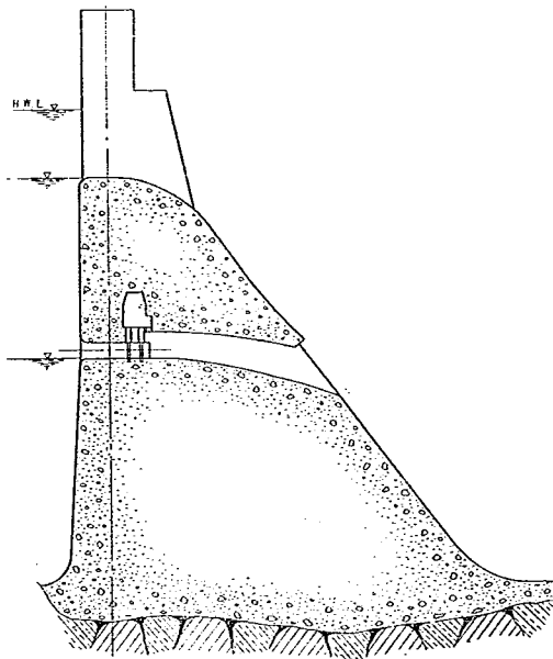
図-3 II型放水管を有する堰堤
