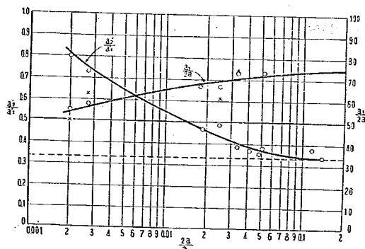
図-11 沖波失鋭度と波高上昇比 ( a_1/2a ) との関係. 2a/\lambda は沖波の失鋭度, a_1' は砕波点における静水面上の波高, a_2' は同じく静水面下の波高, a_1/2a は砕波点より岸側における全波高 2a = a_1 + a_2 に対する静水面上波高 a_1 の比.
