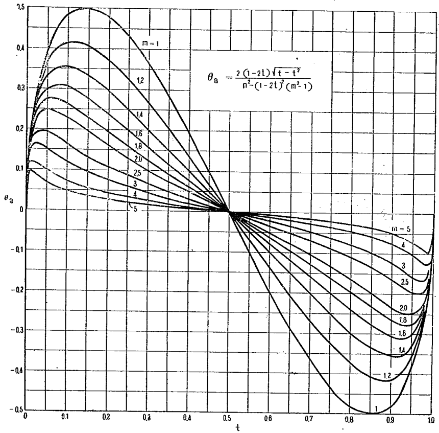
附図—7 \theta_a \sim t, m 曲線
