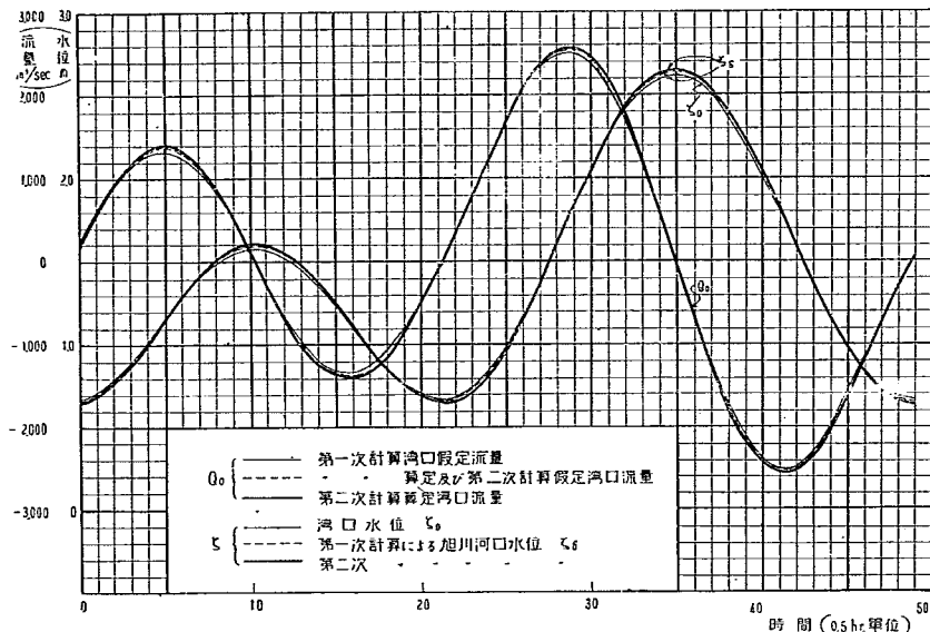
図-10 平水時締切後の湾口の仮定及び算定流量並びに旭川河口水位
