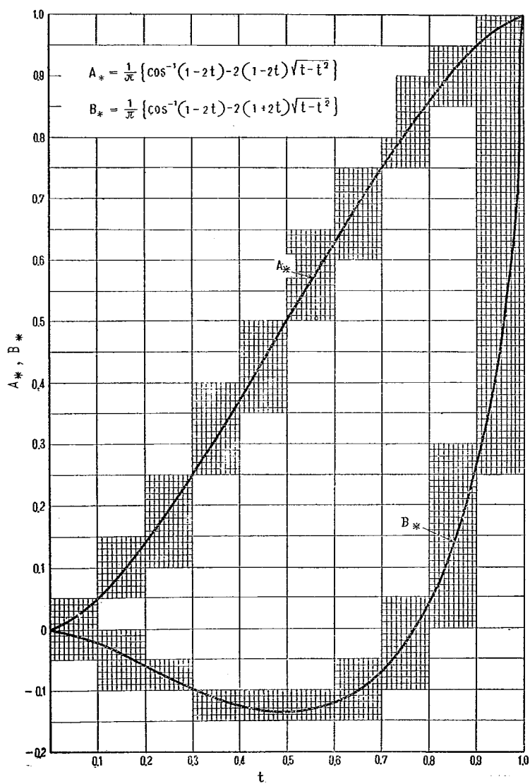
附圖-1 A_*, B_* \sim t 曲線
