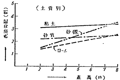
図-12 直高と表法勾配との関係
