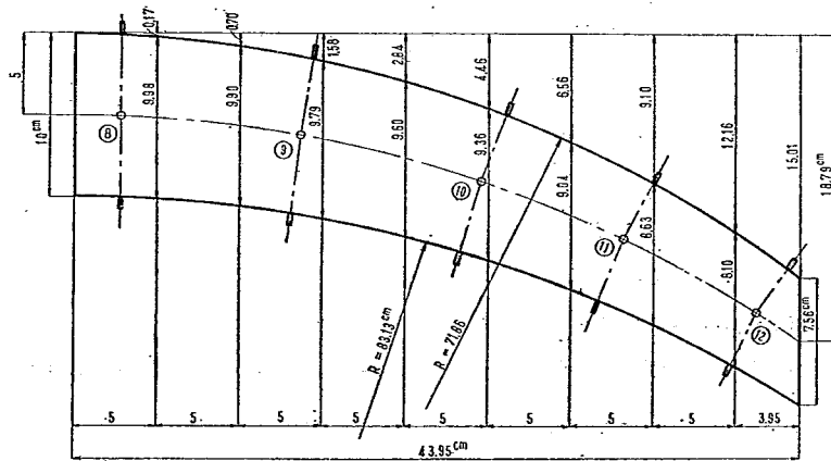
図-7 曲管部側面図
