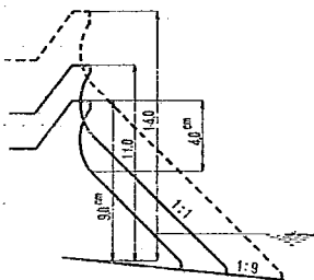
図-1 (b) 模型断面
