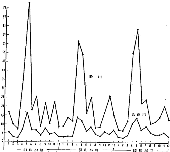
図-12 玉川、先達川平均流量 (m³/sec) (昭和24~26年)
