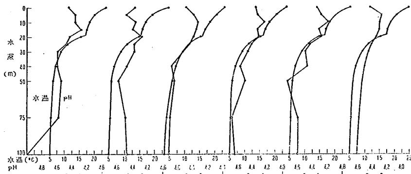
図-5 C断面の pH と水温
