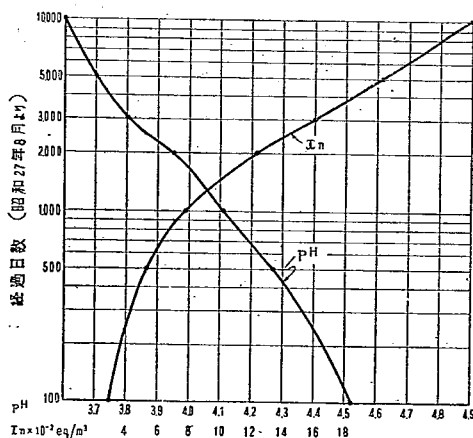
図-11 田沢湖の将来の酸性化程度
