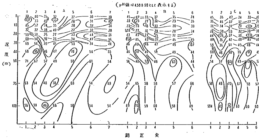
図-2 A. B. C 線垂直断面の等 pH 線 (昭和 27. 8. 12—15)
