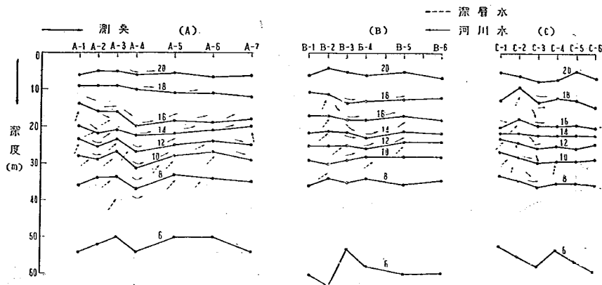
図-9 田沢湖の等温線
