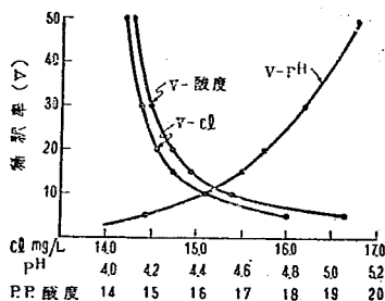
図-6 稀釈率(V)とpH, Cl 含量, P.P. 酸度
