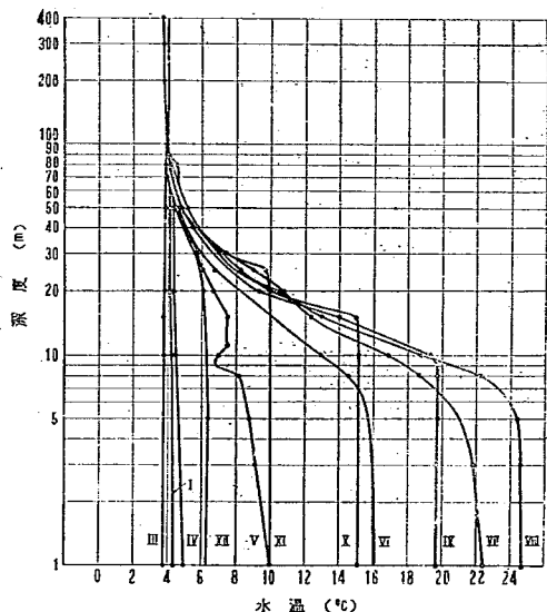
図-7 (A) 田沢湖標準水温(毎月26日)大正15年~昭和8年
