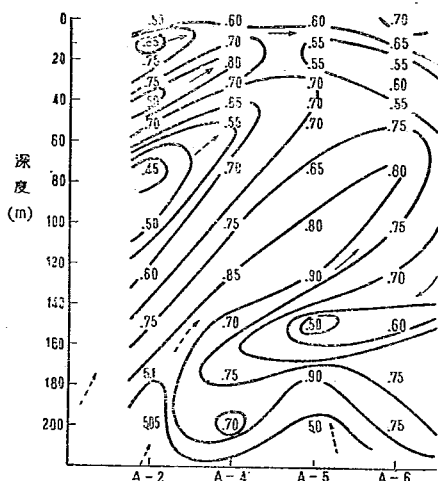
図-14 A断面の等pH線
