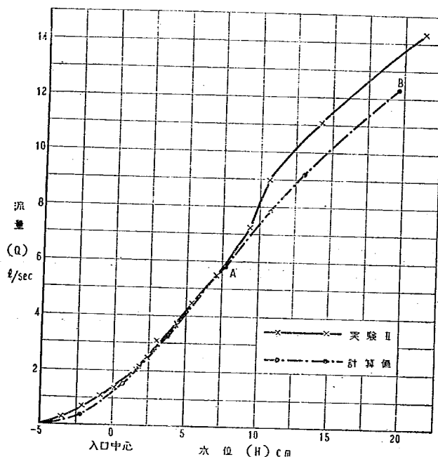
図-25 水位・流量曲線 (2)
