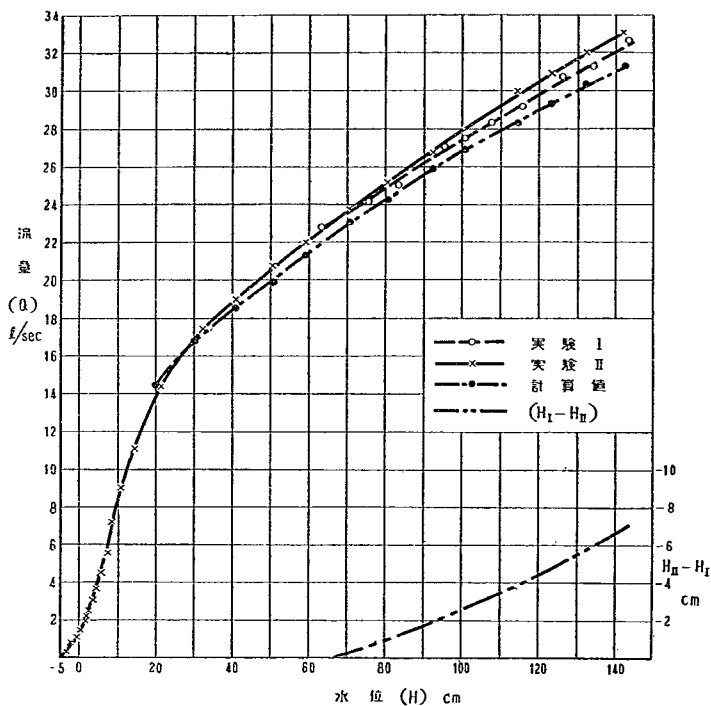
図-12 水位・流量曲線(1)
