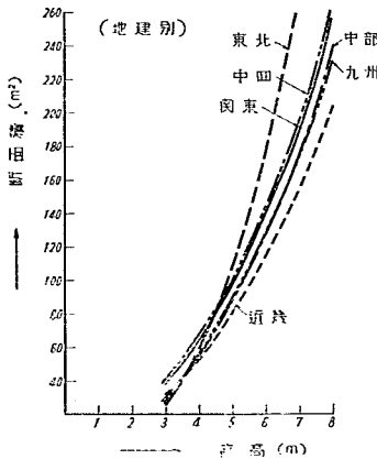
図-11 直高と断面積との関係
