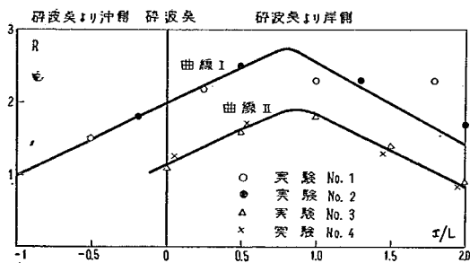
図-7 R と \frac{x}{L} の関係
