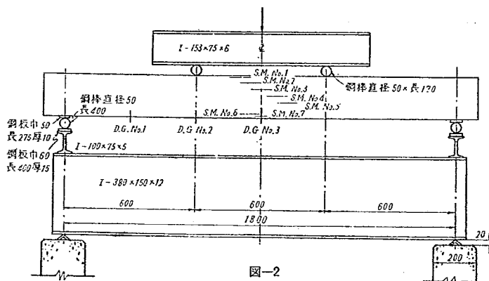
鉄筋コンクリートはりの載荷試験装置正面図
