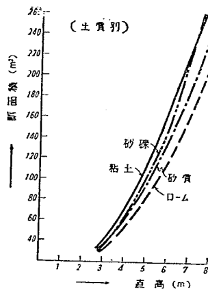
図-16 直高と断面積との関係
