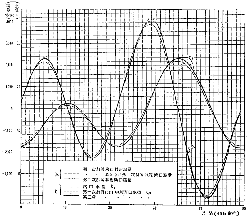
図-9 平時締切前の湾口の假定及び算定流量並びに旭川河口水位
