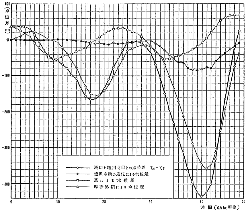
図一15 洪水時の締切前の湾口と旭川河口との水位差の分析
