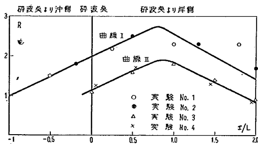
図-7 R と \frac{x}{L} の関係
