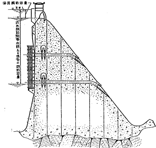
図一2 I型放水管を有する堰堤
