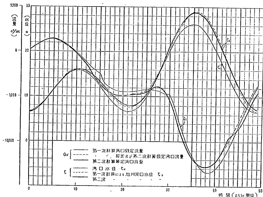
図—13 洪水時締切後の湾口の仮定及び算定流量並びに旭川河口水位
