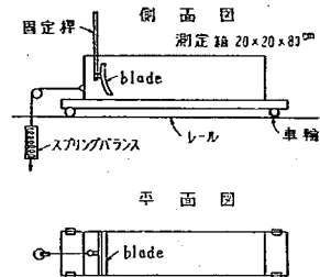
図-60 実験装置の概要 (学生実験)
