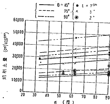
図-20 切削土量と \alpha の関係 (切削幅一定 (43.6cm) として計算 ( d=1.43\sim 1.46\text{gr/cm}^3 , w=2.69\sim 4.94\% ))
