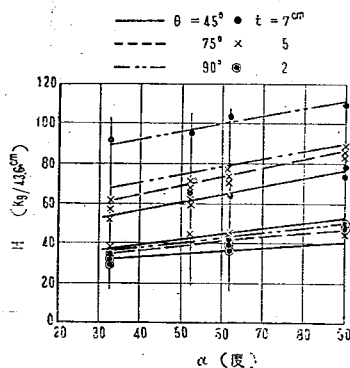
図-18 H と \alpha の関係 (切削幅一定 (43.6cm) として計算 ( d=1.43\sim 1.46\text{gr/cm}^3 , w=2.69\sim 4.94\% ))
