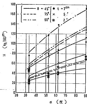
図-17 H と \alpha の関係 (edge の長さ一定 (66.3cm) として計算 ( d=1.43\sim 1.46\text{gr/cm}^3 , w=2.69\sim 4.94\% ))
