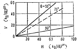
図-43 H と V の関係 (試料: 真砂土, edge: 曲刃) t=5 cm, v=1 速
