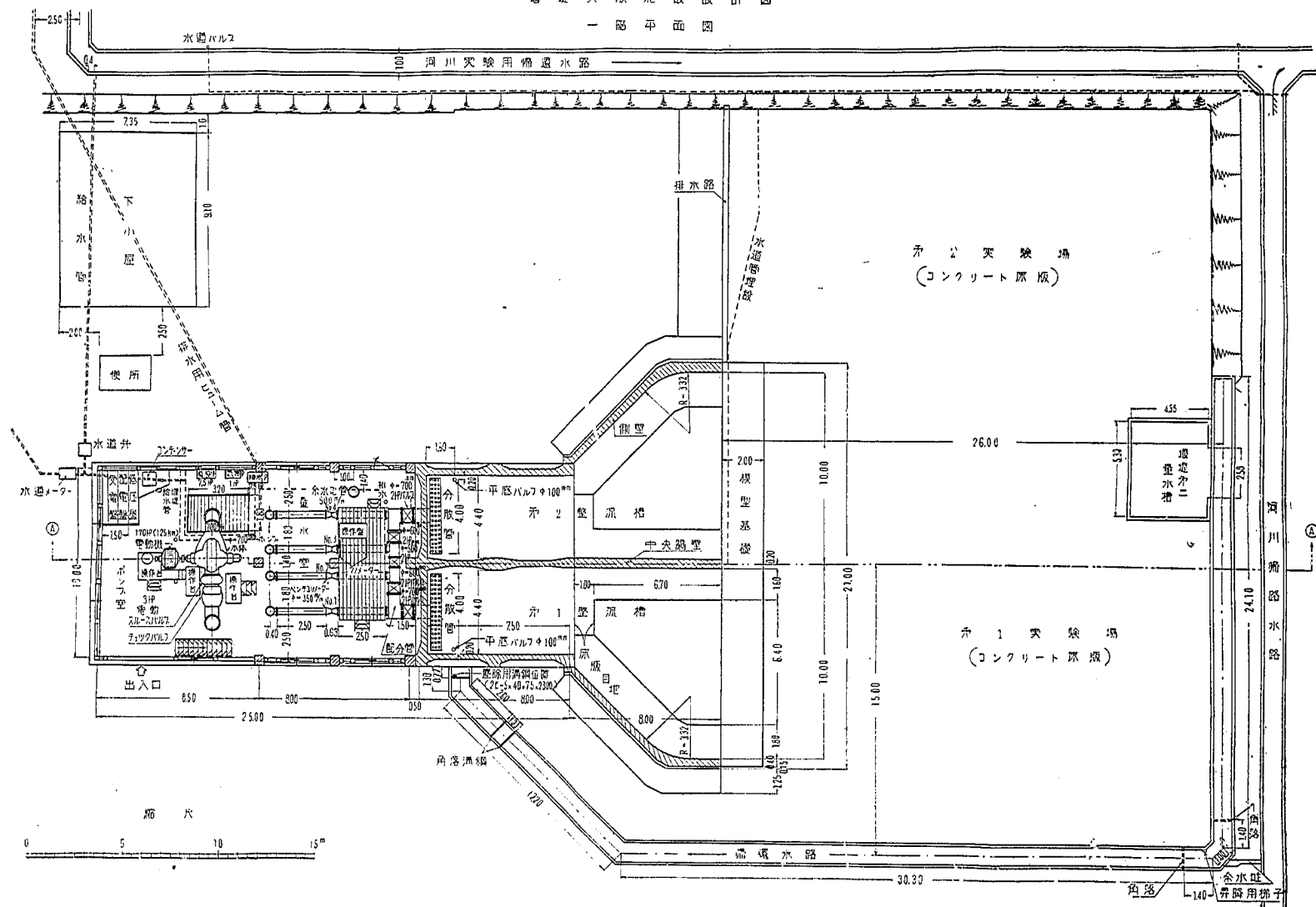
附図-2 堰堤実験施設全般平面図
