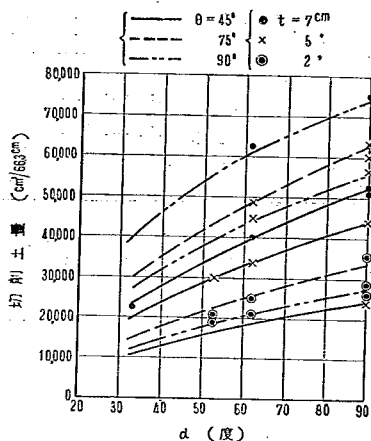
図-19 切削土量と \alpha の関係 (edge の長さ一定 (66.3cm) として計算 ( d=1.43\sim 1.46\text{gr/cm}^3 , w=2.69\sim 4.94\% ))
