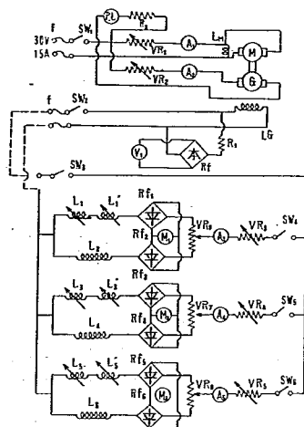
図一5 高周波発生による装置
