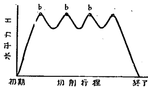
図-9 水平力 H と切削行程
