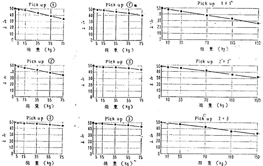
図—16 各ピックアップの検定曲線
