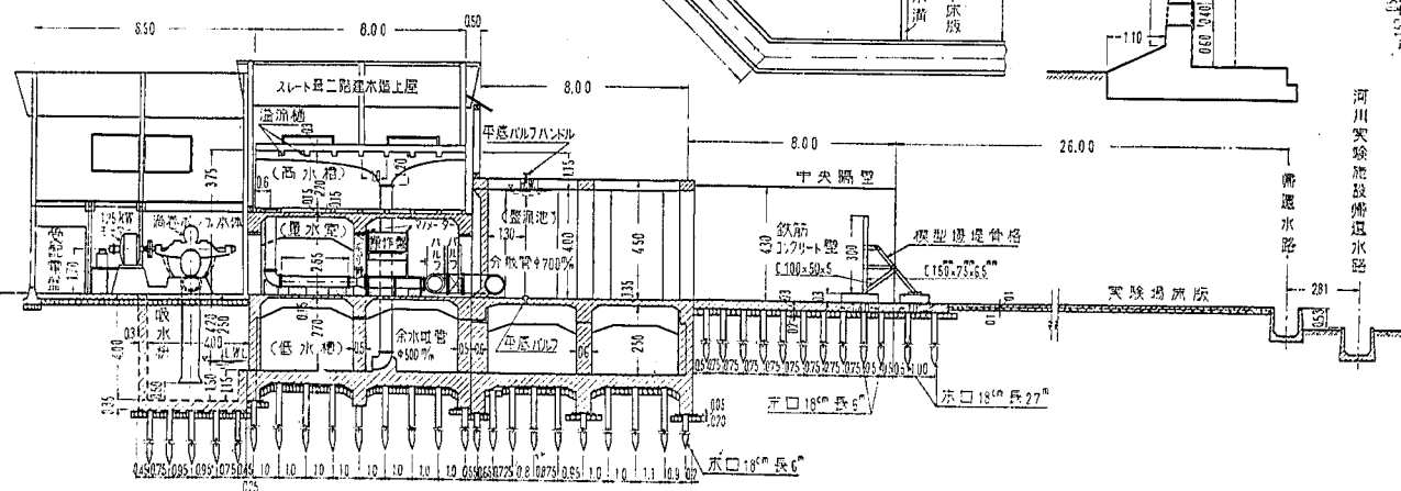
附圖一3 堰堤突驗施設各部構造圖
