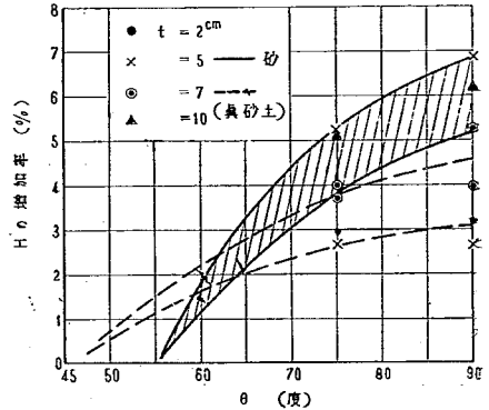
図-55 \theta の変化による H の増加率 (edge: 直刃 (長さ 50cm) \alpha = 90^\circ , v = 1 速, loose な場合)
