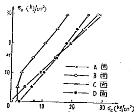
図-9-5 硝子の歪より測定した各面中央部の応力
