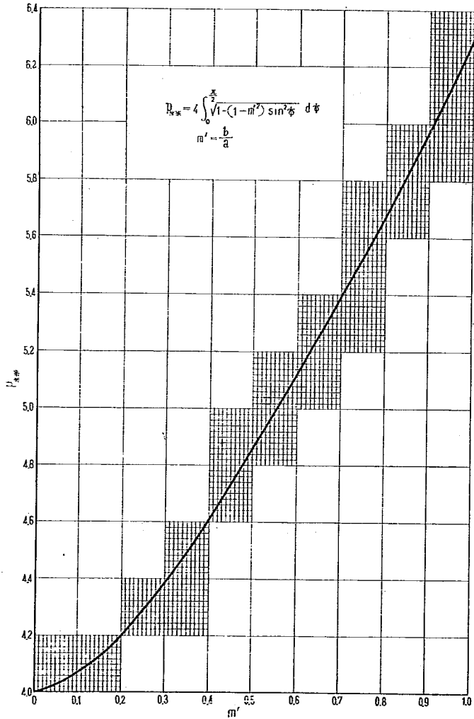
附圖—1 P_{**} \sim m' 曲線
