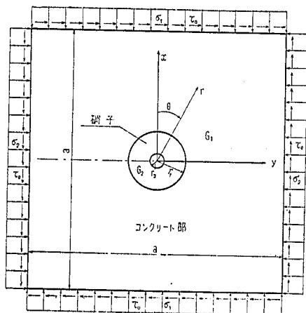
附図—1 供試体に対する外力の作用と、座標の取方 ただし { コンクリートの young 率 = 210,000 kg/cm 2 硝子の " = 750,000 " コンクリートの poisson's numb = 6 " 硝子の " = 4 }
