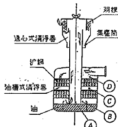
図-9 建設機械用エヤークリーナの構造
