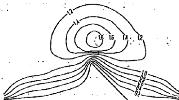
図-12 不透過斜 (45°) 水制合成速度分布図
