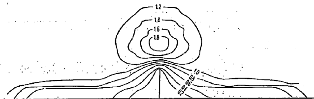
図-10 不透過直角水制合成速度分布図
