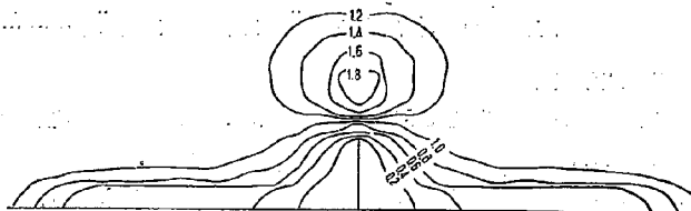
図-11 不透過直角水制 u 分布図
