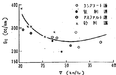
図-2. c 速度と燃料消費率
