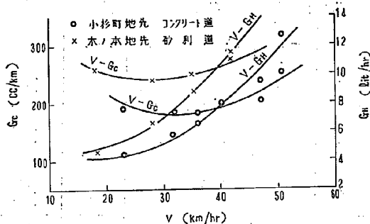
図-3 速度と燃料消費率
