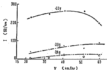
図-7・b V-I 曲線
