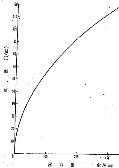
図-3 差圧～流量関係図
