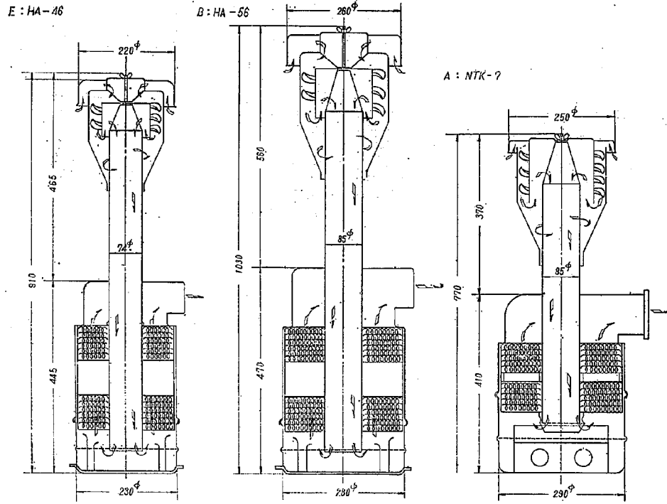
図-5 建設機械用エアークリーナ
