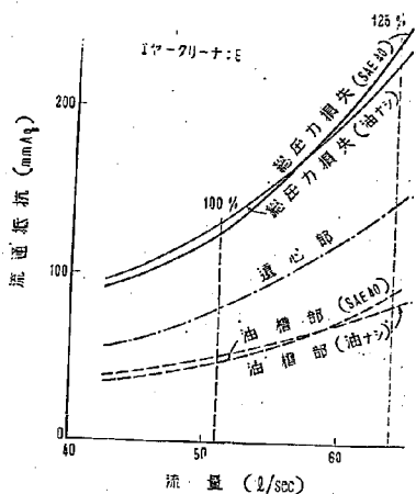
図-21 流通抵抗試験成績図 (E)
