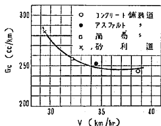
図-9 路面種別ごとの平均速度・燃料消費率の位置
