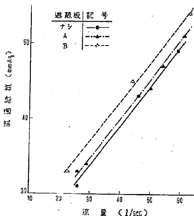
図-28 流通抵抗比較図
