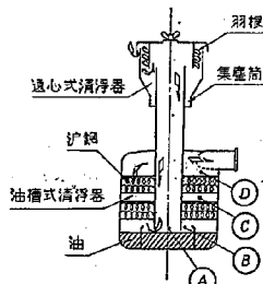
図-9 建設機械用エヤークリーナの構造
