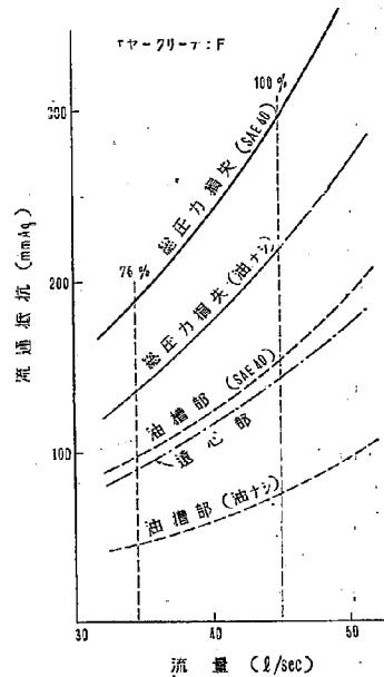
図-18 流通抵抗試験成績図 (B)
