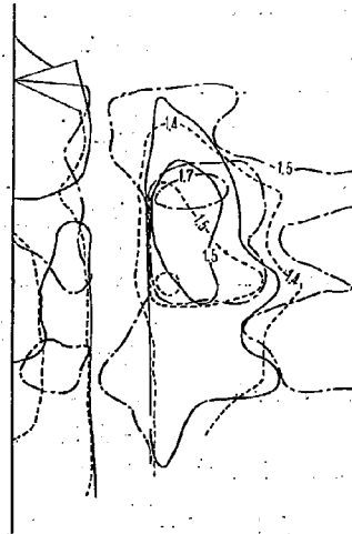
図-9 流速分布図 (流量 30 l/sec)
