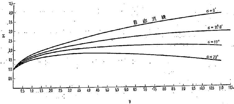
図-2 自由流線と噴出線
