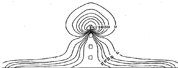
図—15 透過直角水制 \psi 分布図
