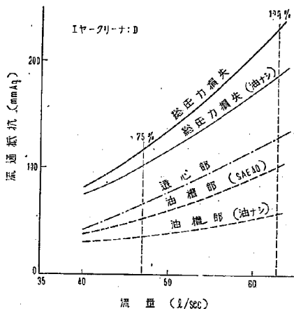
図-20 流通抵抗試験成績図 (D)
