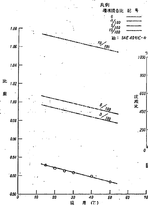
図一15 塵埃混入による比重変化 (SAE 40)
