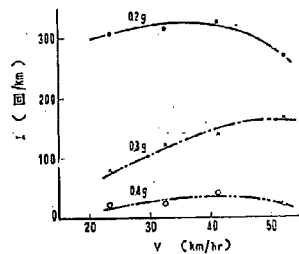
図-7・d V-I 曲線
