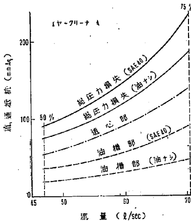
図-17 流通抵抗試験成績図 (A)
