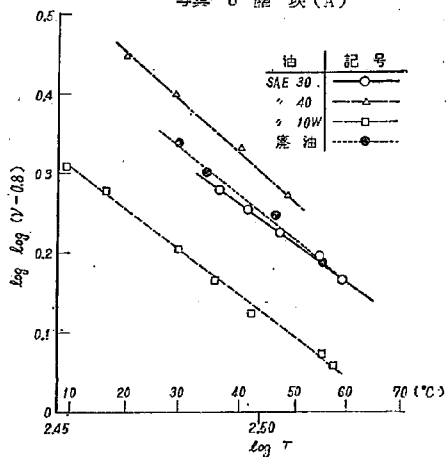
図-8 油の粘度特性
