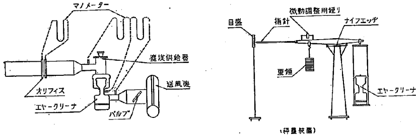
図-1 試験装置
