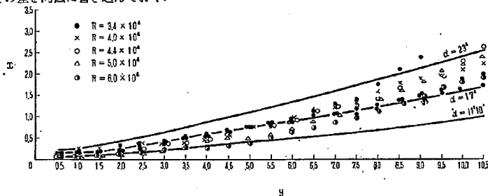
図-5 噴出角と Reynolds 数の関係
