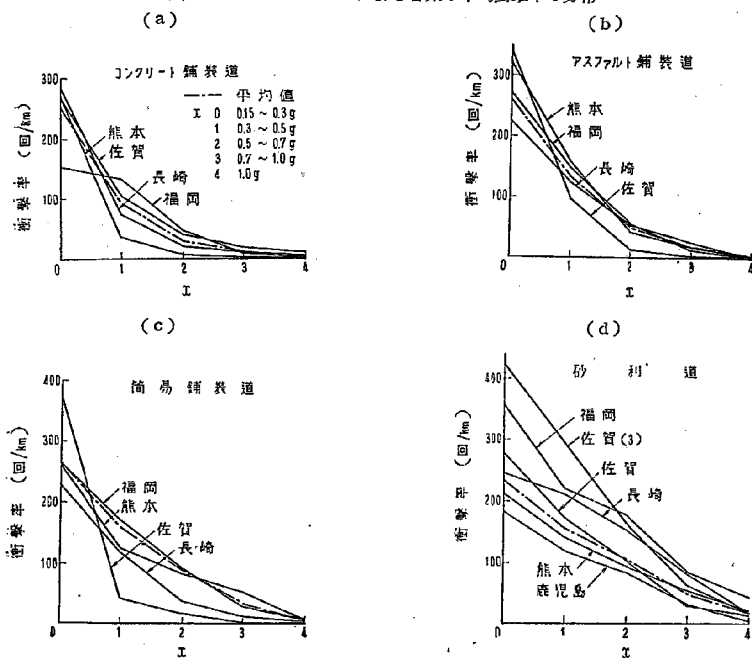
図-11 振動強度分類計による各県の平均損傷率の分布
