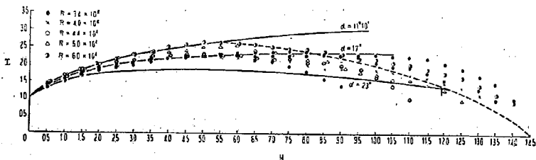
図-6 水制域と Reynolds 数の関係図
