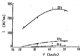
図-7・a V-I 曲線
