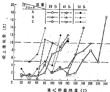
図-24 遠心部容量試験成績図
