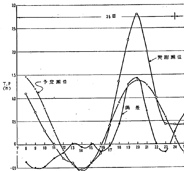
図-11 前芝潮位と偏差
