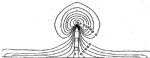
図—14 透過直角水制合速度分布図
