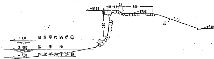
図-27 鈴鹿市南若松町字山中地内若松海岸横断面
