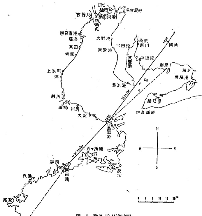
図-1 颱風13号進路図
