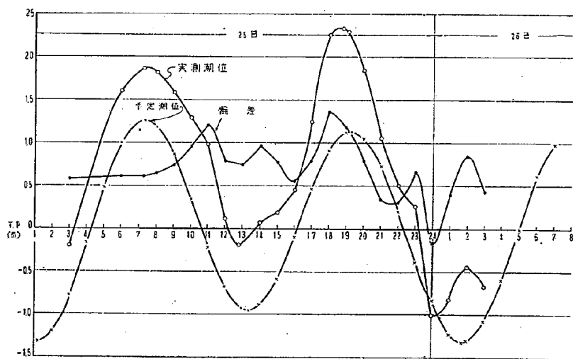
図—9 名古屋潮位と偏差
