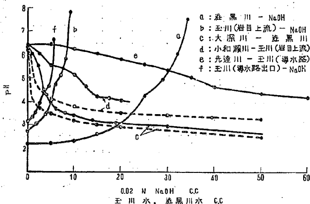
図一8 玉川および玉川と支流との滴定曲線 (100 c.c.)
