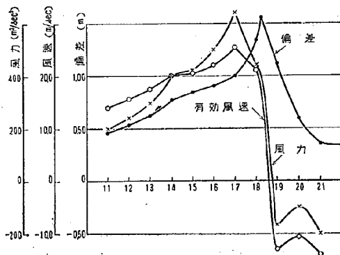
図-13 鳥羽の偏差と風速、風力との相関
