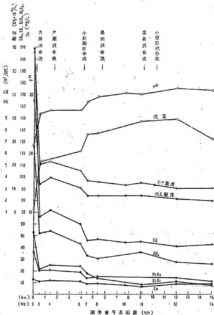
図-2 玉川の流下中における水質の変化 (昭和28.10.3~7)
