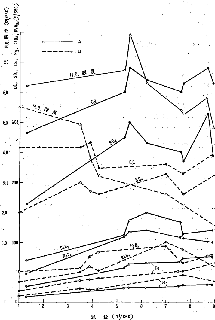
図-6 溶存成分の流出量と流量
