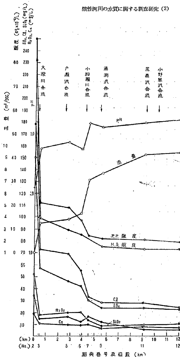
図-3 玉川流下中における水質の変化 (昭和26.10.3~6)
