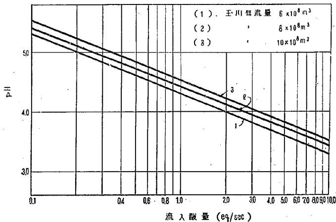
図-10 貯水池の pH と流入酸量
