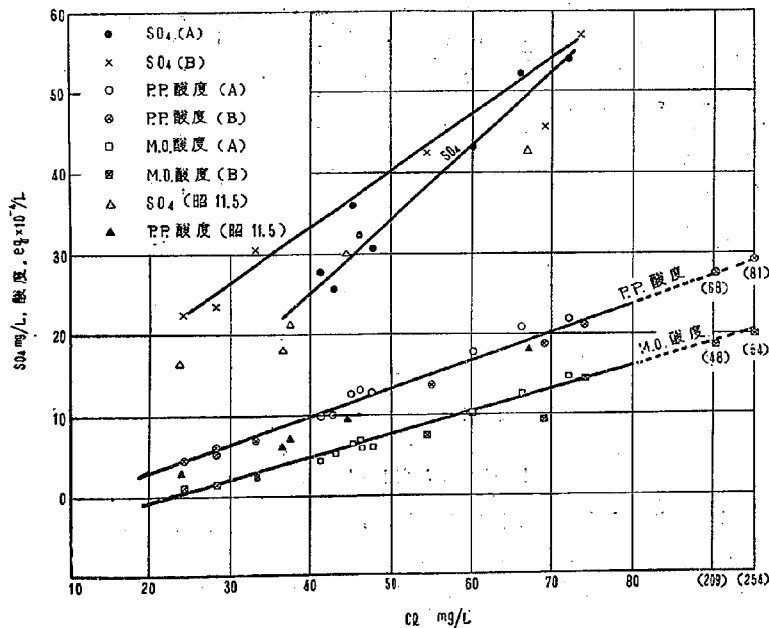
図-4 \text{Cl} と \text{SO}_4 、酸度の関係
