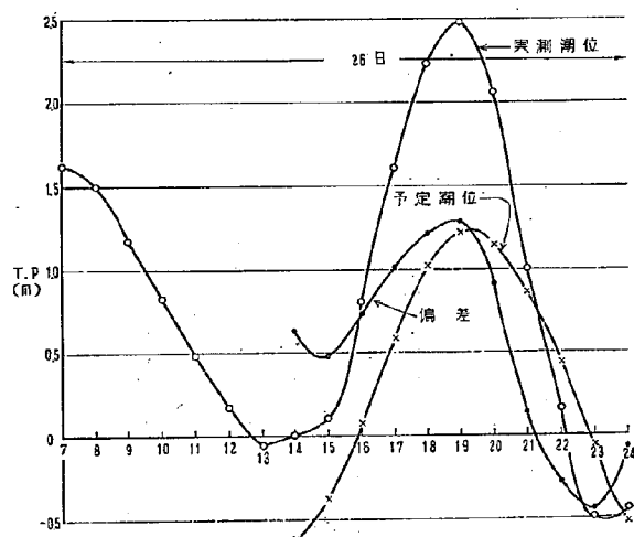
図-10 武豊潮位と偏差
