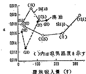
図-26 油槽部塵埃吸入量と \alpha との関係
