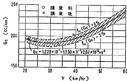
図-5 燃料消費率曲線
