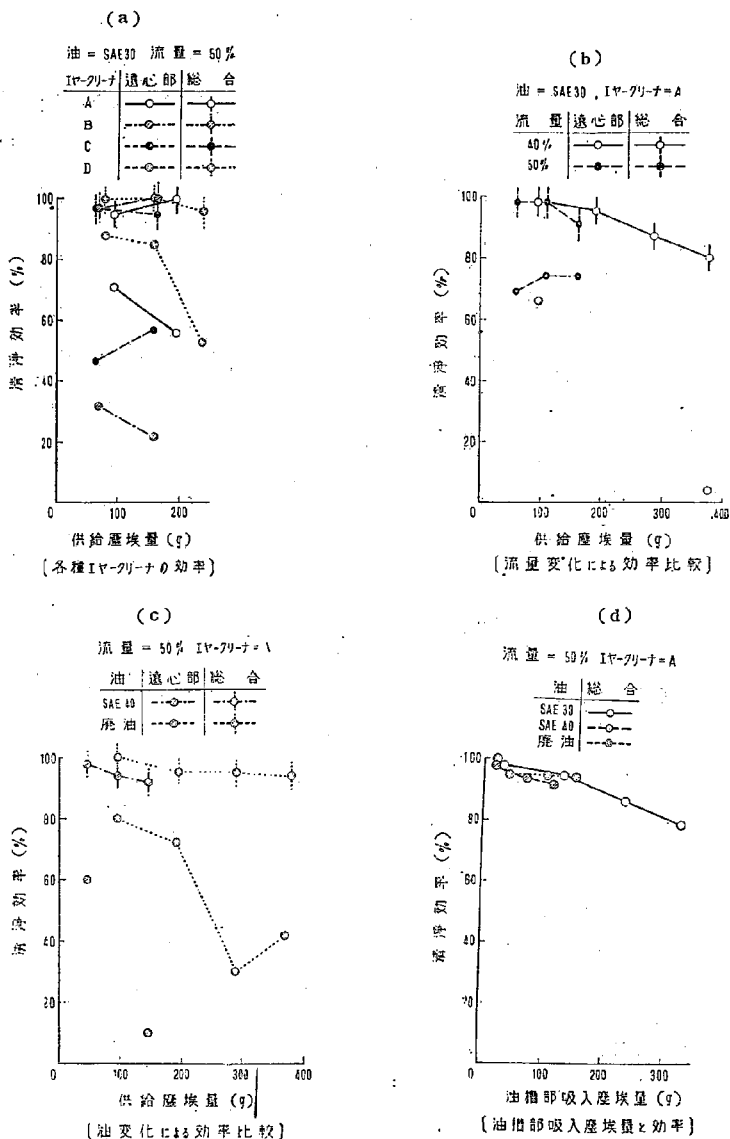
図-23 洗浄効率試験成績図
