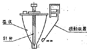
図-4 塵埃供給器
