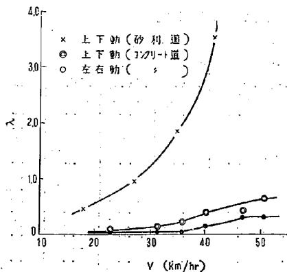
図-4 速度と \lambda の関係
