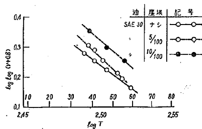
図—12 塵埃混入による粘度変化 (SAE 30)
