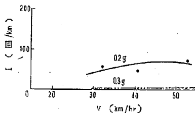
図-7・c V-I 曲線
