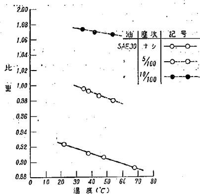
図一14 塵埃混入による比重変化 (SAE 30)
