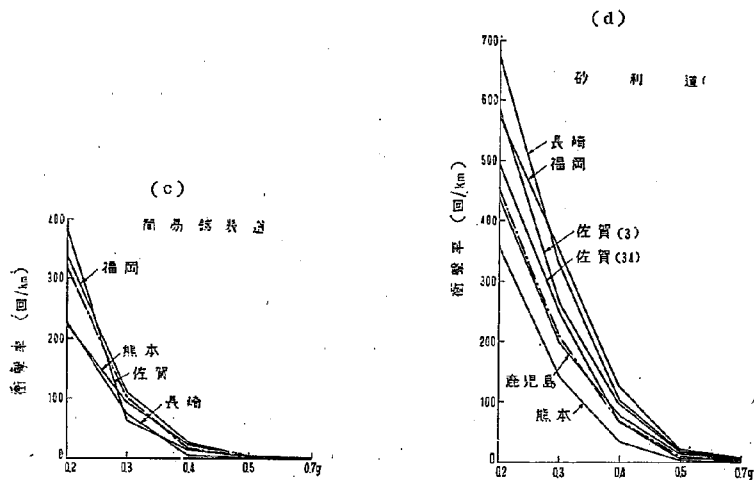
図-10 ベド・メーターによる各県の平均損傷率の分布
