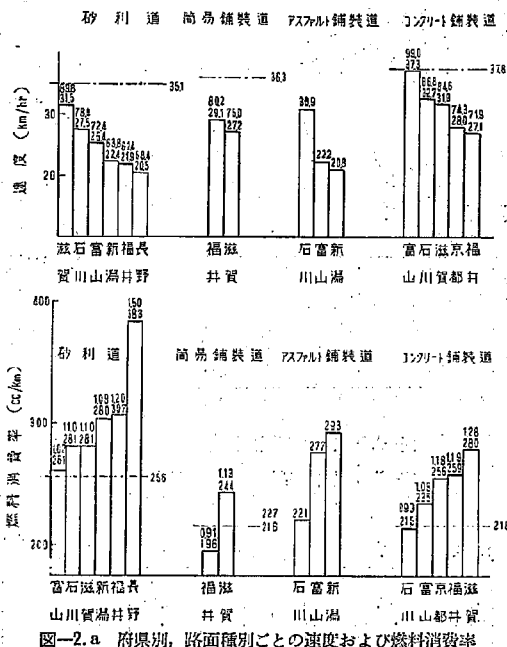
図-2. a 府県別、路面種別ごとの速度および燃料消費率
