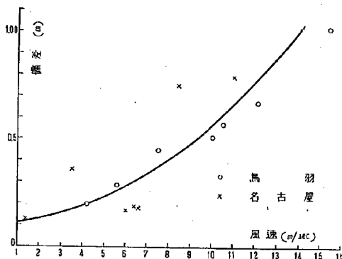
図-15 偏差と風速との関係
