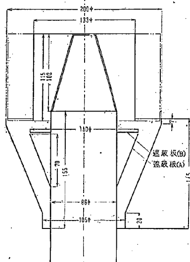
図-27 遠心部遮蔽板
