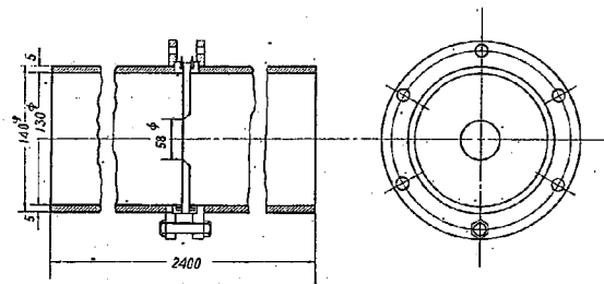
図-2 流量測定用オリフィス
