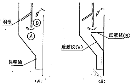
図-10 エアークリーナの遠心部
