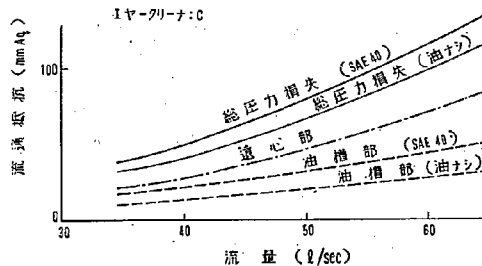
図-19 流通抵抗試験成績図 (C)
