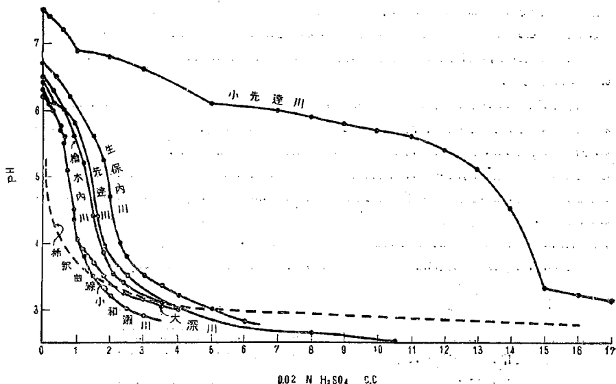
図—9 支川の滴定曲線 (100 c.c.)
