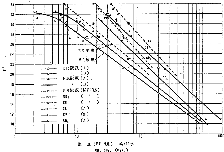
図—5 pH と酸度, Cl , SO_4
