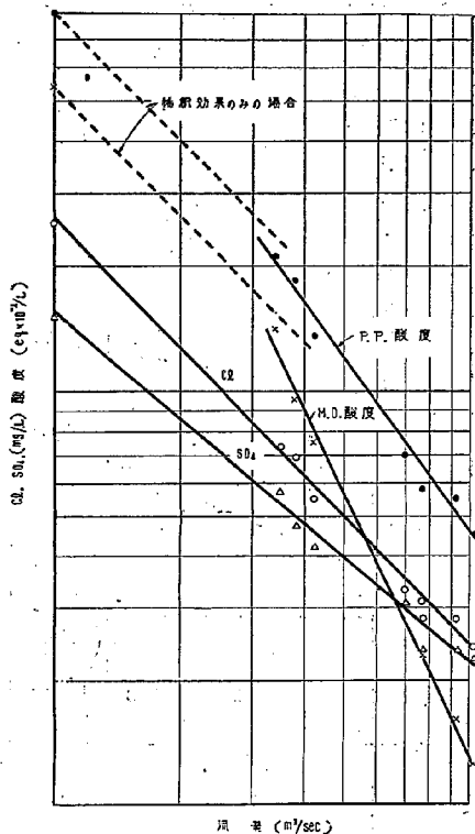
図-7 流量と水質(B)
