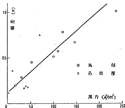
図-16 偏差と風力との関係
