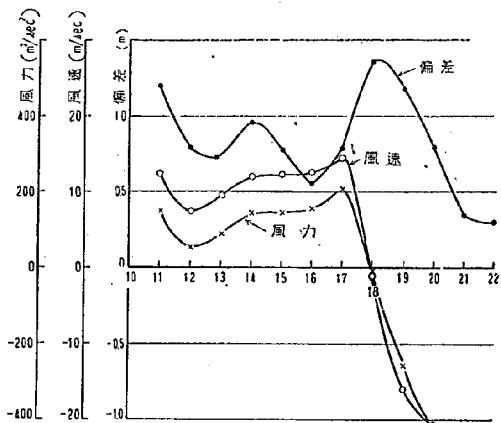
図-14 名古屋の偏差と風速、風力との相関
