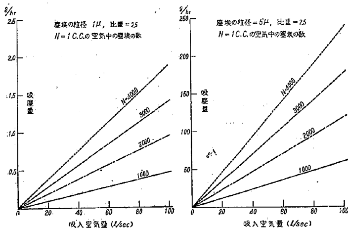
図-11 エアークリーナの吸塵量
