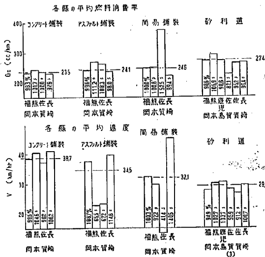
図-8 各県の平均燃料消費率
