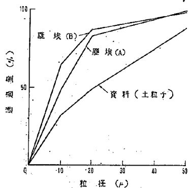
図-6 塵埃の粒度分布
