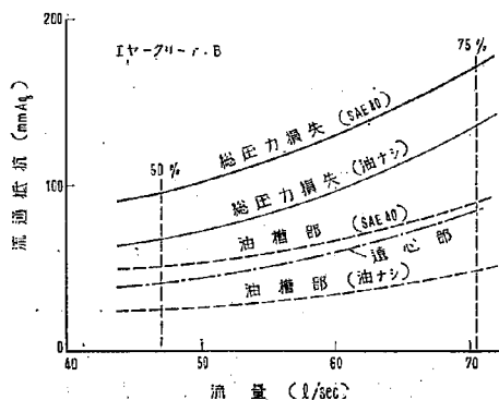
図-22 流通抵抗試験成績図 (F)
