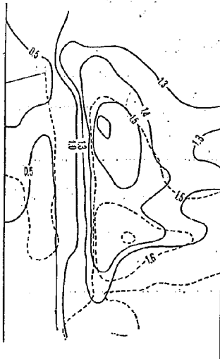
図-8 流速分布図 (流量 40 l/sec)
