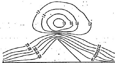
図-13 不透過斜 (45°) 水制 u 分布図
