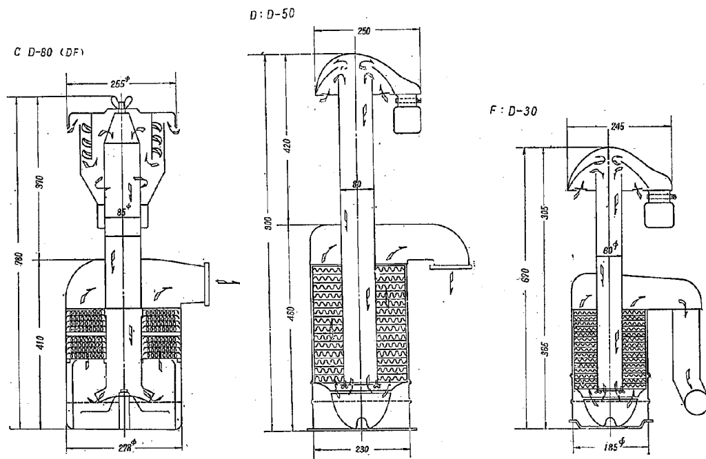
図—5 建設機械用エアークリーナ
