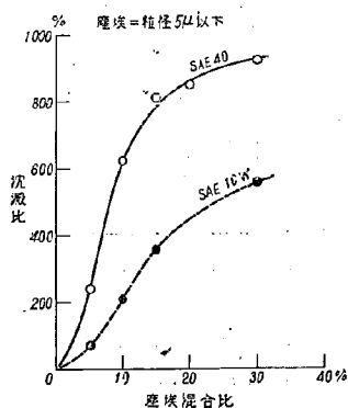
図一16 油中における塵埃の沈澱状況
