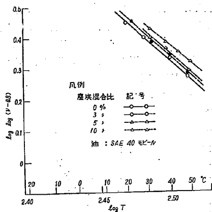
図一13 塵埃混入による粘度変化 (SAE 40)
