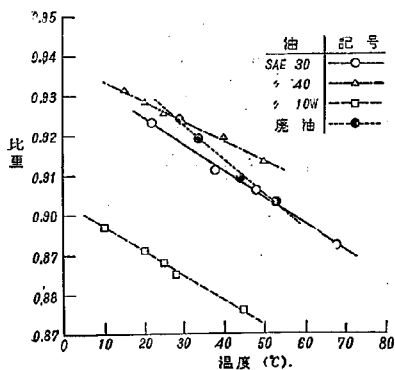
図-7 油の比重特性
