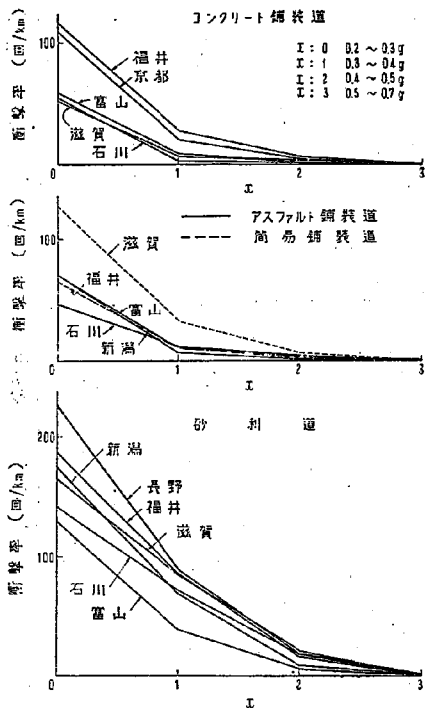
図-2. b 燃費率分布図
