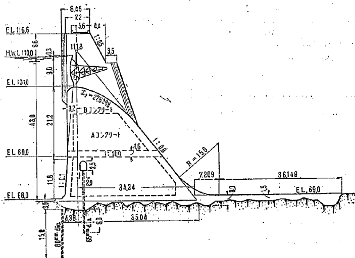
図-2 旭川第一堰堤標準断面 (単位m)
