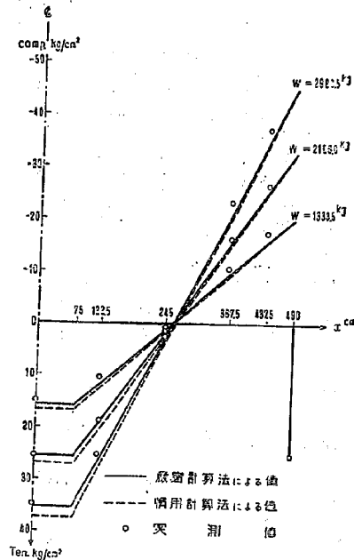
図-10 梁部下縁における応力
