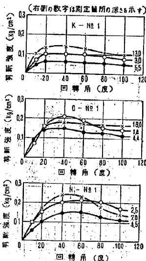
図-3 剪断強度と回転角の係
