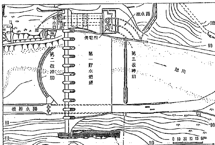
図-1 堰堤平面図
