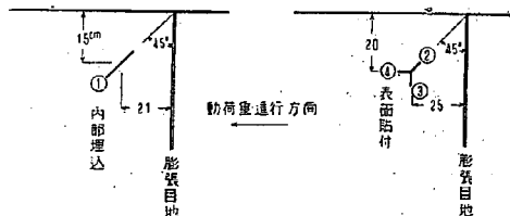
図-7 隅角部ゲージ位置
