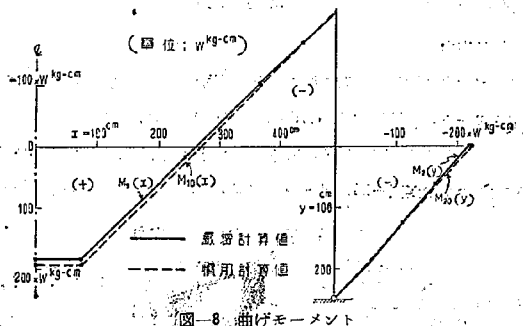
図-8 曲げモーメント
