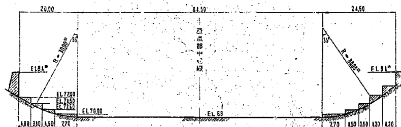
図-6 実験 No. 7 横断面図
