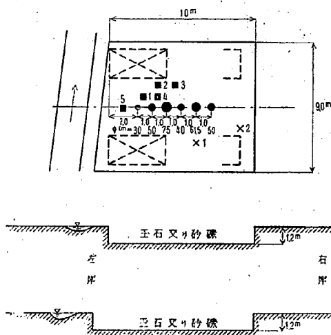
圖-2 (c) 砂川第5堰堤
