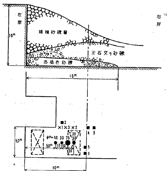
図一2 (b) 前入沢第8床固め
