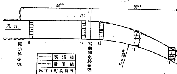
図-12 実験値と計算値の比較-1 (水面と底圧)
