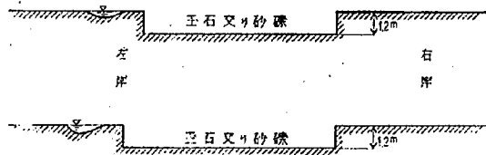
図-2 (c) 砂川第5堰堤
