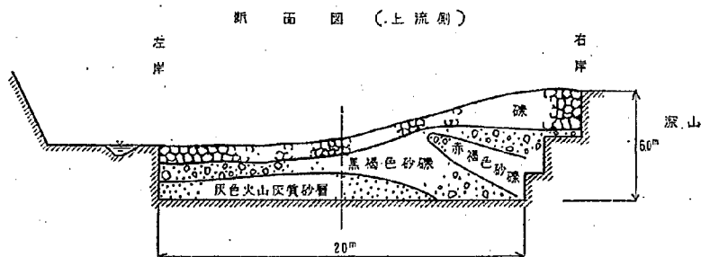
図-2 a) 深山第10床断面図
