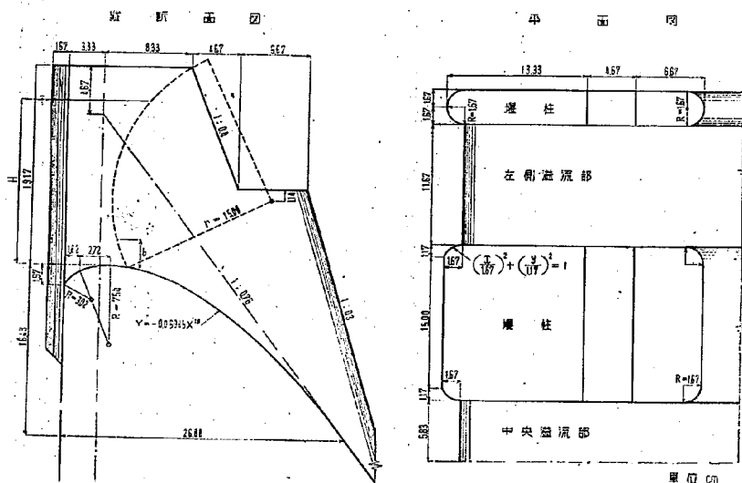
図-12 溢流部模形 (鋸細グム)
