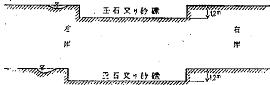
図-2 (c) 砂川第5堰堤
