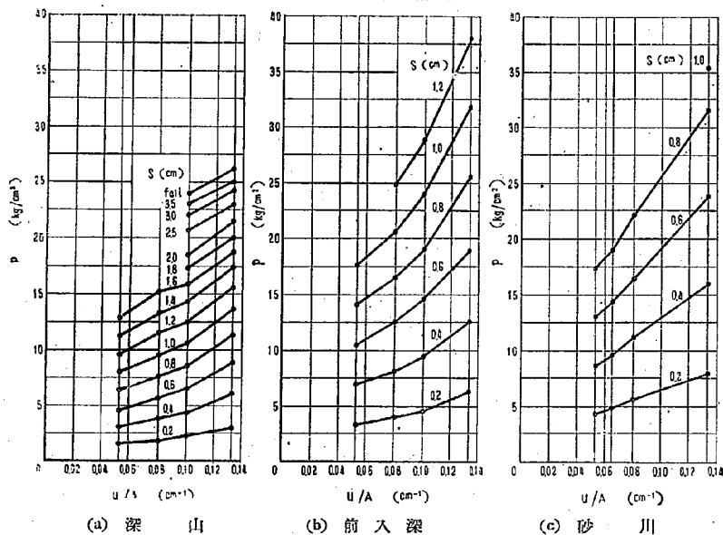
図-10 p_0 と u/A との関係
