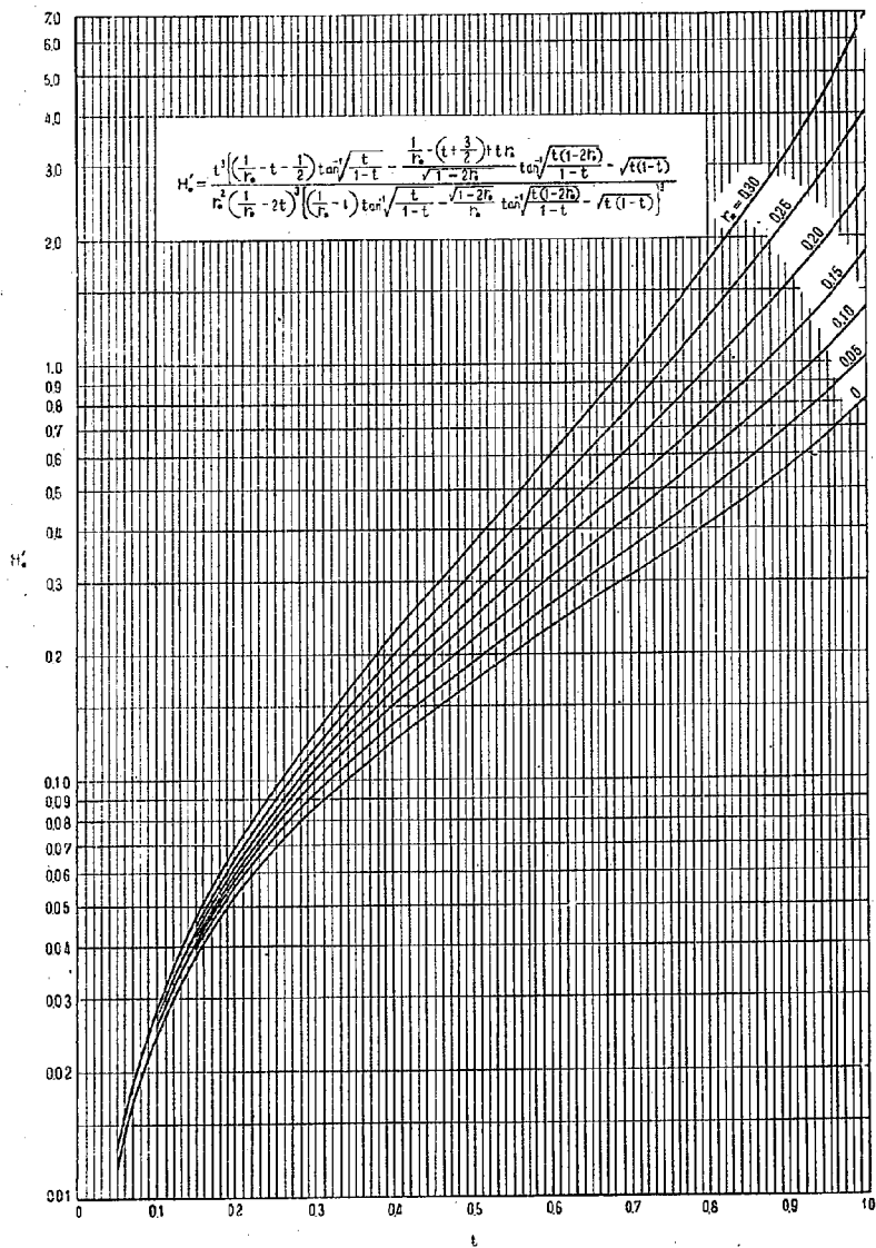
附圖—3 H_w \sim t, t_0 曲線
