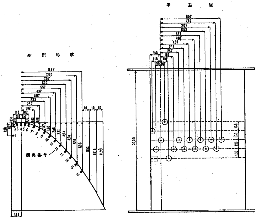
图-2 溢流部模型 (型式-1)
