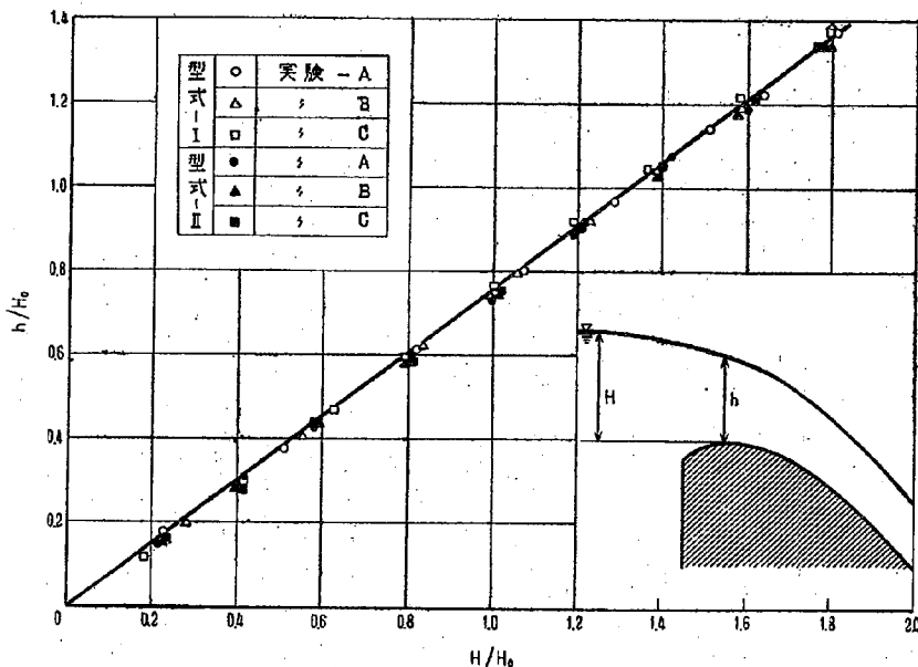
図—7 溢流深と溢流頂水深
