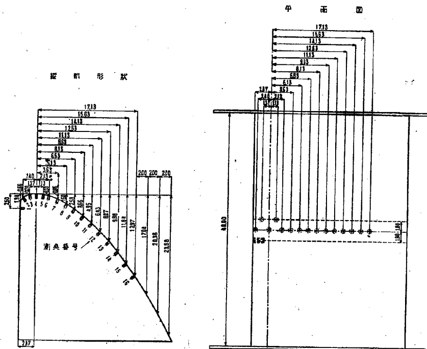
圖-3 溢流部模型 (型式-II)
