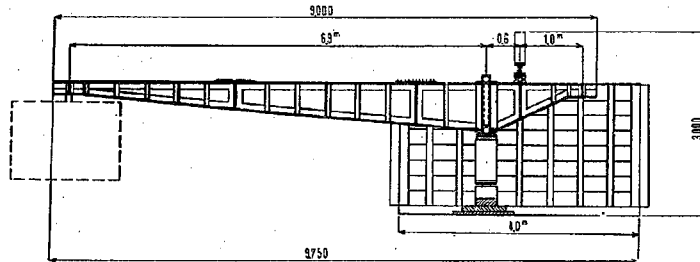
図-1 (b) 側断面図
