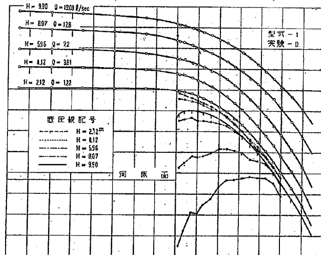
図-8 水面縦断形状と底面圧力 (型式-1)
