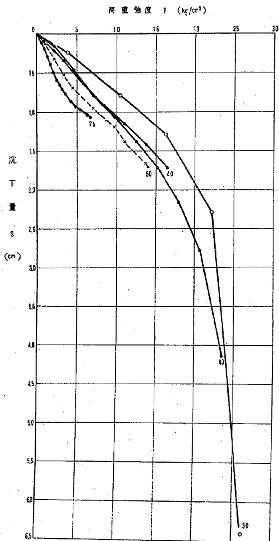
圖—8 載荷試驗結果—2
