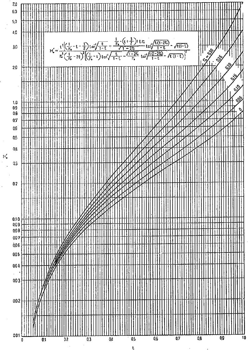
附圖—3 H_w \sim t 曲線
