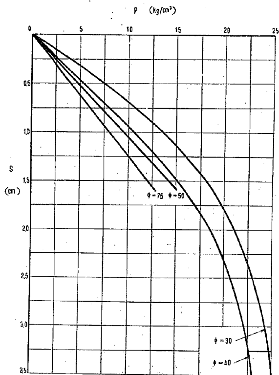
圖-9 載荷試験，修正曲線—3 (a) 深 山
