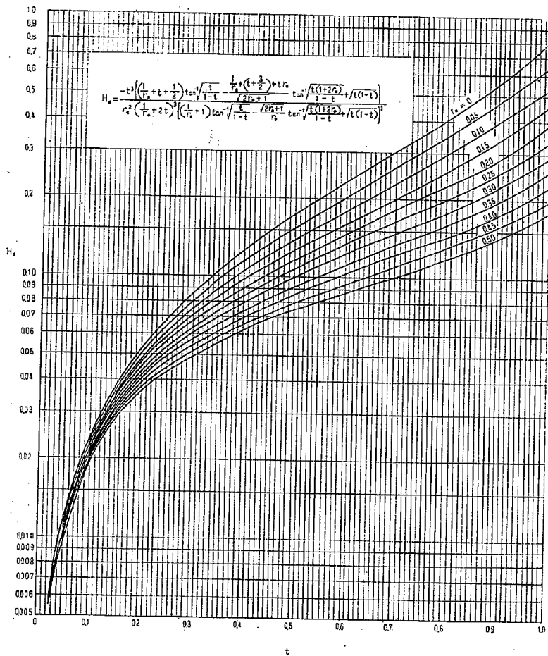
附圖—6 H_s \sim t, r_s 曲線
