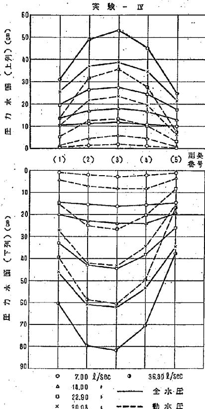
図-16 阻柱前面圧力
