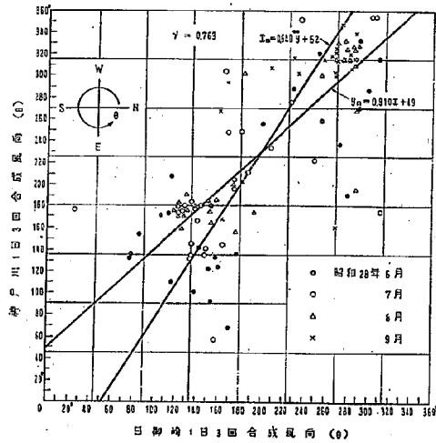
図一5 (b) 日御崎，神戸川河口の夏季風向の相関（1日3回）
