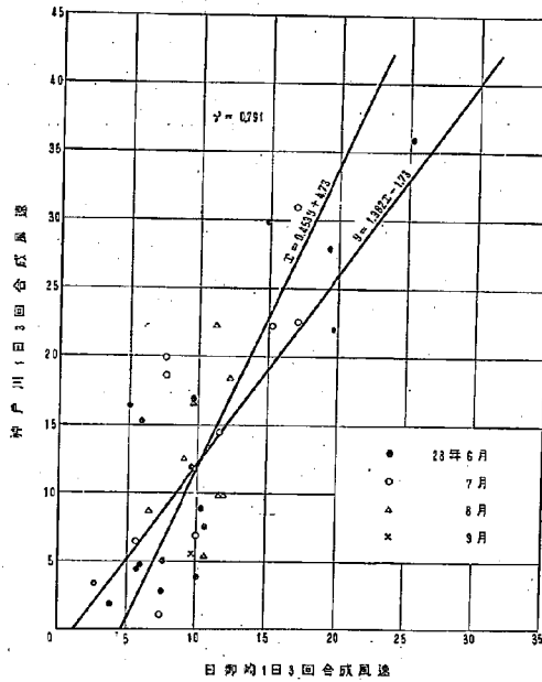
図一5 (a) 日御崎，神戸川河口の夏季海風風速の相関（1日3回）
