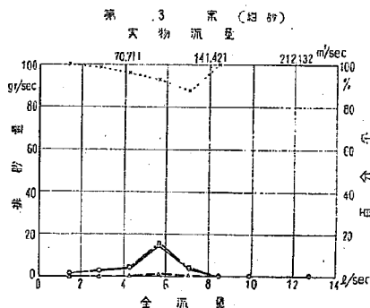
圖-11 排砂量分配圖
