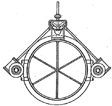
断面 A-A
