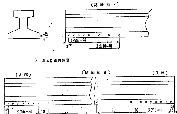
図-3 測定位置
