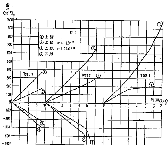
図-16-1 変みと荷重の関係
