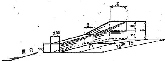
図一2 角形採雪筒の略図
