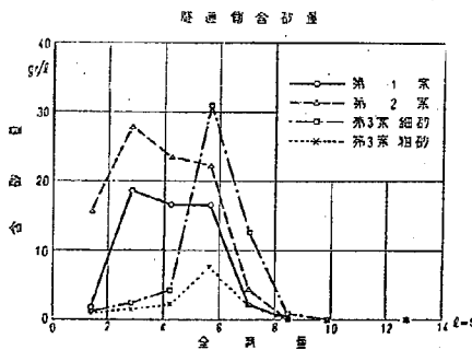
圖-12 含砂量圖
