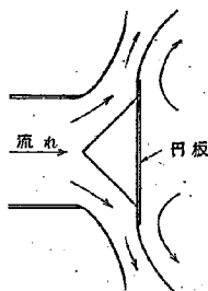
図-19 円板を取付けた場合の流況
