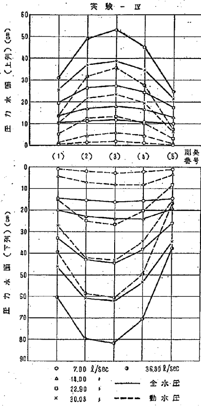
図-16 阻柱前面圧力
