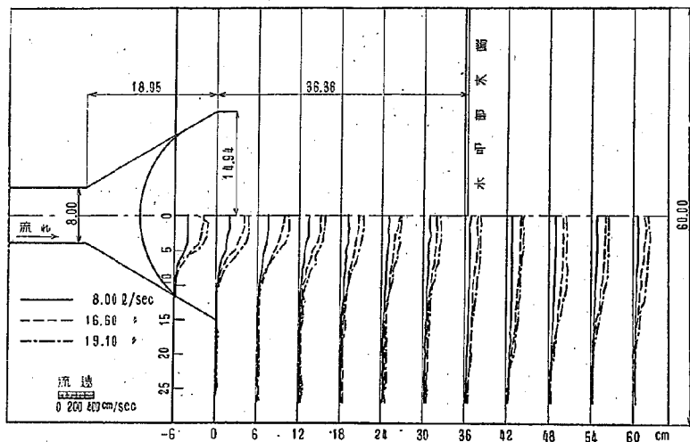
图-6 流速平面分布图
