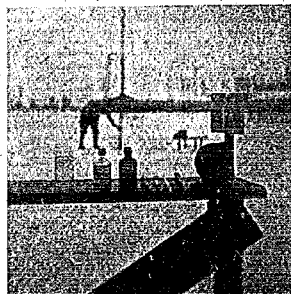
写真二 遠心分離器法による積雪の含水量測定器を測定台に取り付けた状況
