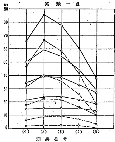
図-17 阻柱前面圧力
