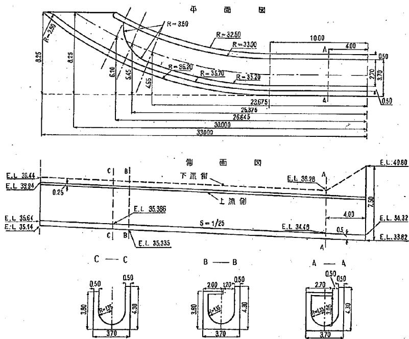
図-5. 排砂機構第3案
