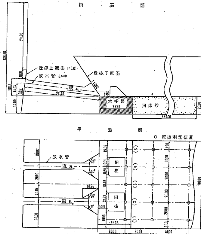
図—1 模型実験全体図 (藤井川防災ダム)
