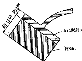
図-5 アバット附近に於ける水平断面
