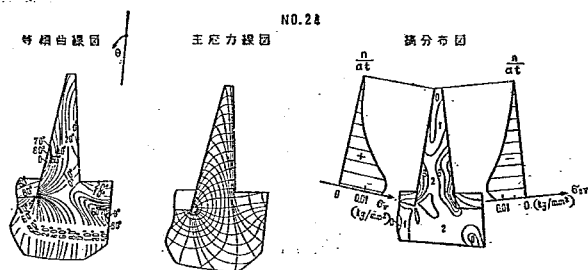
図-10-5 No. 24 に於ける等傾曲線, 主応力線, 綫分布及び縁応力分布
