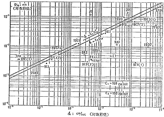
図-11 k と D_{10} との関係
