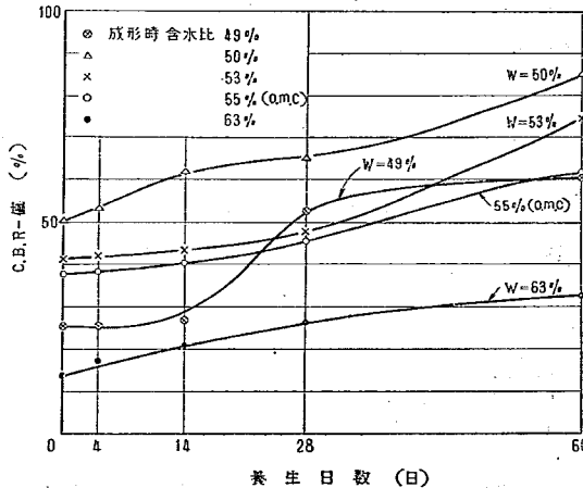
図-11. 石灰・フライ・アッシュ混合による関東ロームの C.B.R.-値 と養生日数との関係
