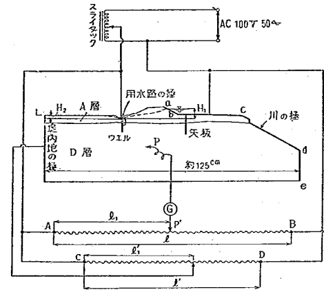
図-14 電気的模型略図
