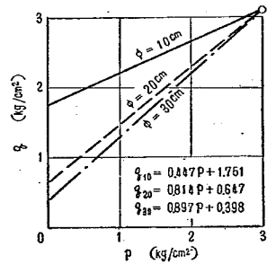
図-6 計算による p と q の関係
