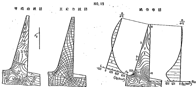
図-10-4 No. 19 に於ける等傾曲線, 主応力線, 綫分布及び縁応力分布
