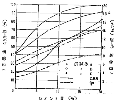
図一12 (1). セメント量と 7 日養生 C.B.R. および q_u -値 との関係
