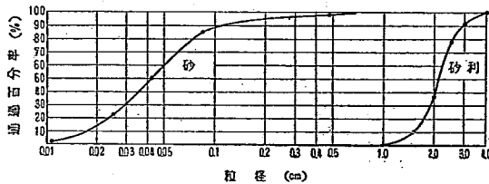
図-2 つめた試料の粒径分布
