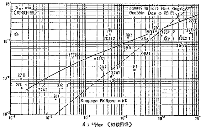
図-12 k と D_{20} との関係
