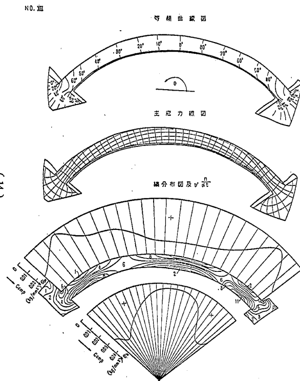
図—9-3 No. XII に於ける等傾曲線，主応力線，綫分布及び縁底力分布
