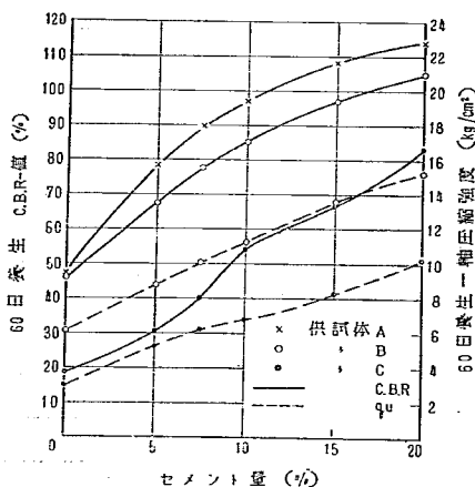
図—12 (2). セメント量と 60 日養生後の C.B.R. および q_u -値 との関係
