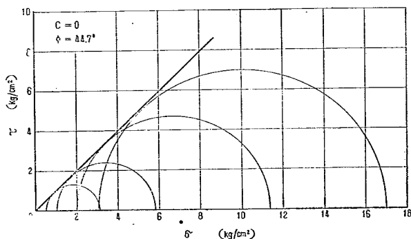
図—14 砂路盤材料の3軸試験結果
