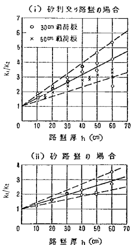
図-18 路盤厚が増加した場合の支持力係数の増加
