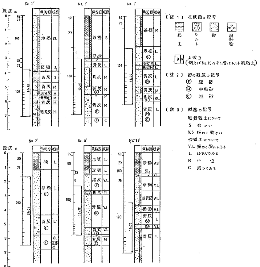
図—9 前年度調査区間に対する sounding 結果
