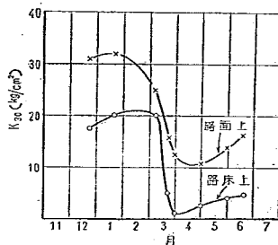
図-4 月別に測定した K_{30} の変化 (滝沢村において、東北地建、武田技官)
