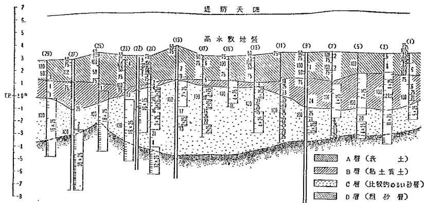
図-6 堤防法尻川表における sounding 結果
