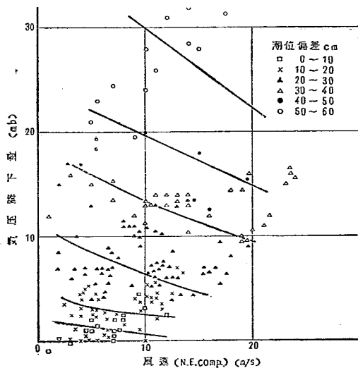
図-5 気圧降下量—風速—潮位偏差の關係
