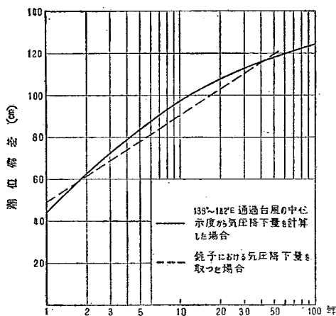
図-14 潮位偏差の確率
