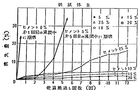
図-23. 乾湿繰返し試験に於ける繰返し回数と損失量との関係
