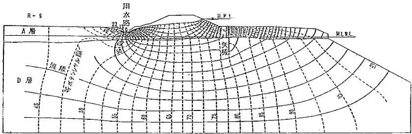
図-16 電氣的模型により求めた流線網の例（止水矢板を打ったもの）
