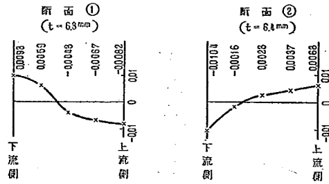
図-12 垂直断面 No. 14 における上下方向応力 \sigma_z の分布 ( \text{kg/mm}^2 ) (Compression を + とす)
