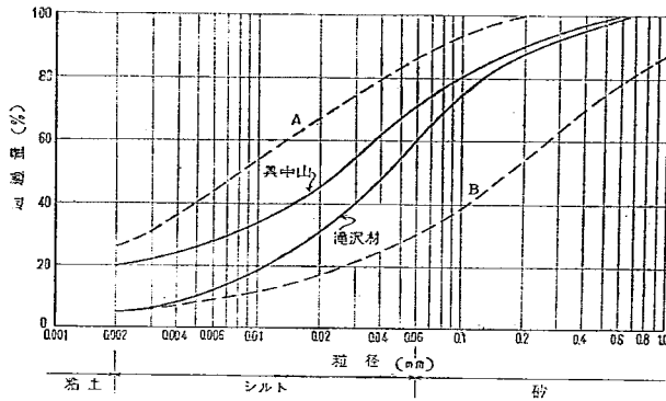
図一 凍上を受け易い土の範囲と調査地区における代表的な土の粒度分析試験結果
