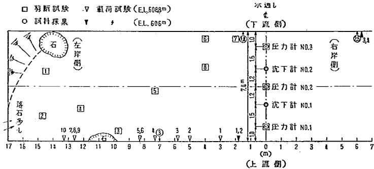
図—15 計器の据付と現場実験の位置砂川第4堤基礎平面)
