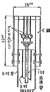
図—25 沈下計の頭部
