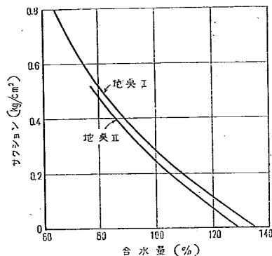
図-6 路床土のサクシオンと含水量の関係 (滝沢村)
