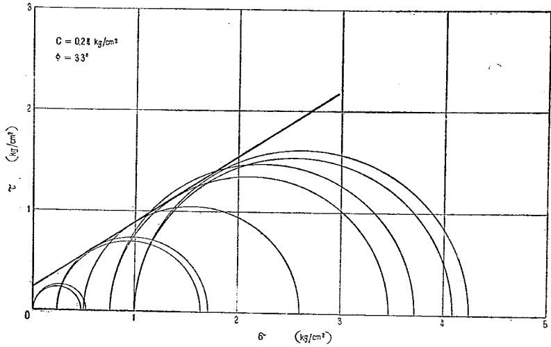
図一10 関東ローム路床土の3軸試験結果
