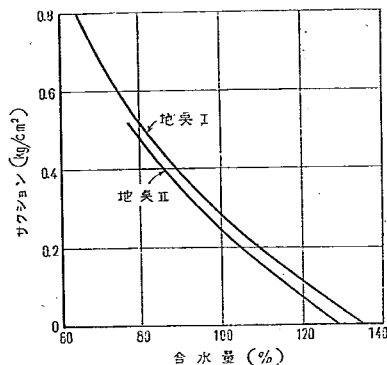
図-6 路床土のサクションと含水量の関係（滝沢村）
