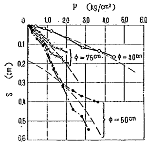
図-18 剪断強度 p と沈下量 s の関係
