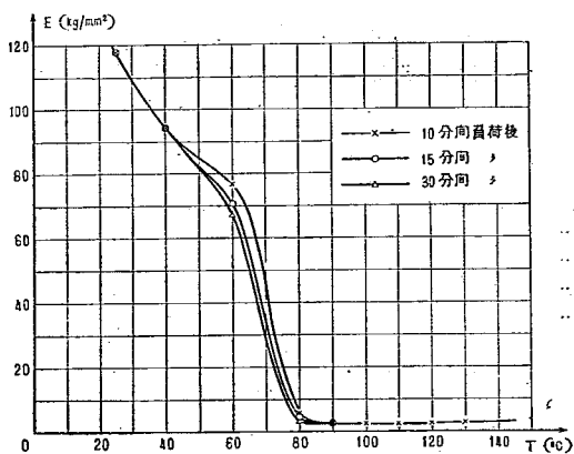
図-3 温度と Young 率との関係
