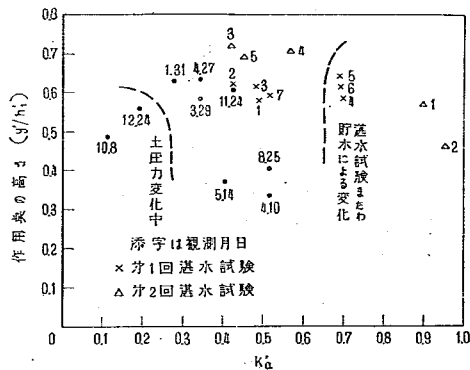
図-42 実測圧力の作用点の厚さとの全土圧 E_a を静水圧分布に置き替ふたときの土圧計数
