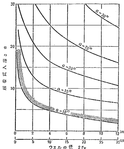
図-23 ウエルの径と所要貫入深さの関係
