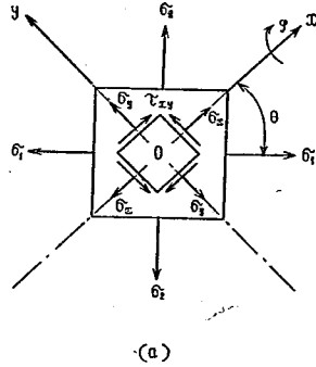
図—4 傾斜入射と二次主応力
