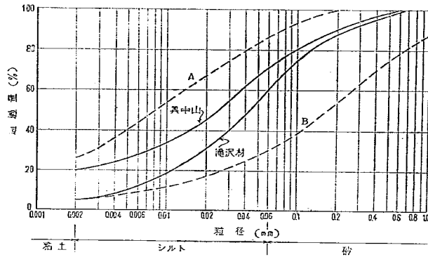
図-1 凍上を受け易い土の範囲と調査地区における代表的な土の粒度分析試験結果
