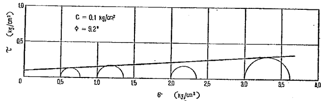
図一11 腐蝕土交りの関東ローム路床土の3軸試験結果
