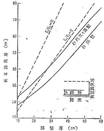
図-20 路盤厚と換算路床厚の関係
