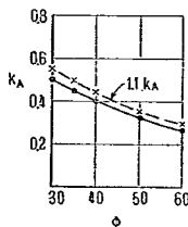
図—41 クーロンの土圧計数
