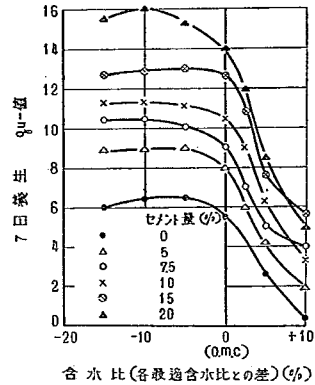
図一13 (2). 最適附近の含水比と7日養生一軸圧縮強度との関係
