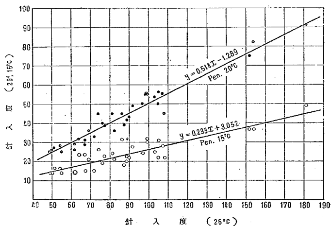
図-4. 針入度 (25°C)—針入度 (20°, 15°C) との関係 (100g・5秒)
