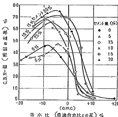
図—8. 最適含水比附近における締固め直後の C.B.R. 値
