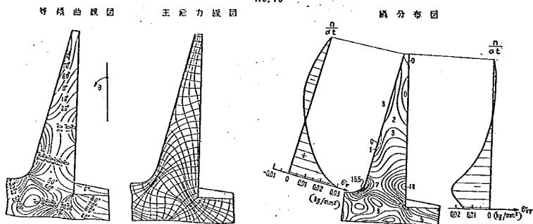
図-10-4 No. 19 に於ける等傾曲線, 主応力線, 綫分布及び縁応力分布
