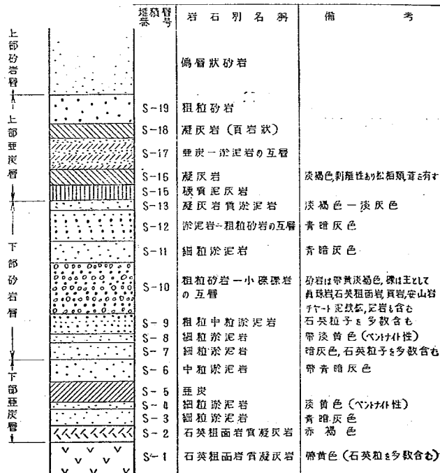
図-4 地上地帯小川層岩層略図
