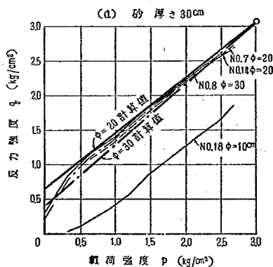
図—3 載荷重の増加による測定値の例
