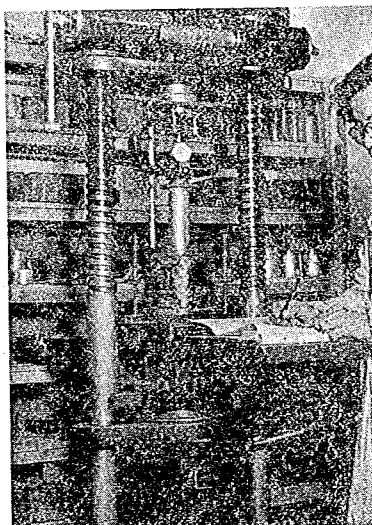
写真-4. C. B. R. 試験状況
