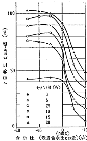
図一13 (1). 最適附近の含水比と7日養生 C.B.R.-値との関係
