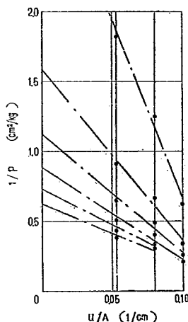
図-22 周辺面積比と 1/p の関係
