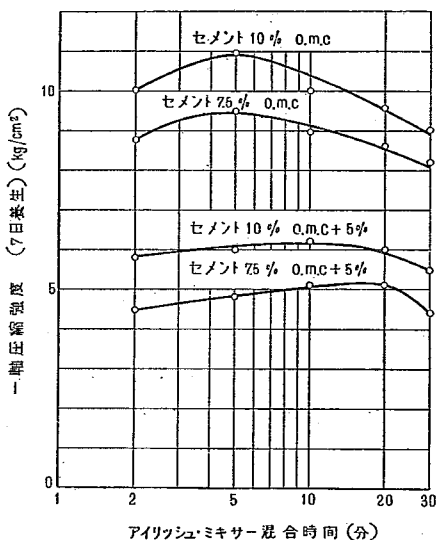
図-6. アイリッシュ・ミキサーの混合時と一軸圧縮強度との関係
