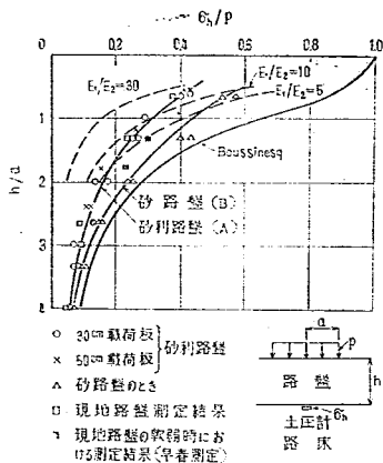
図-17 路盤と路床の境界における応力測定結果
