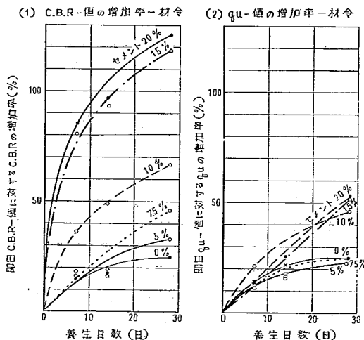
図-26. 供試体 D の養生日数と強度の増加率との関係
