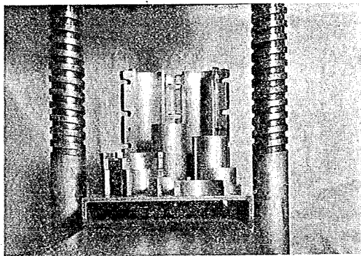
写真-9. q_u -供試体製作用モールド
