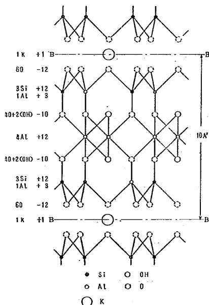
図-3 イライトの構造
