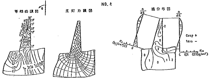
図—10-1 No. 4 に於ける等傾曲線、主応力線、縞分布及び縁応力分布
