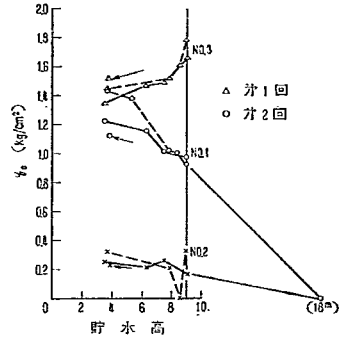
図—45 湛水試験中に於ける貯水厚と q_0
