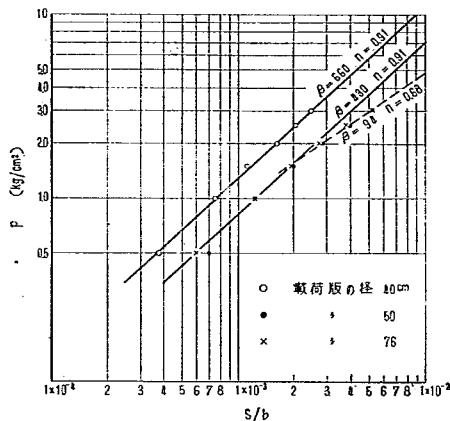
図-20 p と s/b との関係 (砂川第4堰堤)
