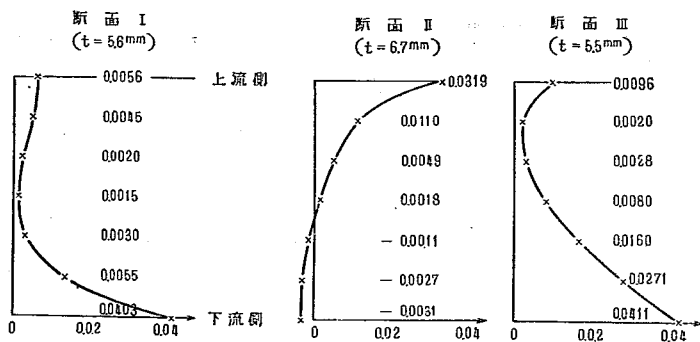
図-11 水平断面 No. VII に於ける \sigma_0 の分布 ( \text{kg/mm}^2 ) (Compression を + とす)
