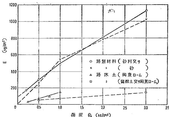
図-16 側圧と弾性係数の関係
