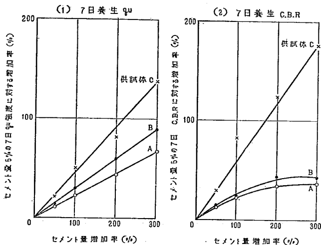
図-14. セメント量の増加率と強度の増加率との関係
