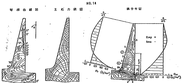
図—10-3 No. 14 に於ける等傾曲線、主応力線、縞分布及び縁応力分布
