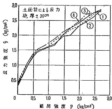
図-9 土圧計を鉄製函に取付けたときの p-q の関係
