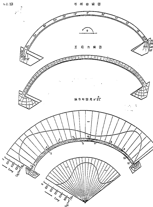
図—9-4 No. XVII に於ける等傾曲線，主応力線， \sigma/\sigma_0 分布及び \tau/\tau_0 分布
