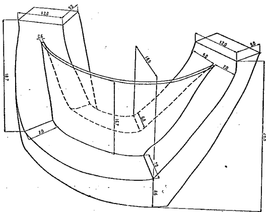
図-6 アーチ・ダム模型供試体
