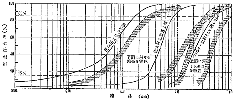
図-26 フィルター材料の選定
