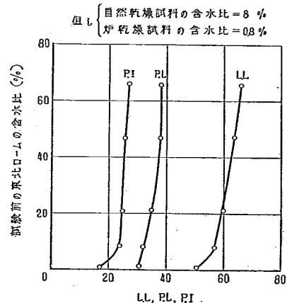
図-4. 東北ローム [A-7-5 (20)] の初期含水比による Consistency Limit の変化
