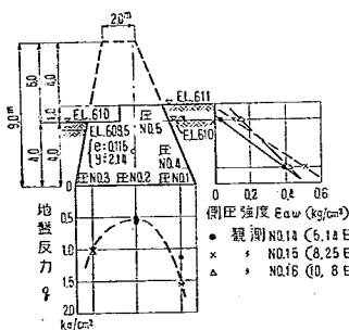
図-31 地盤反力及び側応力 (実測値)
