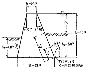
図—40 砂川第4堤堰の断面
