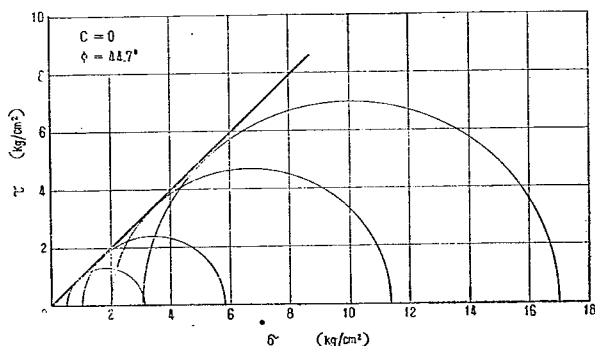
図—14 砂路盤材料の3軸試験結果
