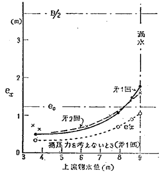
図-48 湛水試験中における合力の作用点
