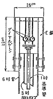
図—25 沈下計の頭部
