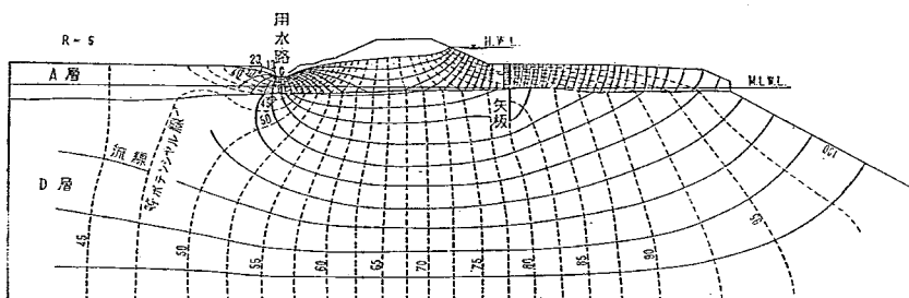
図-16 電気的模型により求めた流線網の例（止水矢板を打ったもの）
