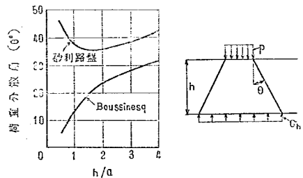
図-21 砂利路盤による荷重分散角
