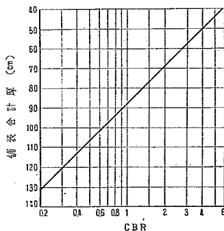
図-9 CBR の設計曲線の外挿
