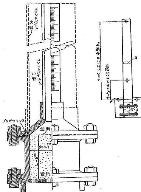
図-10 透水試験装置の略図
