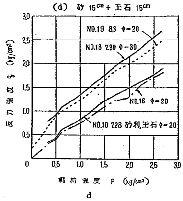
図-4 載荷強度 p と反力強度 q の関係
