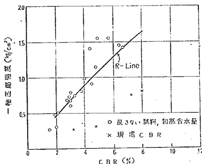
図-3 CBR と一軸圧縮強度の関係
