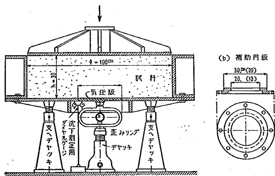
図-1 土圧計測定実験装置
