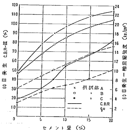
図—12 (2). セメント量と 60 日養生後の C.B.R. および q_u -値 との関係
