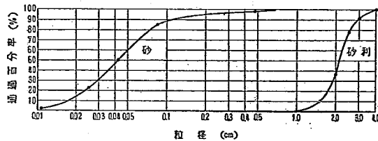
図-2 つめた試料の粒径分布
