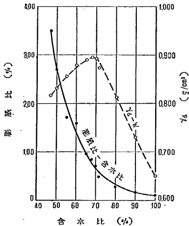
図-19. 4日水浸膨脹比と含水比との関係
