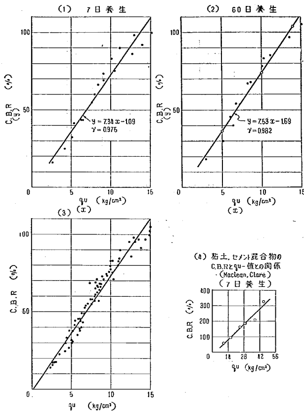
図—18. C.B.R.-値と q_u -値との関係
