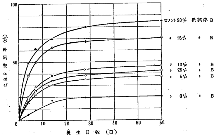
図-10. 即日の C.B.R.-値 に対する C.B.R. の増加率と養生日数との関係
