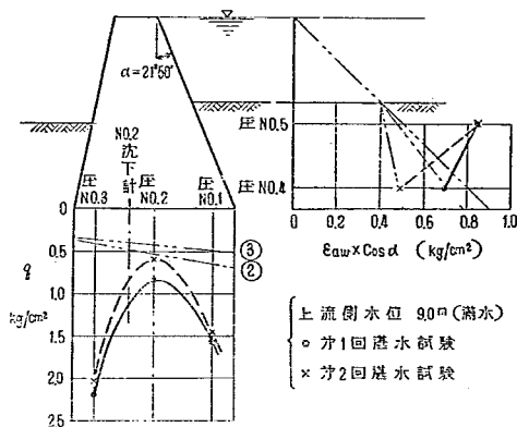
図—34 貯水により満水のときの反力
