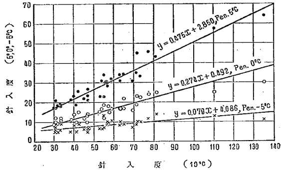
図-5. 針入度 (10°C)—針入度 (5°C, 0°C, -5°C) との関係 (200 g・60 秒)
