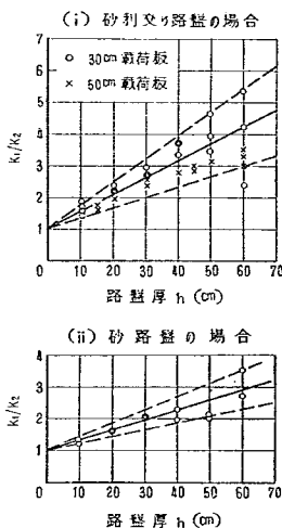
図-18 路盤厚が増加した場合の支持力係数の増加
