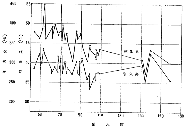
図一2. 針入度—軟化点、引火点との関係
