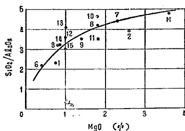
図-8 \text{SiO}_2/\text{Al}_2\text{O}_3 と \text{MgO} の関係
