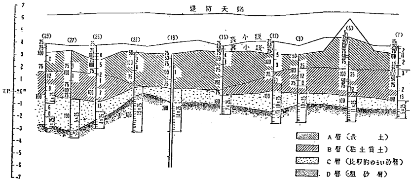
図—7 堤防法尻裏ける sounding 結果
