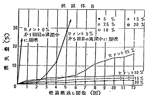
図-23. 乾湿繰返し試験に於ける繰返し回数と損失量との関係
