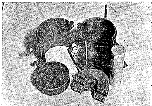
写真-8. 主要な C.B.R. 試験装置
