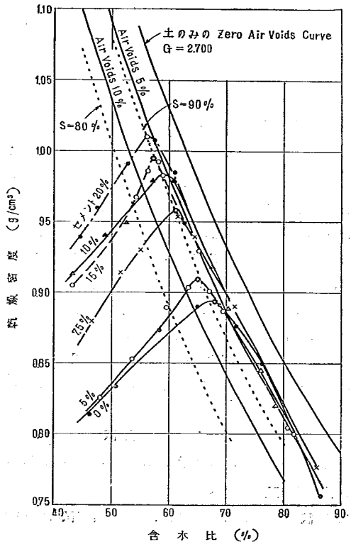
図-7. 締固め試験結果
