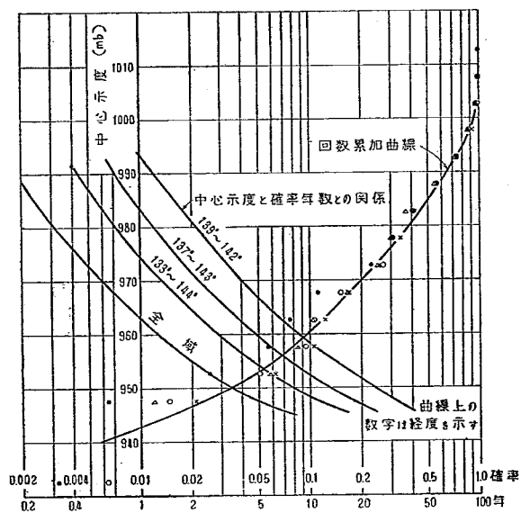
図-8 35°N を通過する示度の確率 (大正元年昭和 26 年)
