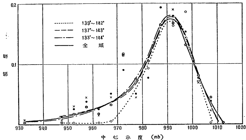
図-7 35°N 通過台風中心示度の頻度分布
