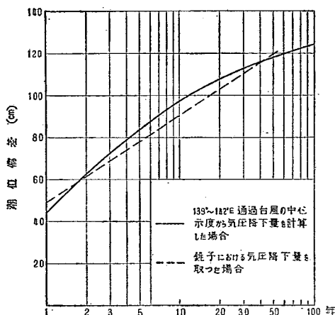
図-14 潮位偏差の確率
