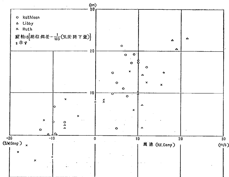
図-2 風向と潮位偏差との関係
