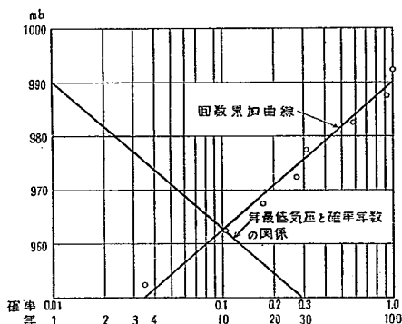
図-10 銚子年最低気圧の確率
