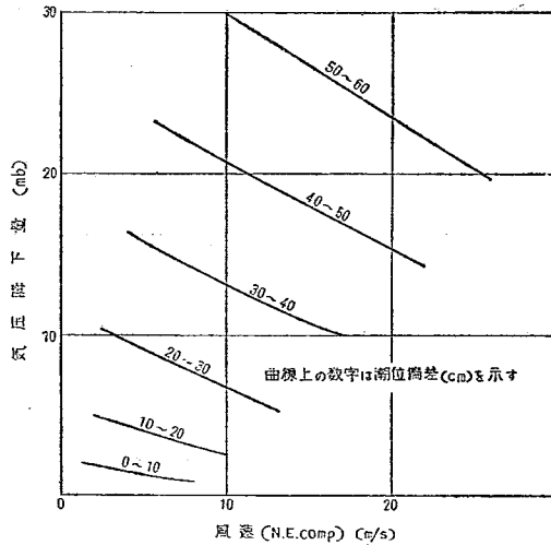
図-6 気圧降下量-風速-潮位偏差の相関関係
