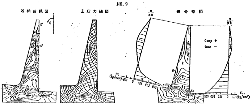
図—10-2 No. 9 に於ける等傾曲線、主応力線、縞分布及び縁応力分布
