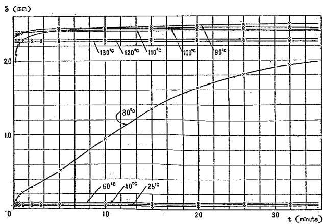
図-2 中央集中荷重 1kg に対する負荷時間と撓み \delta_1 との関係
