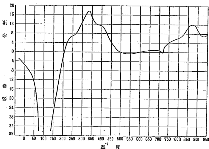
図-2. 関東ロームのコロイドの示差熱分析結果
