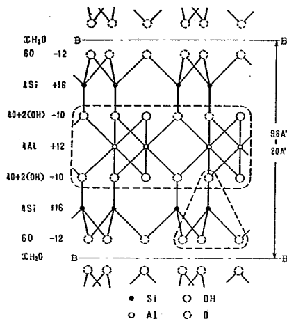
図-2 モンモリロナイトの構造
