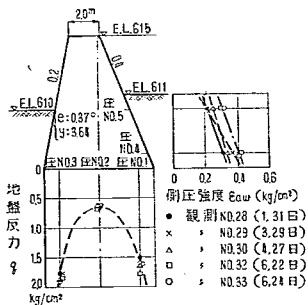
図-31 地盤反力及び側応力 (実測値)
