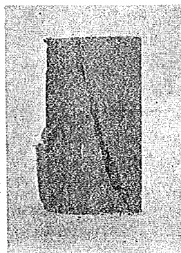
写真-6. 一軸圧縮用供試体の破壊状況 セメント 15%, 供試体 B, 養生日数 0日
