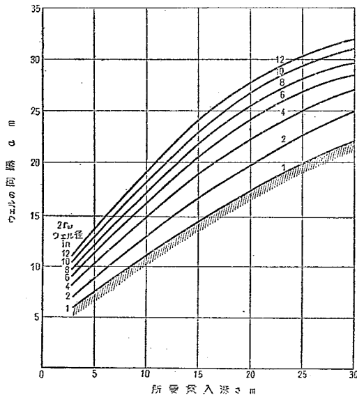
図-24 ウエルの間隔と所要貫入深さとの関係
