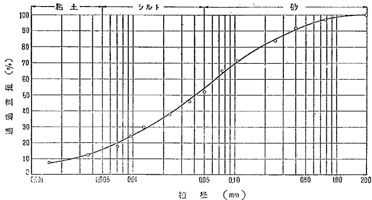
図-1. 使用した関東ロームの粒度
