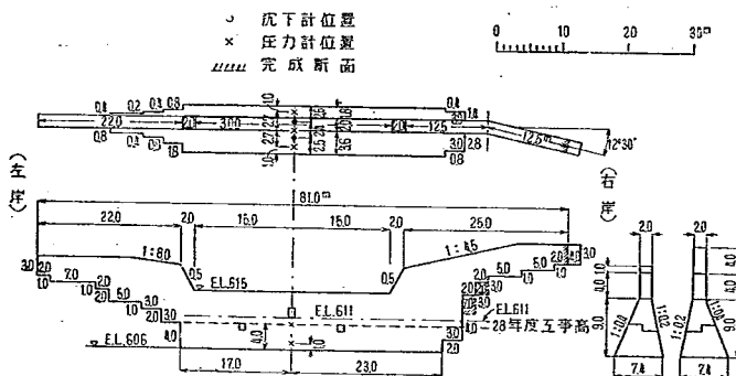
図—24 砂川第4砂防堰堤及び計器の位置
