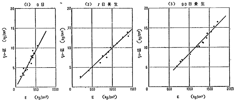
図-17. 弾性係数 (E) と一軸圧縮強度 ( q_u ) との関係
