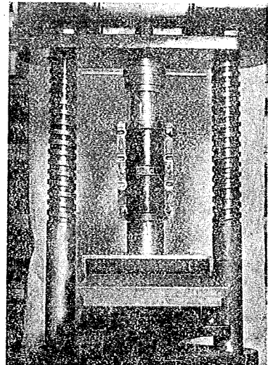
写真-3. 一軸圧縮試験用供試体作製状況
