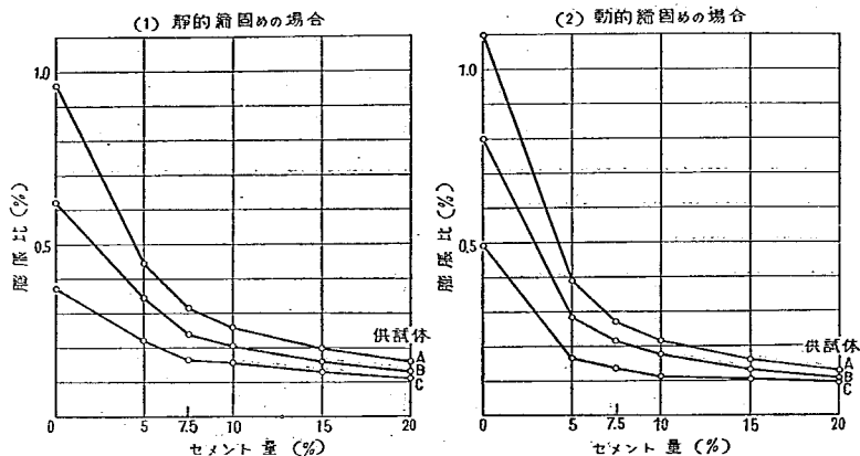
図-21. セメント量と膨脹比との関係
