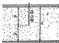
図一19 止水矢板の効果
