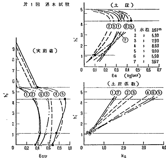
図一38 第1回湛水試験
