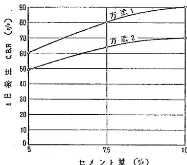
図-5. 関東ロームにセメントを加える方法の相違による C.B.R.-値の変化
