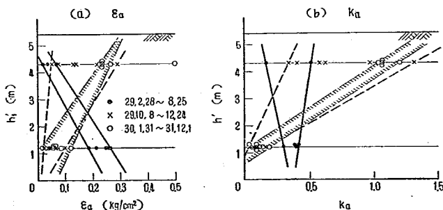
図-37 観測時期によつて区分した \epsilon_a 及び k_a
