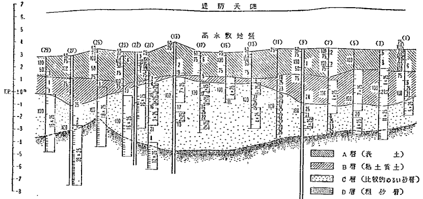
図—6 堤防法尻川表における sounding 結果
