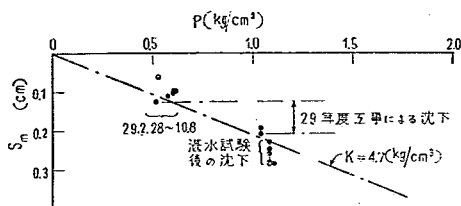
図-47 堤体の荷重強度 p と沈下 s_m の関係
