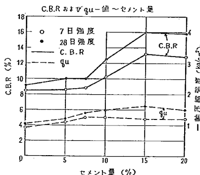
図-27. セメント量と強度 (7 日および 28 日) との関係
