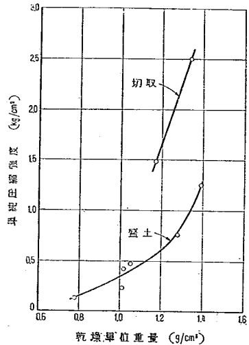
図-8 奥中山盛土箇所における乾燥単位重量と単純圧縮強度との関係
