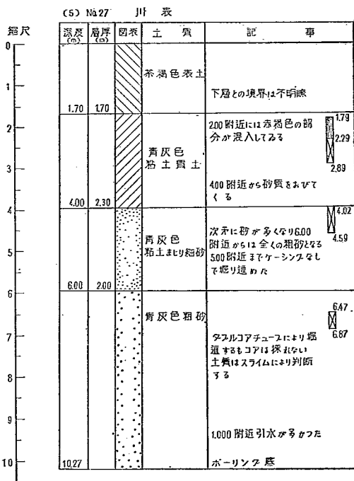
図-5-5 ボーリングによる土質柱状図および観察事項
