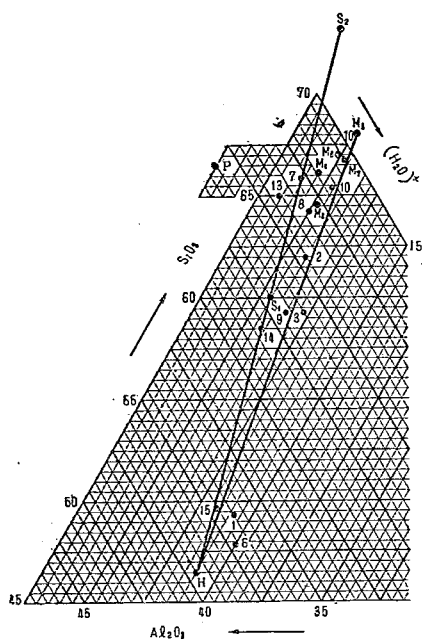
図—6 \text{SiO}_2\text{-Al}_2\text{O}_3\text{-(H}_2\text{O)}^{+3} 成分系図
