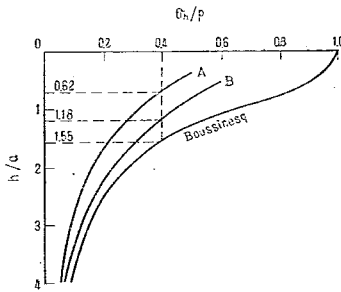
図-19 換算路床厚の求め方
