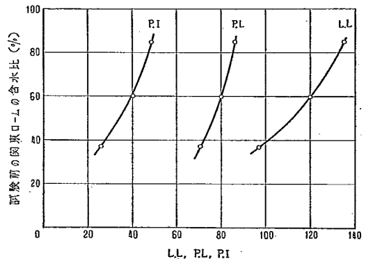
図-3. 関東ロームの初期含水比による Consistency Limit の変化
