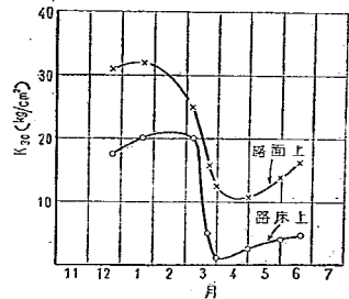
図-4 月別に測定した K_{30} の変化 (滝沢村において、東北地建、武田技官)
