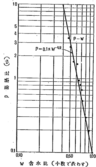
図-20. 膨脹比と含水比との関係
