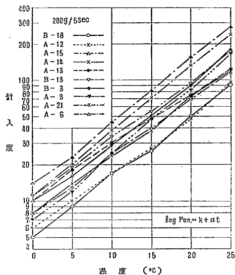
図-3. log Pen—温度との関係
