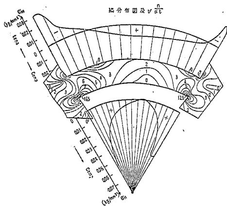
図-9-1 No. IV に於ける等傾曲線, 主応力線, 応分布及び終端力分布
