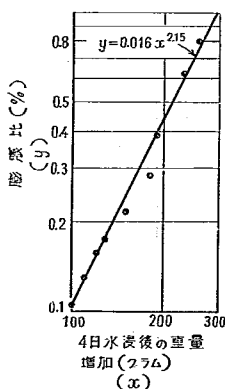
図-22. 膨脹比と供試体の重量の増加量との関係
