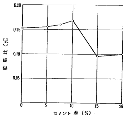
図-28. 供試体 D のセメント量と膨脹比との関係
