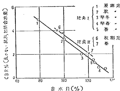
図-5 自然含水量と CBR の関係（滝沢村）
