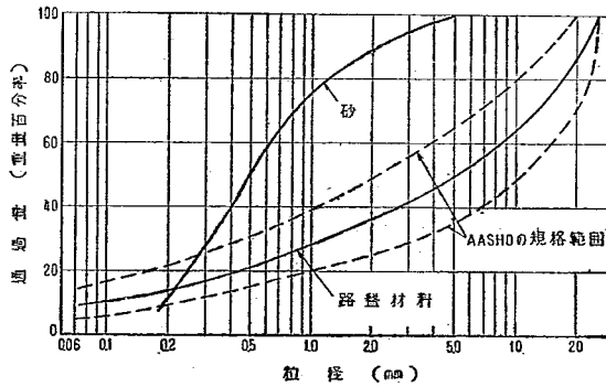
図一12 使用材料の粒径加積曲線
