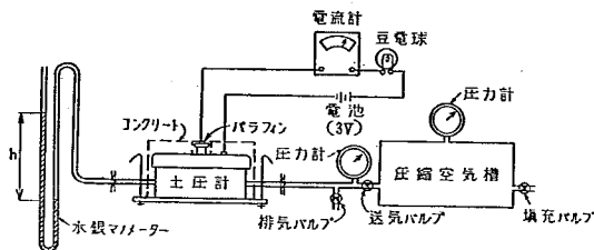
図-12 反力測定説明図
