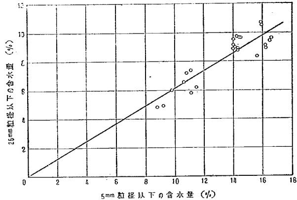
図—15 路盤材料全部の含水量と路盤材料の中、4 番篩通過の材料の含水量との関係
