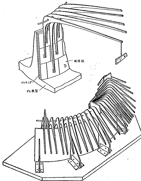
図-8 荷重装置概念図
