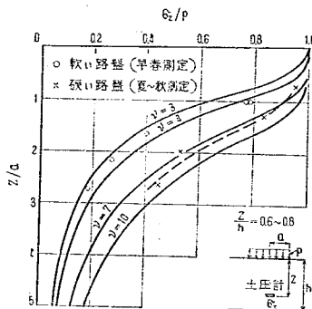
図-22 砂利路盤中の応力測定結果
