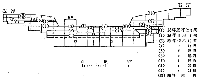
図—26 堤体コンクリート打工程
