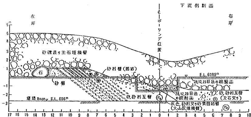
図—14 掘削面の地層
