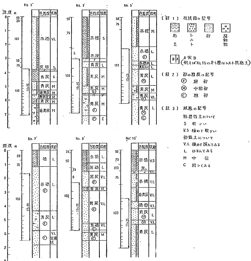
図-9 前年度調査区間に対する sounding 結果
