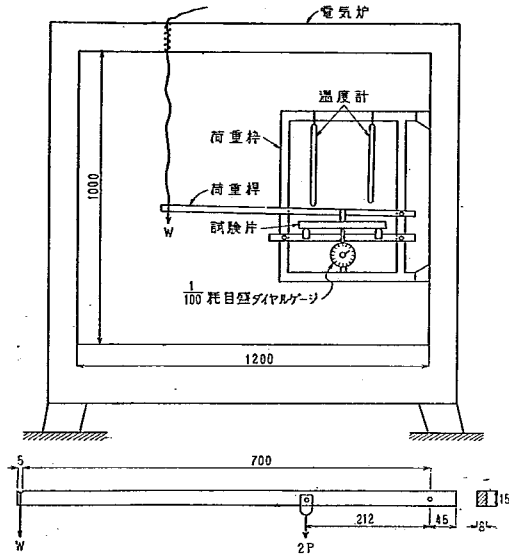
図-1 撓み測定要領と荷重棒
