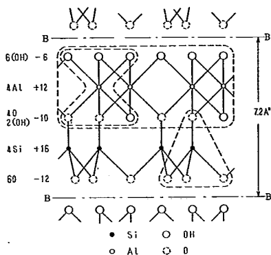
図-1 カオリナイトの構造
