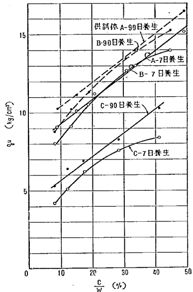
図-15. C/W Ratio と一軸圧縮強度との関係
