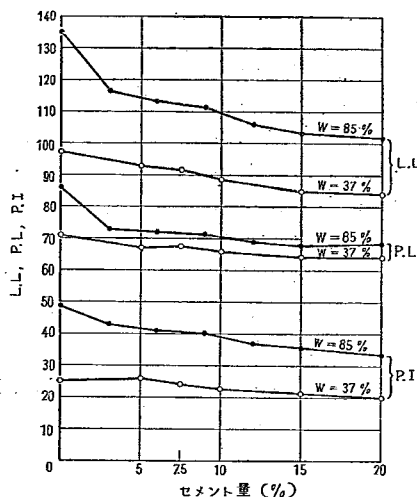
図—29. 混合直後のセメント量と Consistency limit との関係
