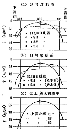
図-44 地盤反力の分布
