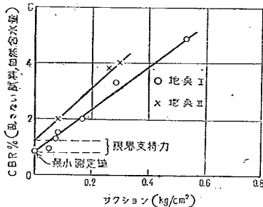
図-7 路床土のサクシヨンと CBR の関係
