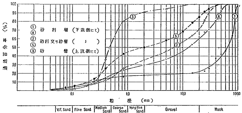
図—16 砂川第4砂防堰堤建設地基礎地盤粒度分布曲線
