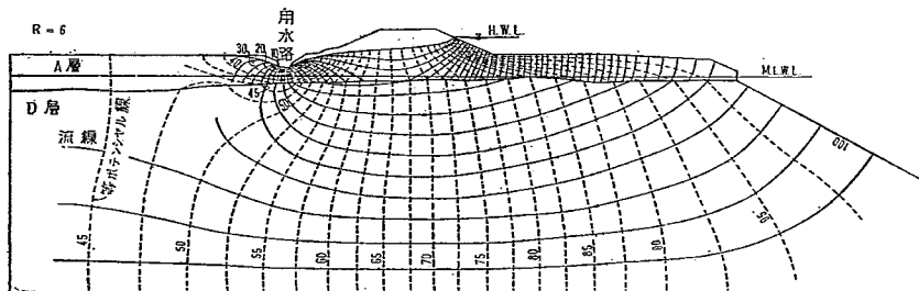
図-15 電気模型により求めた流線網の例
