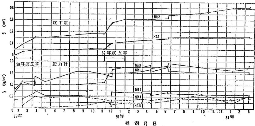
図-27 地盤反力及び沈下量(実測値)
