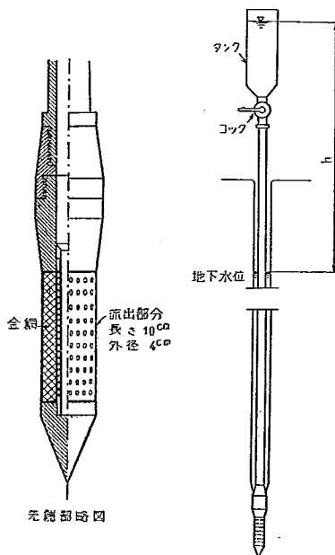
図-3 現場透水試験機
