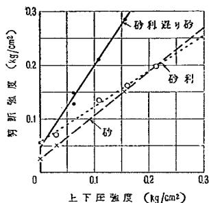
図—17 現場せん断試験結果
