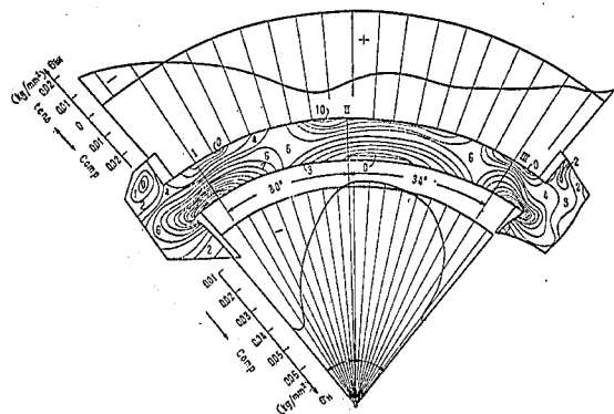
図-9-2 No. VII に於ける等傾曲線, 主応力線, 応分布及び終端力分布
