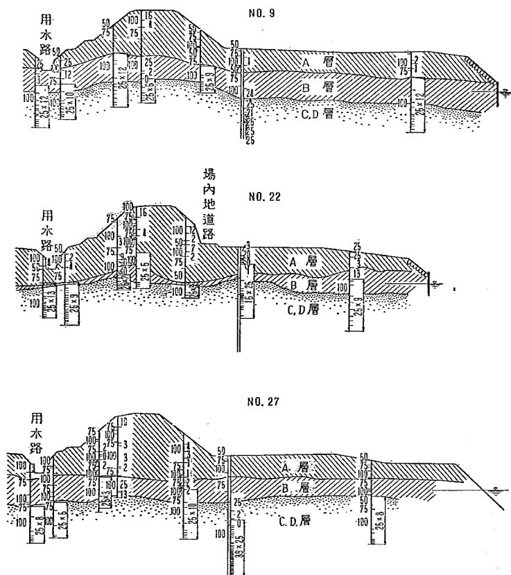
図-8 堤防の3横断面における sounding 結果
