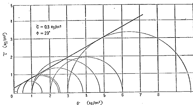
図—13 砂利路盤材料の3軸試験結果 (大型3軸試験器)
