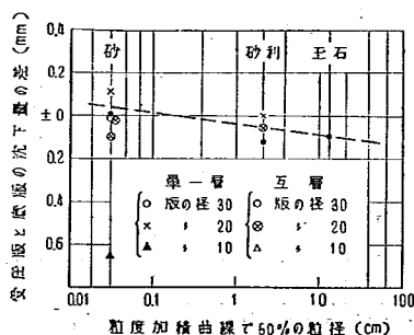
図-7 粒度と受圧版と底版の変位差
