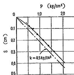
図-23 p = 1/a と沈下量との関係
