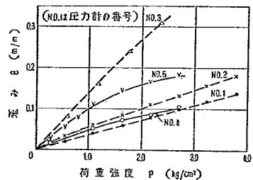
図-11 圧力計の受圧面への荷重と歪みの関係
