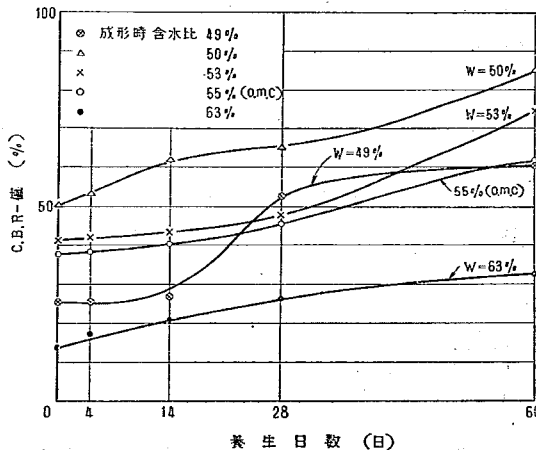
図-11. 石灰・フライ・アッシュ混合による関東ロームの C.B.R.-値 と養生日数との関係
