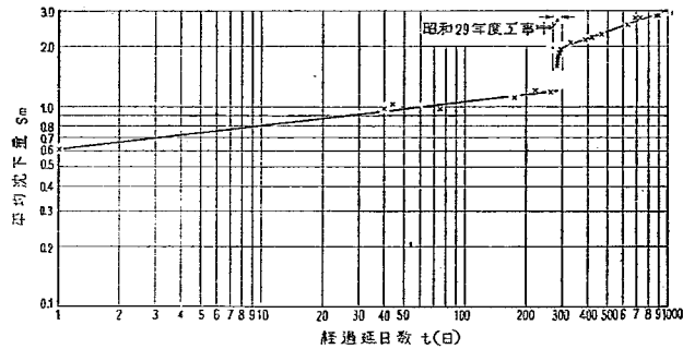
図—46 堤体の経過時間と平均沈下量
