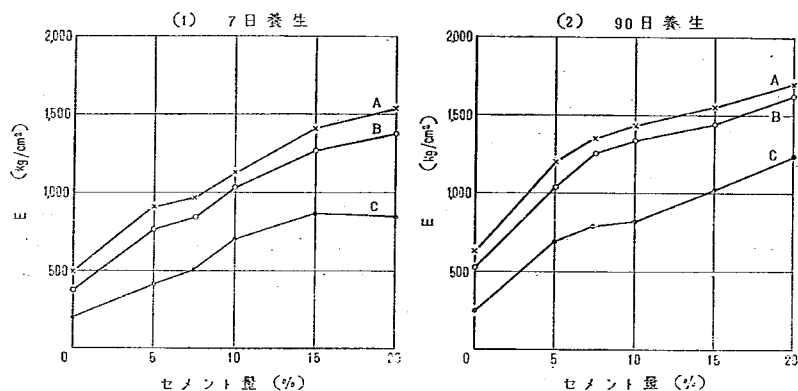
図—16. E とセメント量との関係
