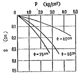
図-19 載荷板径の相違による p-s 曲線
