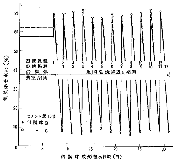
図-24. セメント量 15% の供試体 B および C の乾湿繰返し試験中の含水比の変化
