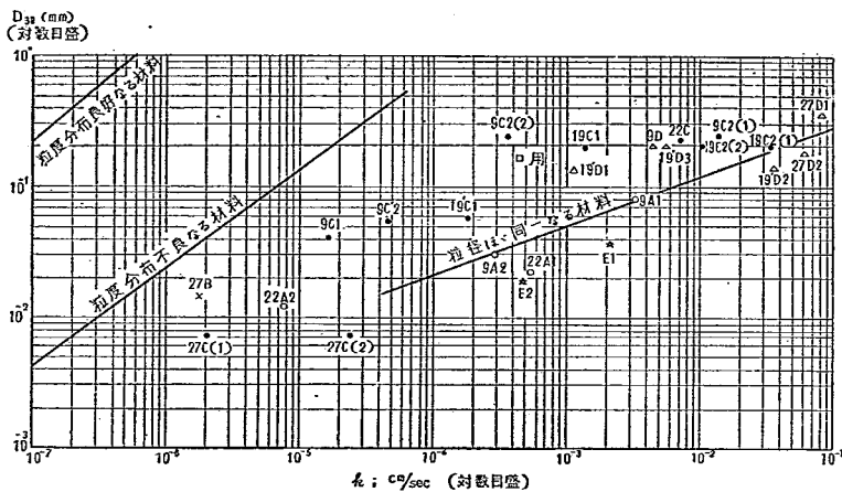
図-13 k と D_{30} との関係
