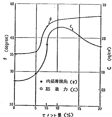
図-25. 三軸圧縮試験結果、セメント量、内部摩擦角 ( \phi ) および粘着力 ( C ) との関係 (供試体 C)
