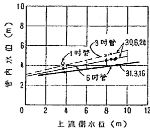
図-33 No. 2 沈下計の管内水位 (E.L. 606 m を 0 m とした)
