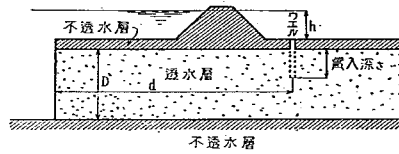
図-20 排水井系の説明図
