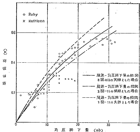
図-12 気圧降下量の潮位偏差との関係
