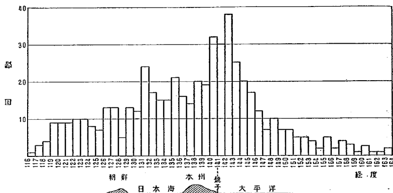
図-15 35° 44' の台風通過度数 (明治 24 ~ 昭和 29 63 年)
