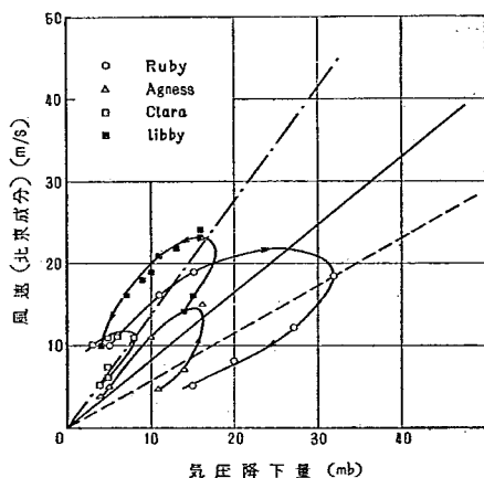
図-11 風速—気圧降下量の関係
