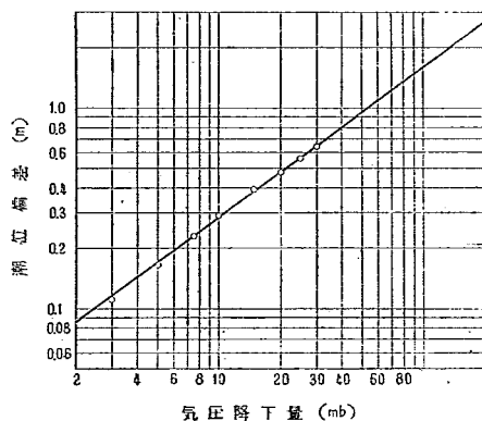
図-13 気圧降下量と潮位偏差との関係
