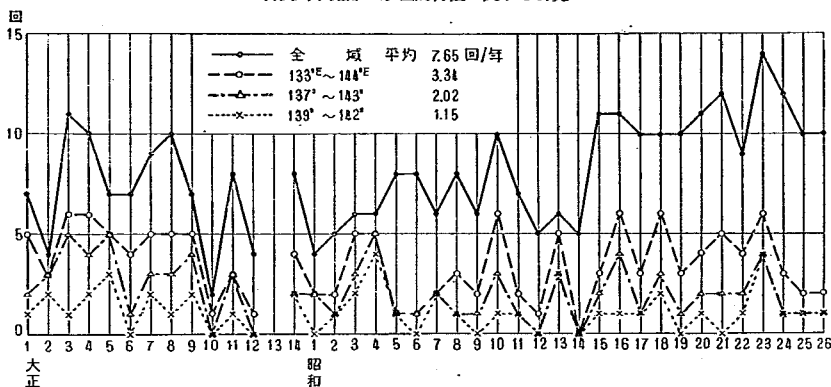
図-9 台風が N35° を通過した回数
