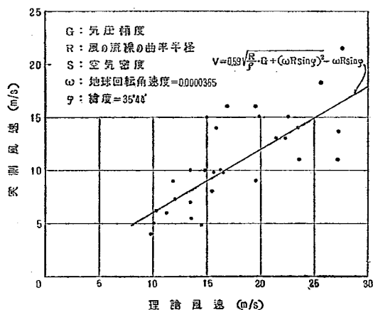
図-3 実測風速と理論風速との関係
