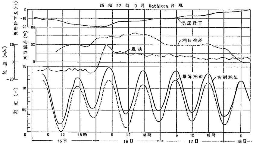
図-4・1 気圧降下量、風速、潮位偏差の変化状況（銚子）
