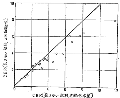
図-2 自然状態と吸水した試料の CBR の比較 (滝沢村附近)
