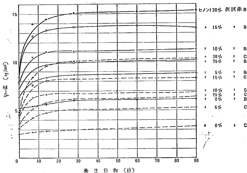
図-9. 一軸圧縮強度と養生日数との関係
