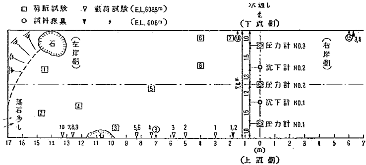
図—15 計器の据付と現場実験の位置砂川第4堰堤基礎平面)
