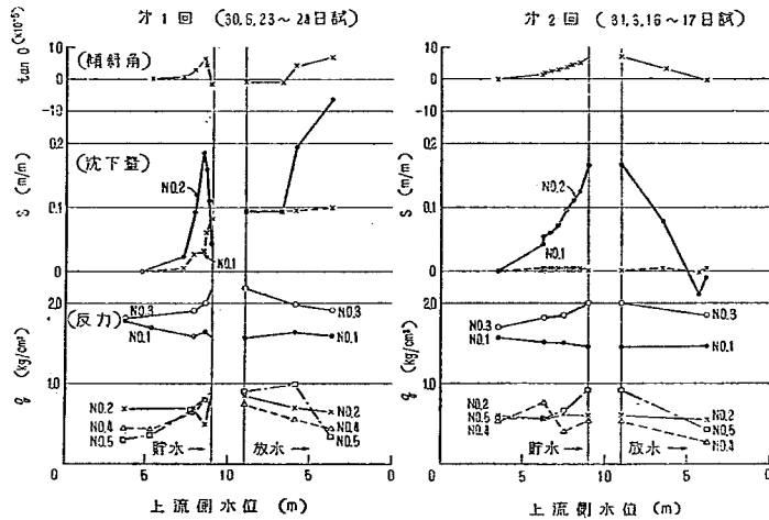
図-32 湛水試験中における測定値
