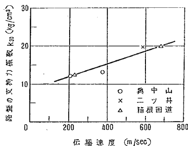
図-23 弾性波の伝播速度と路盤支持力係数の関係
