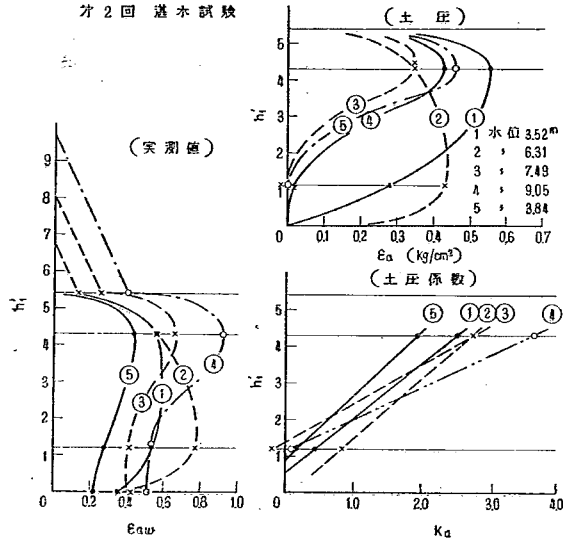
図一39 第2回湛水試験
