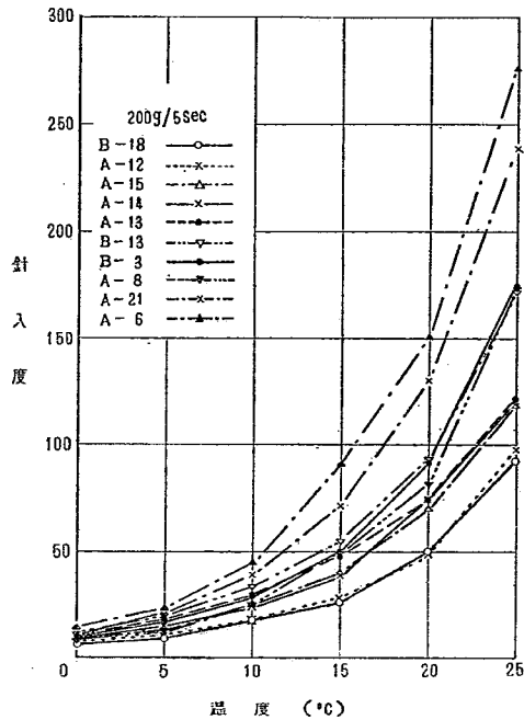
図一2. 針入度の温度依存性
