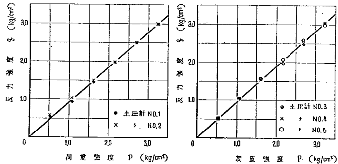
図-10 各土圧計の荷重強度-反力強度関係
