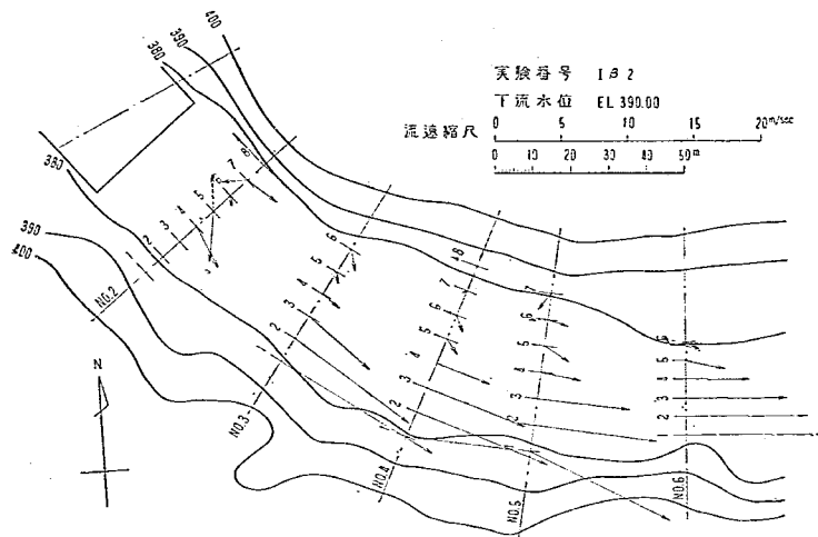
図—11 下流断面流速比較図
