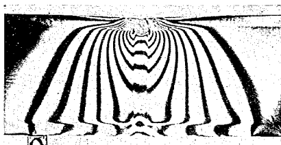
フ ラ ン ズ 無 t_l = 3.9 \phi = 25^\circ 10'
