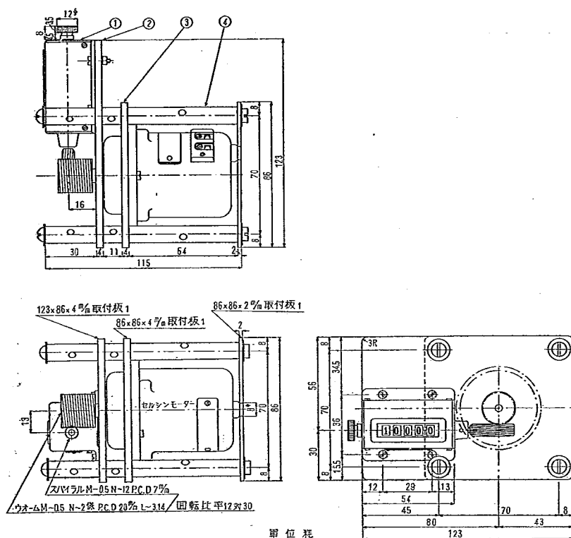
図-3. 水面追随器受信側
