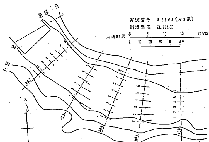
図-23 下流断面流速比較図
