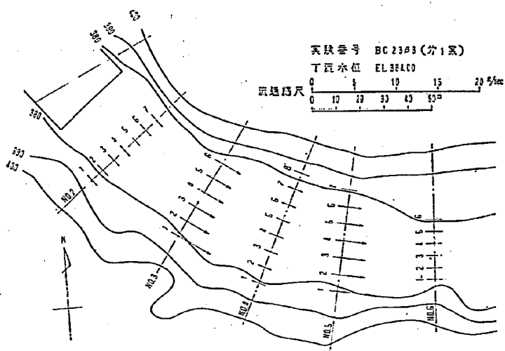
図-22 下流断面流速比較図
