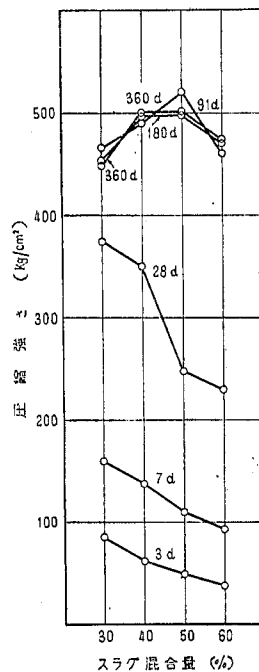
図-10. スラグ混含量と圧縮強さ (A社)
