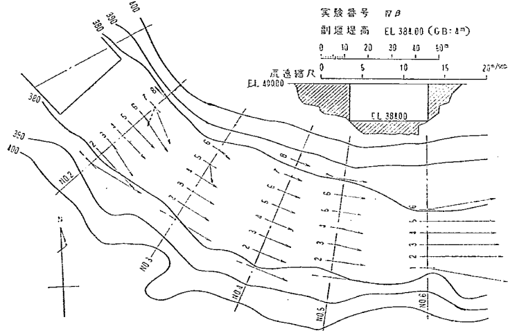
図-20 下流断面流速比較図
