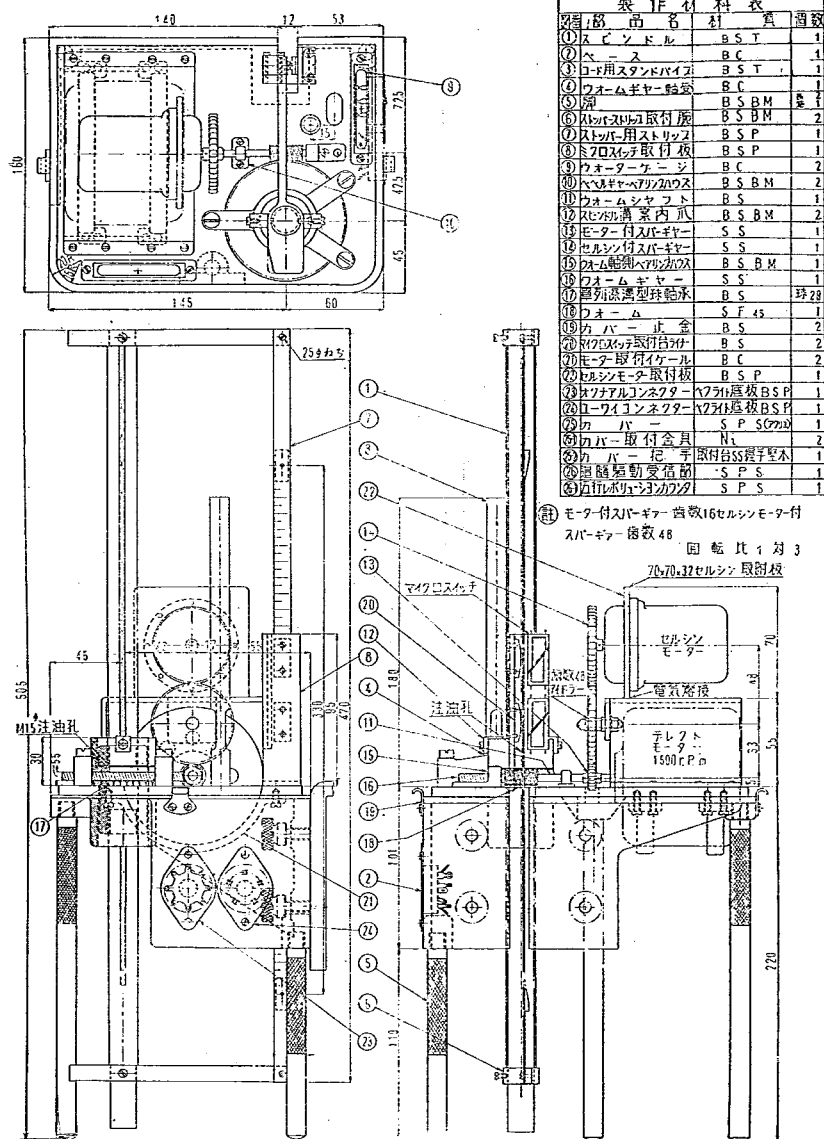
圖一2 水面追隨器発信側
