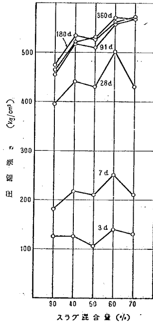
図-12. スラグ混合量と圧縮強さ (B社)
