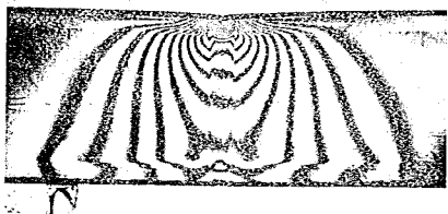
フ ラ ン ズ 無 t_l = 3.9 \phi = 25^\circ 10'
