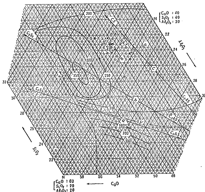
図-1. \text{CaO}-\text{Al}_2\text{O}_3-\text{SiO}_2 三成分系図
