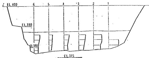
測線 No. 5 実験番号 A 22 \alpha 3 (第3案)
