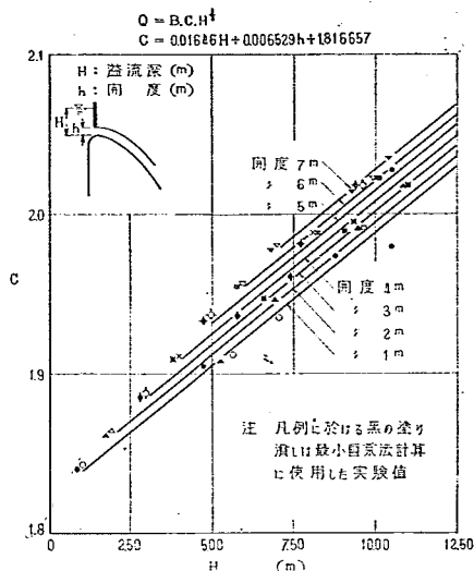
H—C 図—78 自由越流と半開操作組合
