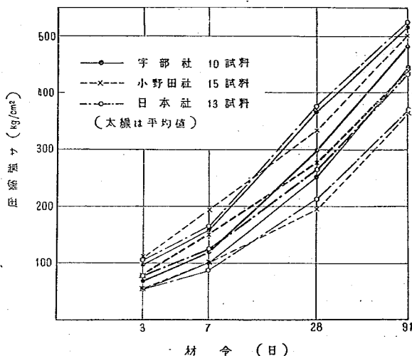
図-1 材令 91\text{ 日} までの各社セメントの圧縮強サ上限、下限及び平均値
