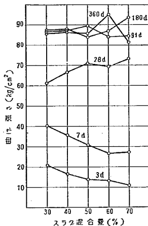
図-4. スラグ混合量と曲げ強さ (D社)
