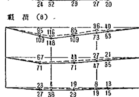
図-13 主桁応力度
