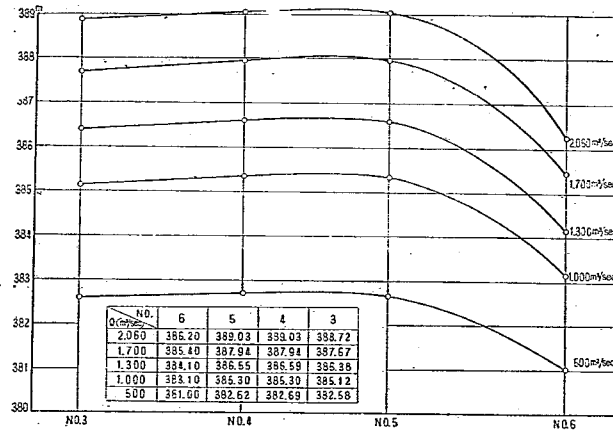
図-3 改良案（4門案）の自然下流水位縦断面図
