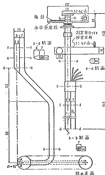
圖一-8 五管式球形壓力計
