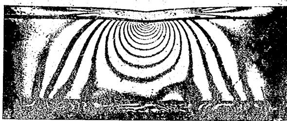
フ ラ ン ジ 附 t_0 = 3.9 \text{ mm}
