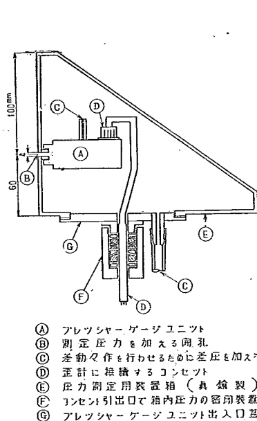
図一7 変動圧力測定説明図
