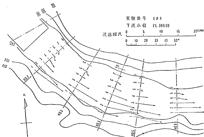
図-10 下流断面流速比較図
