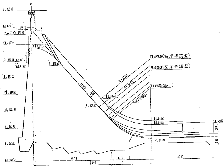
図-1 原案ダム側面図
