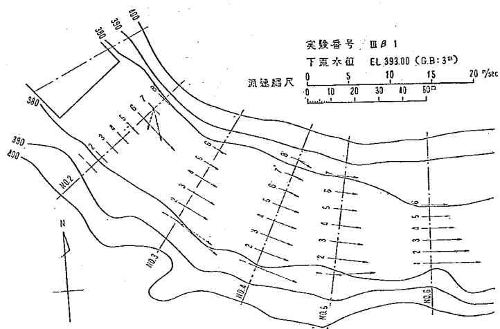
図—16 下流断面流速比較図
