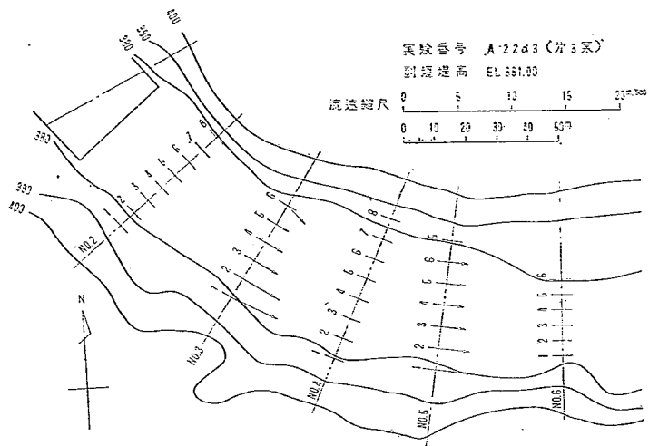
図—24 下流断面流速比較図
