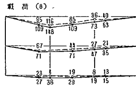
図-13 主桁応力度
