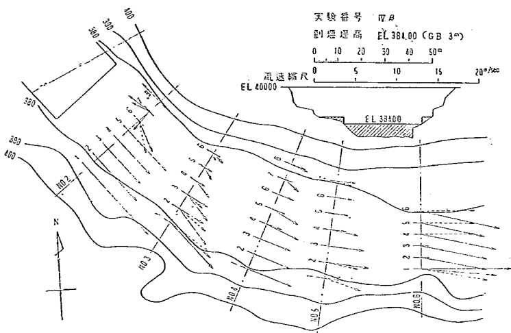
圖—18 下流断面流速比較図
