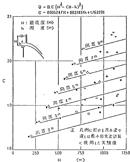
図-60 3門等高半開
