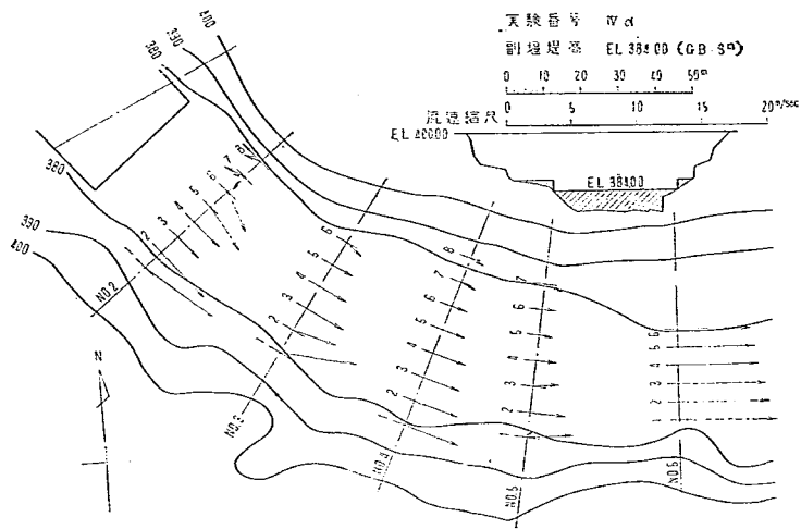
図-19 下流断面流速比較図
