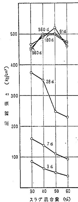
図-10. スラグ混含量と圧縮強さ (A社)
