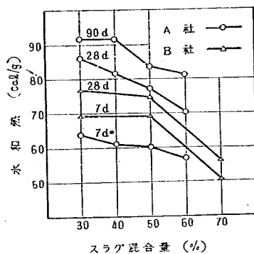
図-15. スラグ混合量と水和熱 (A, B社)
