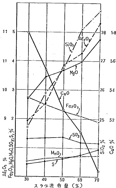
図-2 スラグ混合量と高炉セメント化学成分
