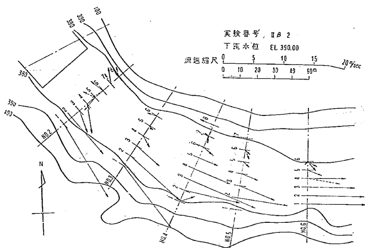
圖—13 下流断面流速比較図
