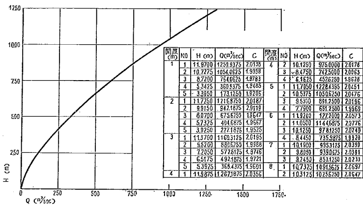
H—Q 図—73 自由越流と半開操作組合
