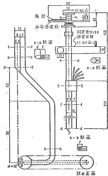
図一8 五管式球形圧力計
