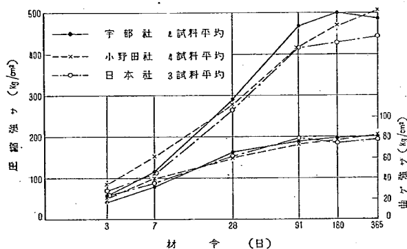
図-2 材令1年までの各社別曲ゲ、圧縮強サ平均値
