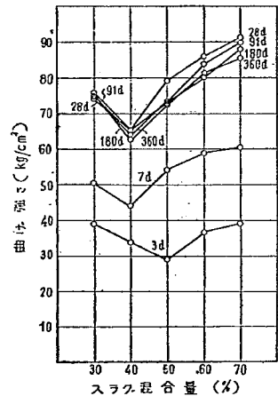
図-6. スラグ混合量と曲げ強さ (B社)
