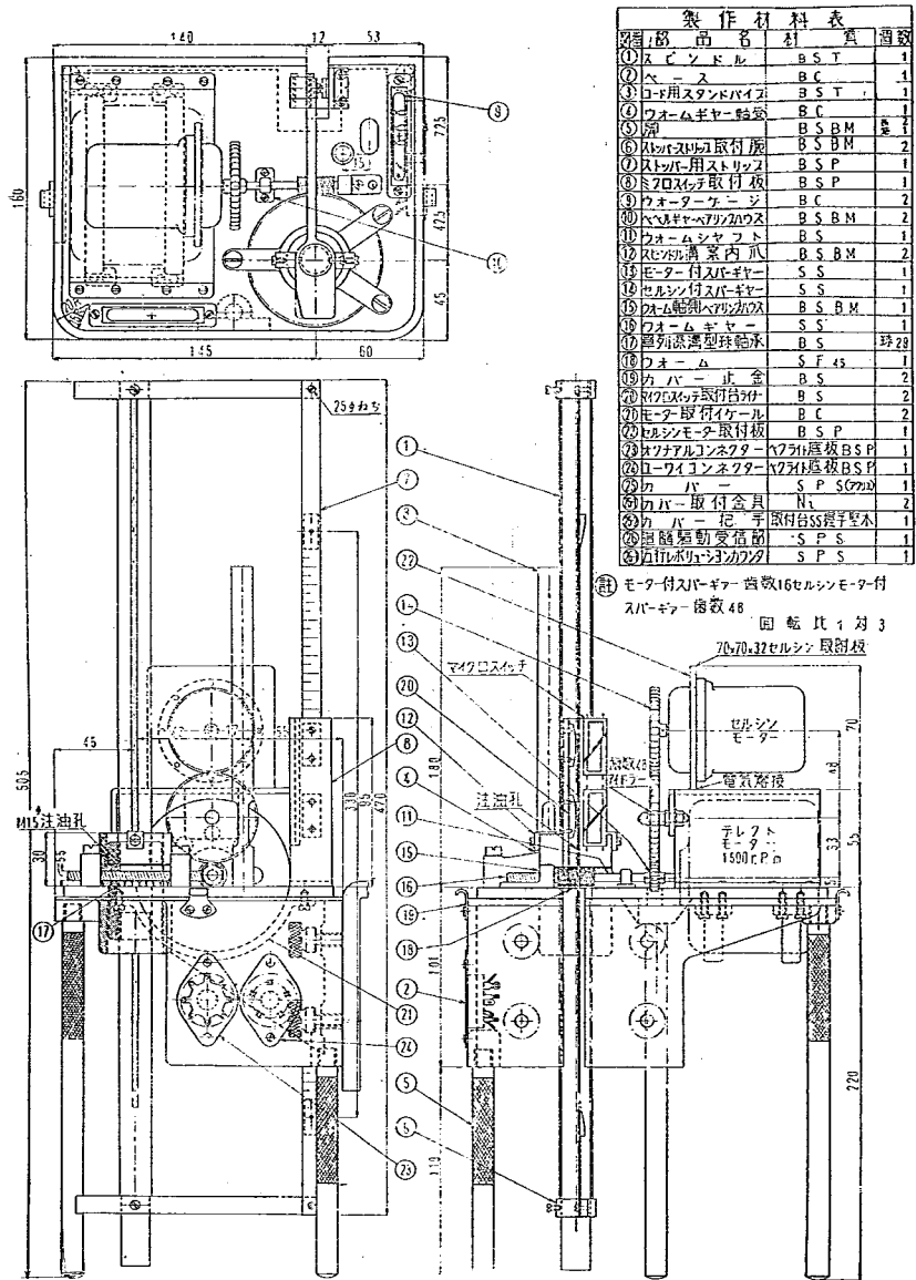
図-2 水面追隨器発信側
