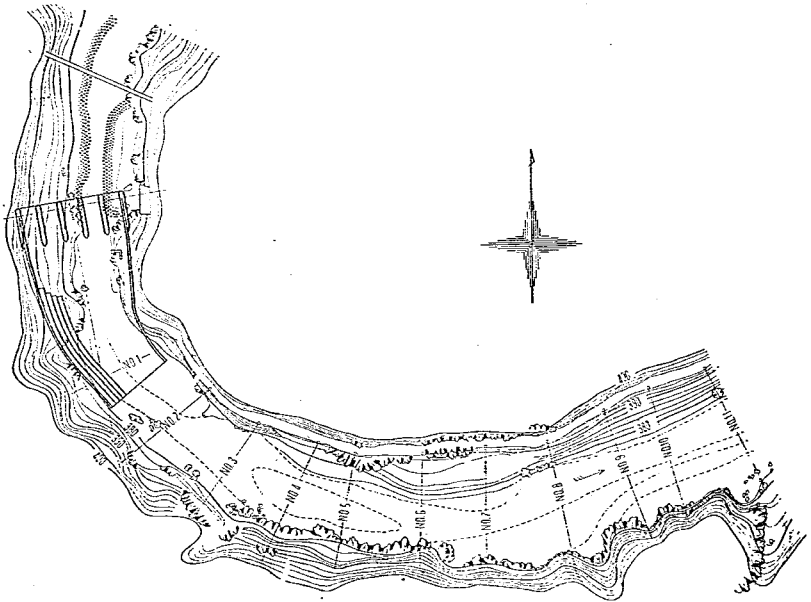
図-2 原案ダム下流平面図
