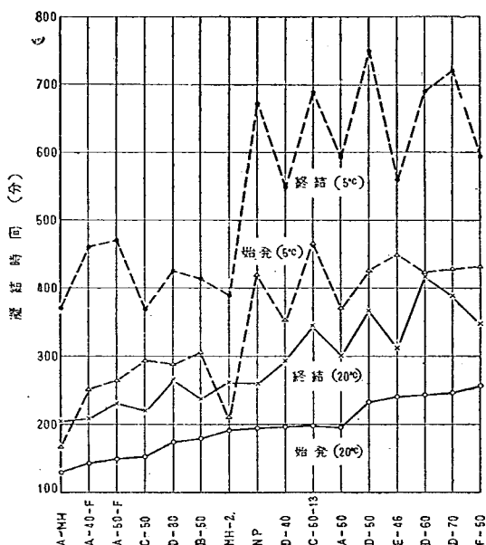
図—17. 凝結時間と温度との関係
