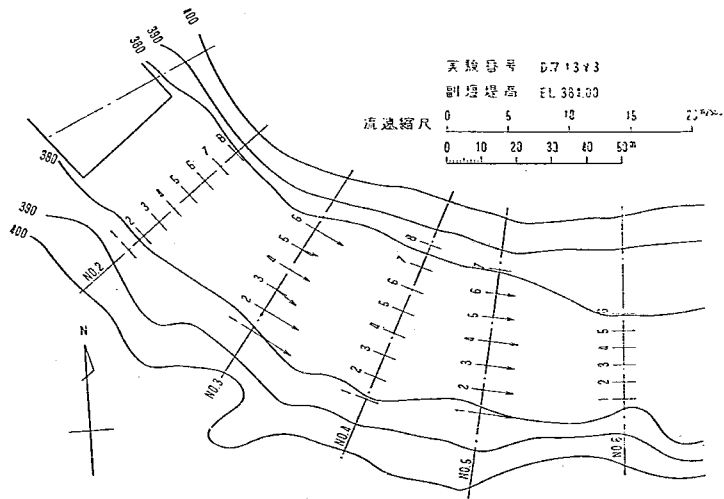
図-35 下流断面流速比較図
