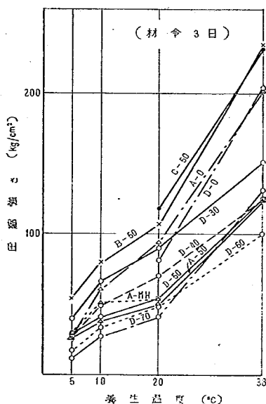
図—18. 養生温度と圧縮強さ (材令 3 日)
