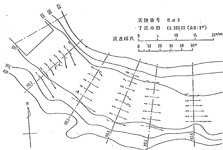
圖—17 下流断面流速比較図
