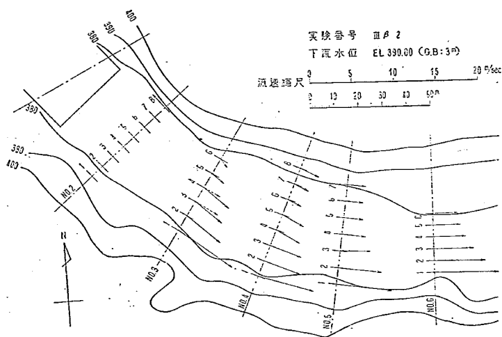
図—15 下流断面流速比較図
