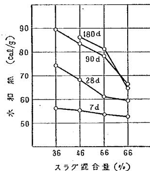
図-16. スラグ混合量と水和熱 (E社)
