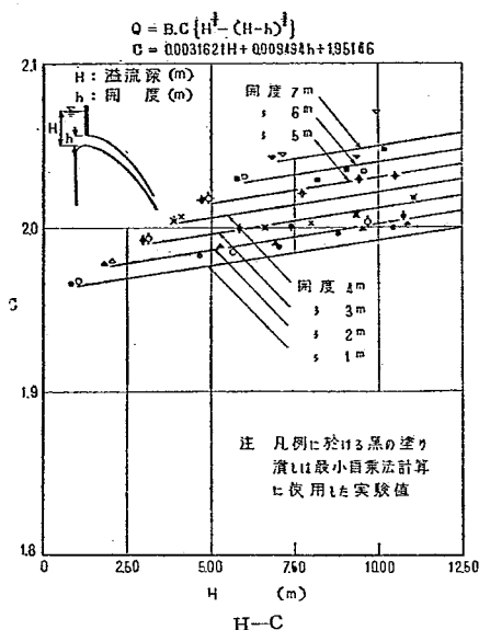
図—76 自由越流と半開操作組合
