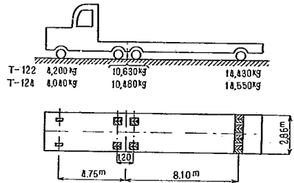
図-1 試験荷重車
