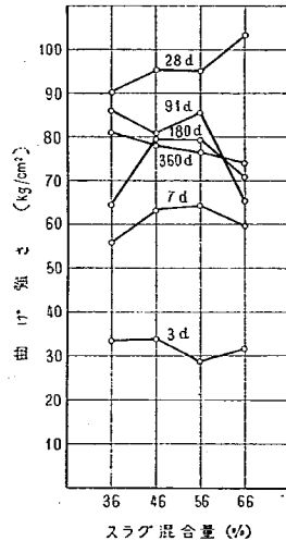
図-7. スラグ混合量と曲げ強さ (C社)
