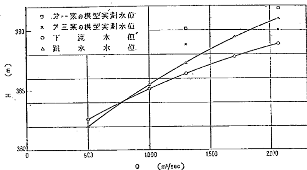
図-4 下流水位流量曲線図
