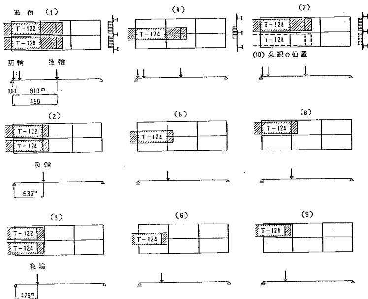
図-6 載 荷 状 態
