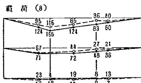
図-12 主桁応力度 (kg/cm 2 )
