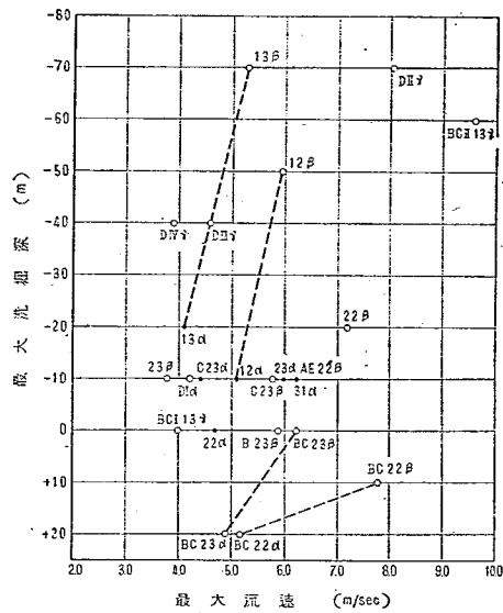
図—28 最大洗掘深—最大流速比較図
