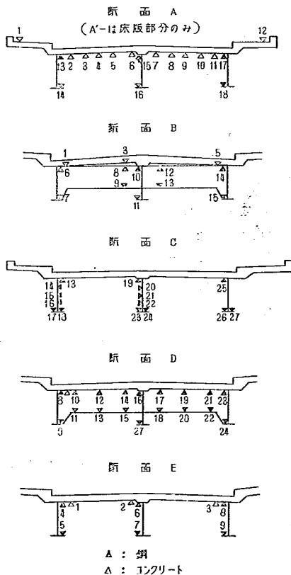
図-3 ひずみ、測定位置
