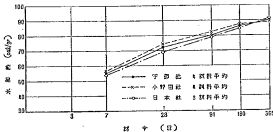
図-3 材令 1 年までの各社別水和熱平均値
