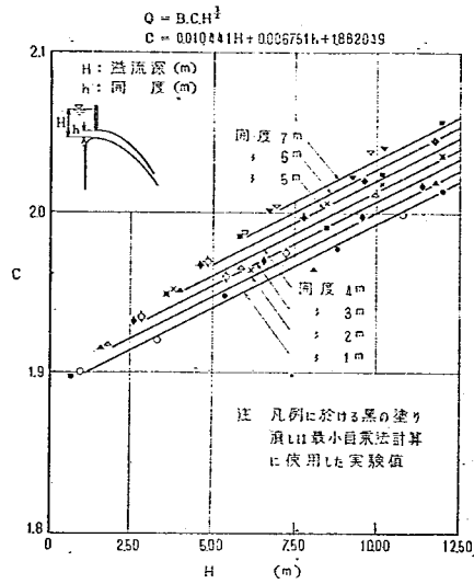
図—74 自由越流と半開操作組合
