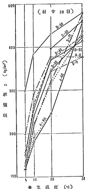
図—20. 養生温度と圧縮強度（材令 28 日）
