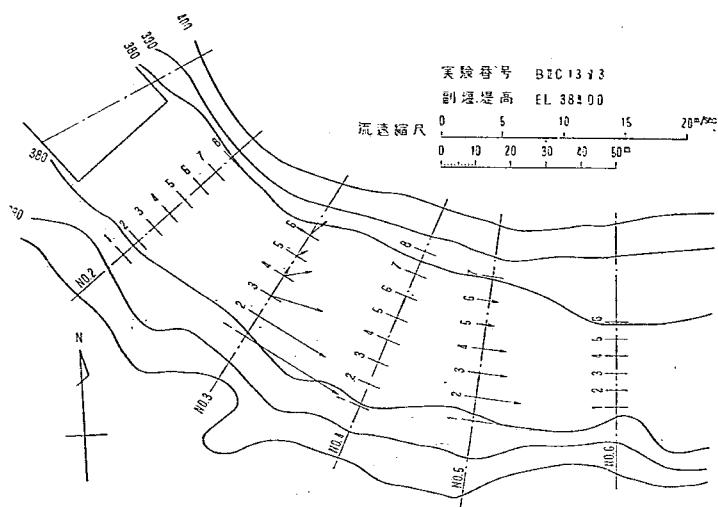
図—37 下流断面流速比較図
