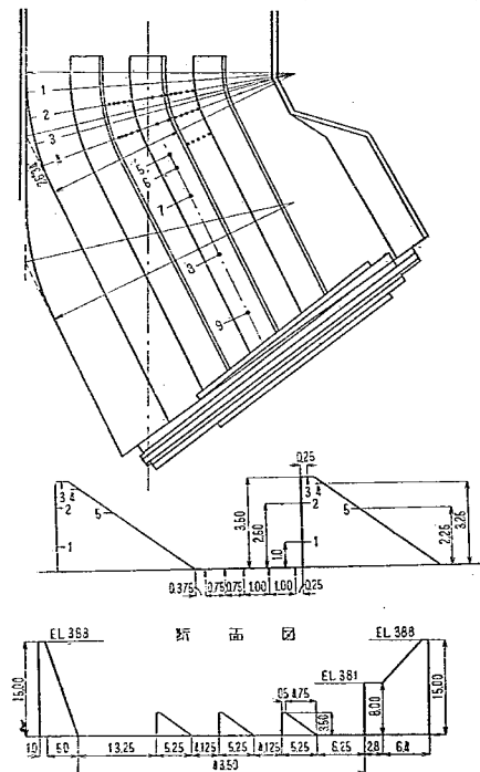
図-41 ピエゾメーター位置図
