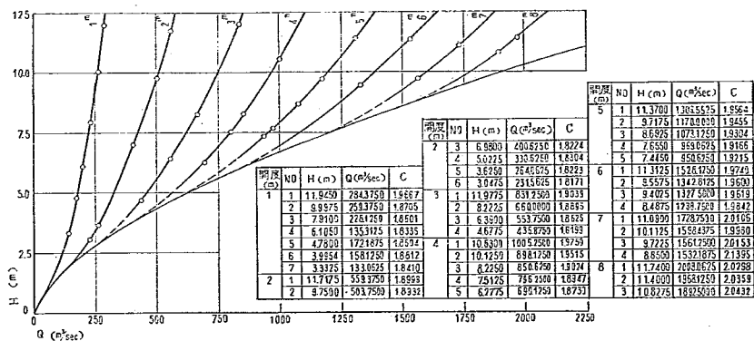
図—57 全門等高半開
