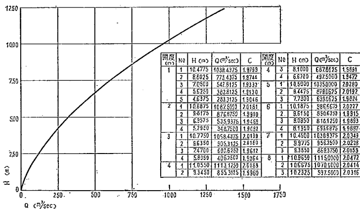
H—Q 図—77 自由越流と半開操作組合
