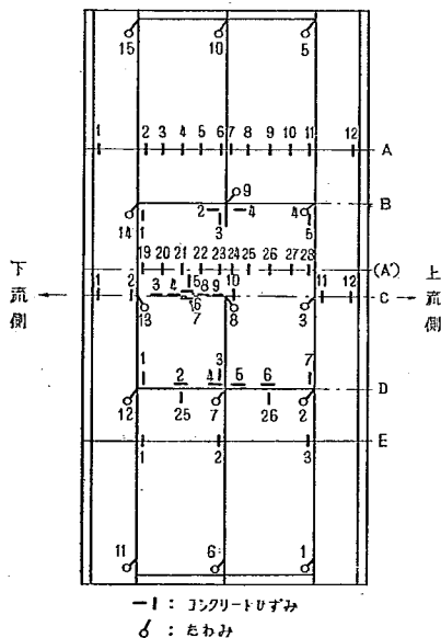
図-2 たわみ、コンクリートのひずみ、測定位置
