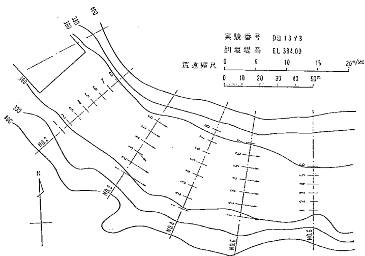
圖—34 下流断面流速比較図
