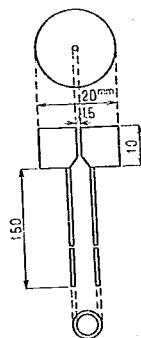
図-6 ピエゾメーター断面図
