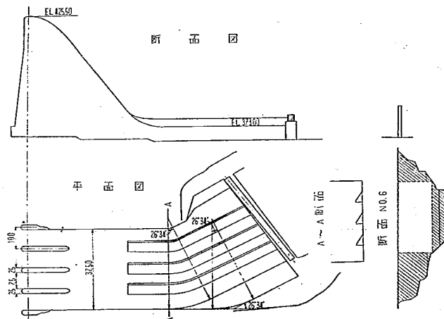
図-9 橋脚間隔導流壁 G.B 副ダム説明図
