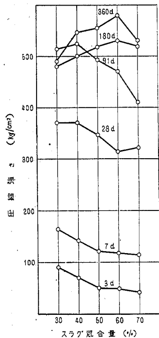
図-9. スラグ混含量と圧縮強さ (社D)
