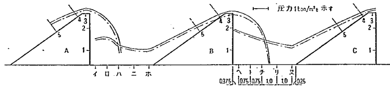
図—42 BC 22 β 3 Guide Baffle 断面圧力分布図
