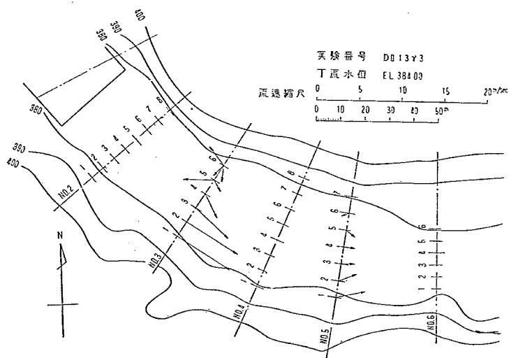
圖—33 下流断面流速比較図
