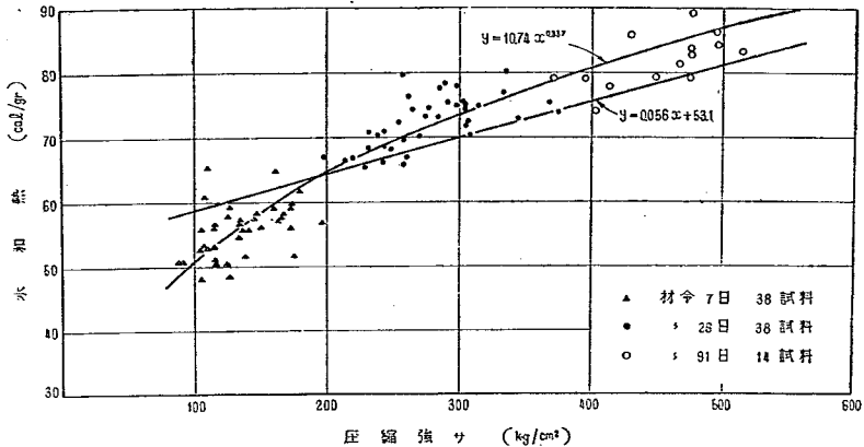
図-5 材令 7 日—91 日間の圧縮強サと水和熱の関係
