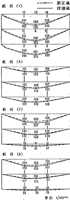
図-10 たわみ (単位 1/100 mm)
