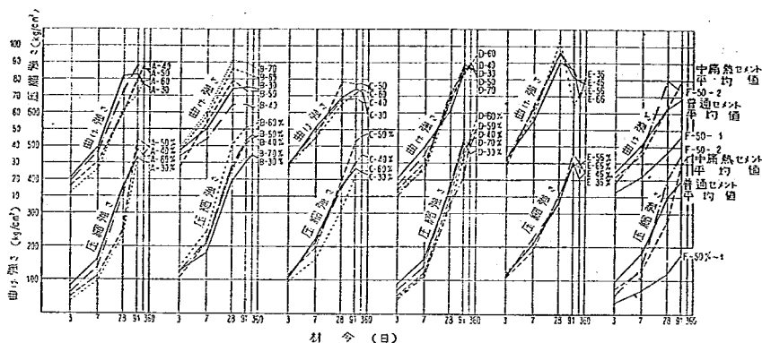
図-3 試製高炉セメント圧縮及び曲げ強さ
