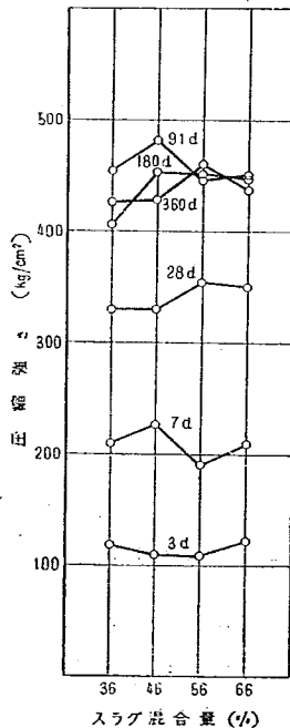
図-13. スラグ混合量と圧縮強さ (E社)
