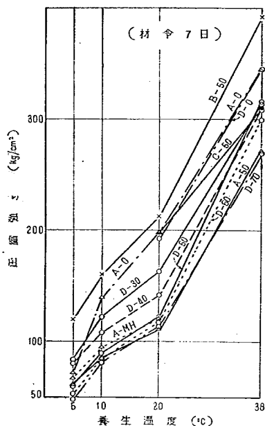
図—19. 養生温度と圧縮強さ (材令 7 日)
