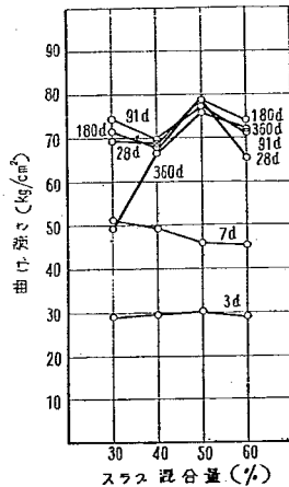
図-7. スラグ混合量と曲げ強さ (C社)
