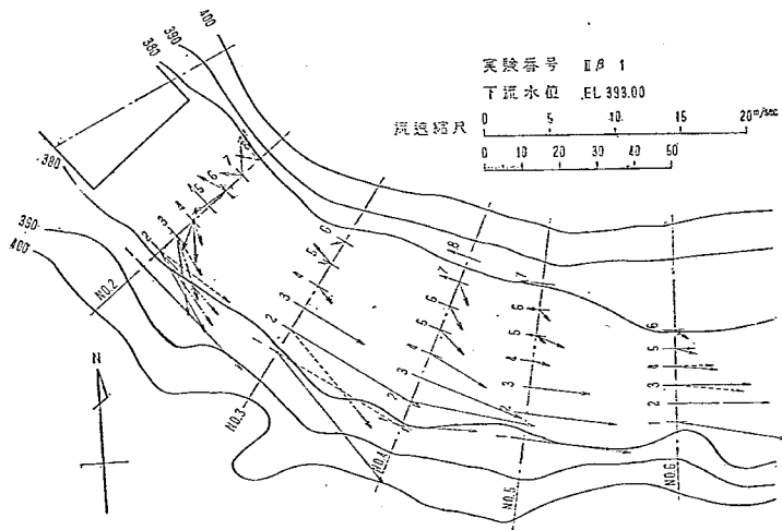
図—12 下流断面流速比較図
