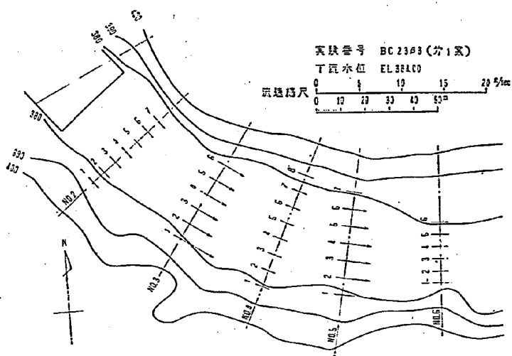
图—22 下流断面流速比較図
