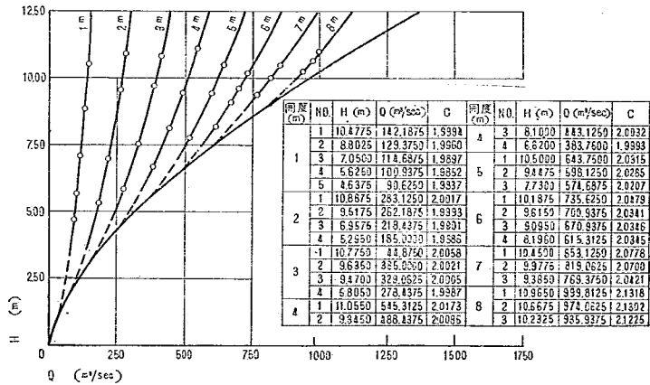
図—75 自由越流と半開操作組合
