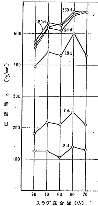
図-12. スラグ混合量と圧縮強さ (B社)
