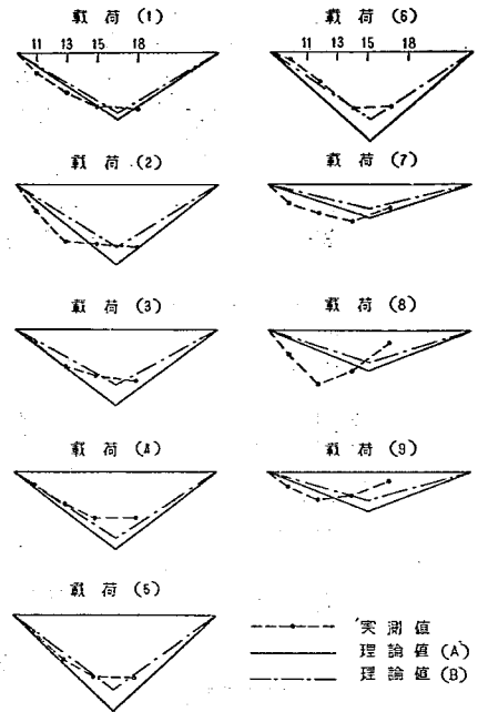
図—14 横桁応力度
