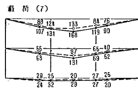
図-12 主桁応力度 (kg/cm 2 )
