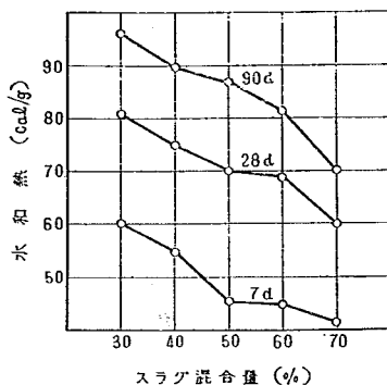
図-14. スラグ混合量と水和熱 (D社)
