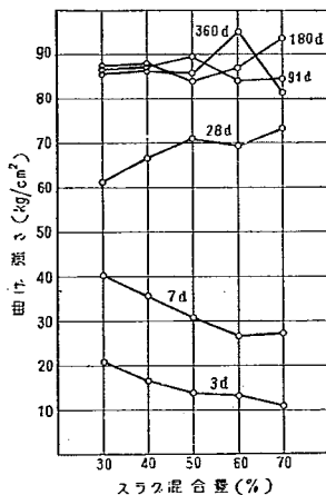
図-4. スラグ混合量と曲げ強さ (D社)
