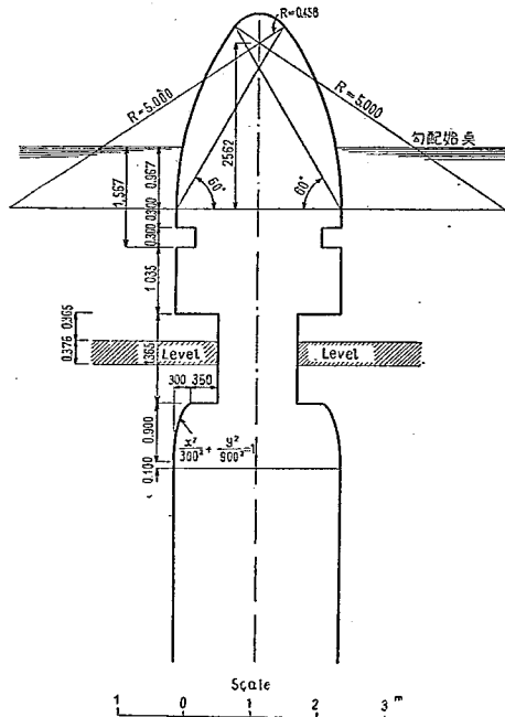
図—49 橋脚詳細図
