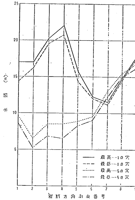
図—43 縦断方向圧力分布図
