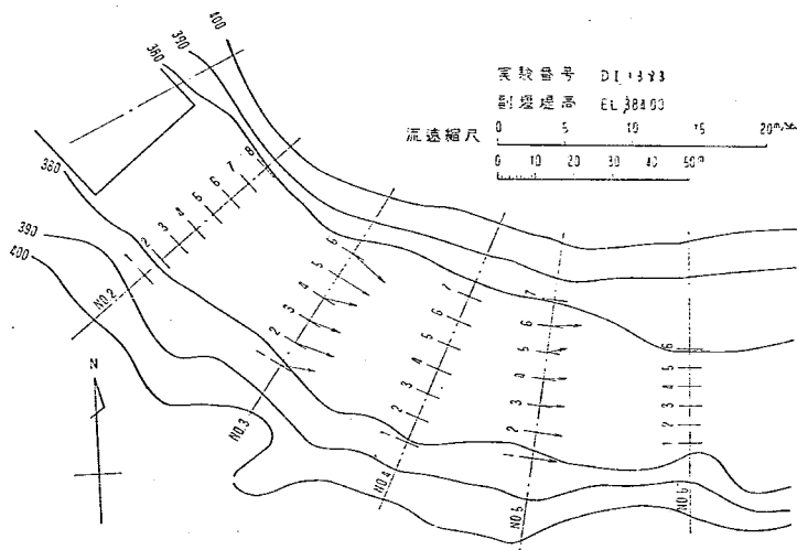
図—32 下流断面流速比較図
