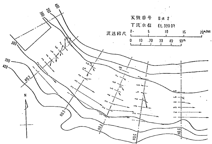
圖—14 下流断面流速比較図
