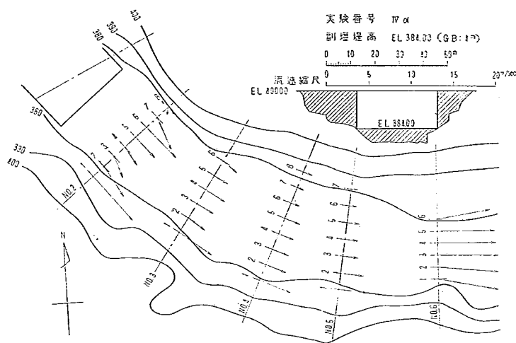
図-21 下流断面流速比較図
