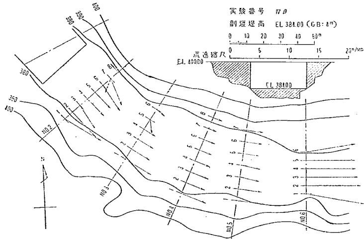
図-20 下流断面流速比較図
