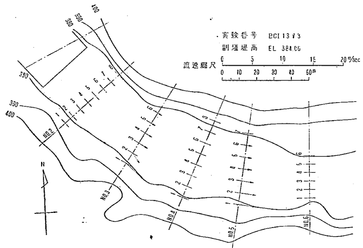
図-36 下流断面流速比較図
