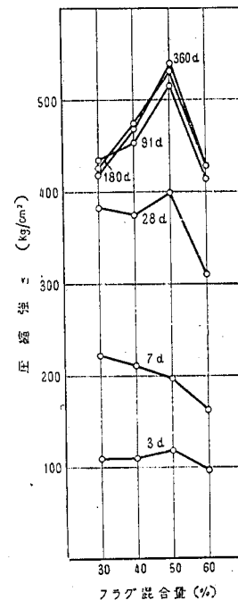
図-11. スラグ混含量と圧縮強さ (C社)
