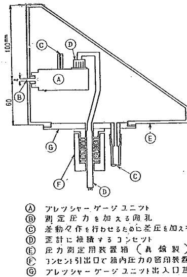
図一7 変動圧力測定説明図
