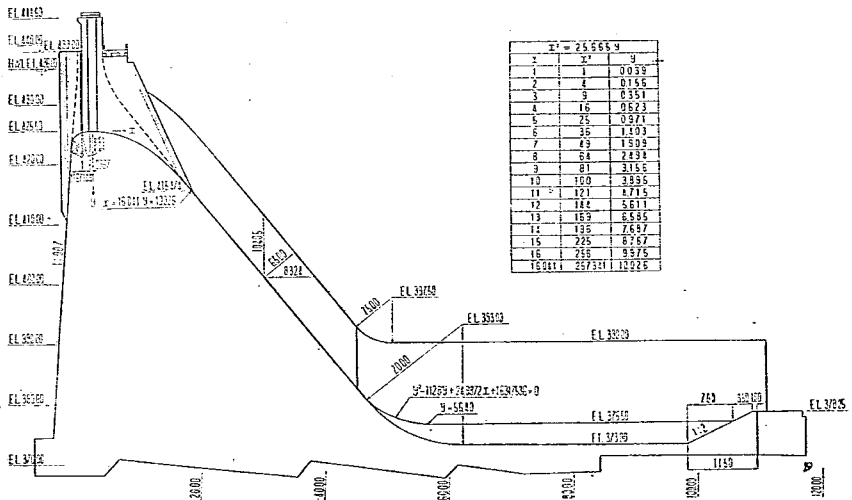
図—29 最終実施案側面図
