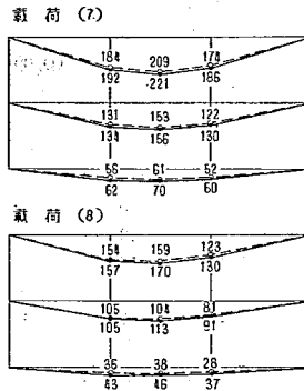
図-11 主桁たわみ
