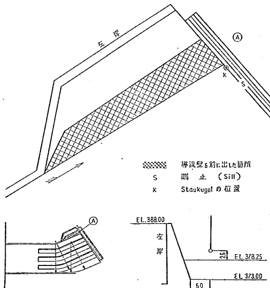
図-39 逆流測定位置図
