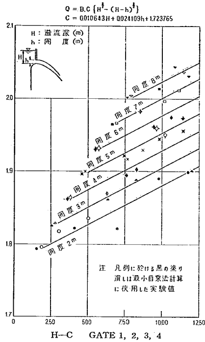
図-58 全門等高半開
