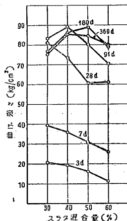
図-5. スラグ混合量と曲げ強さ (A社)
