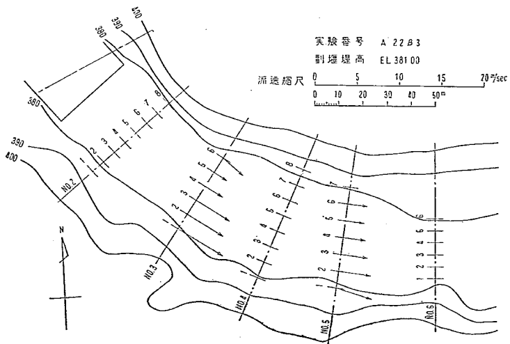
図—25 下流断面流速比較図
