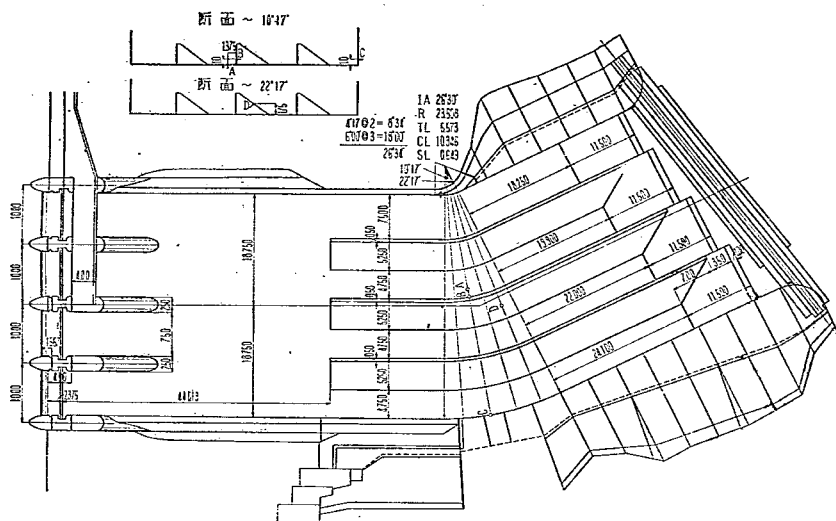
図-30 最終実施案平面図
