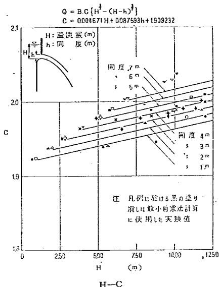
図—72 自由越流と半開操作組合
