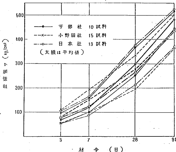
図-1 材令 91 日までの各社セメントの圧縮強サ上限、下限及び平均値
