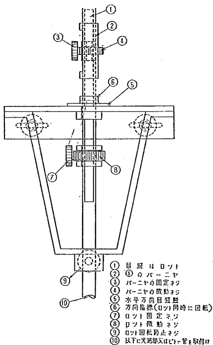
図-5 水面測定器説明図
