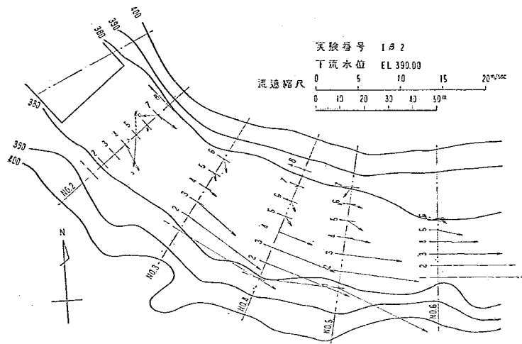
図—11 下流断面流速比較図
