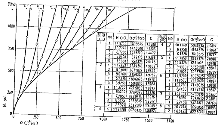
H-Q 図-71 自由越流と半開操作組合 ( 45 )
