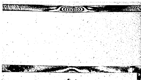
フランジ無 t_P = 2.9
