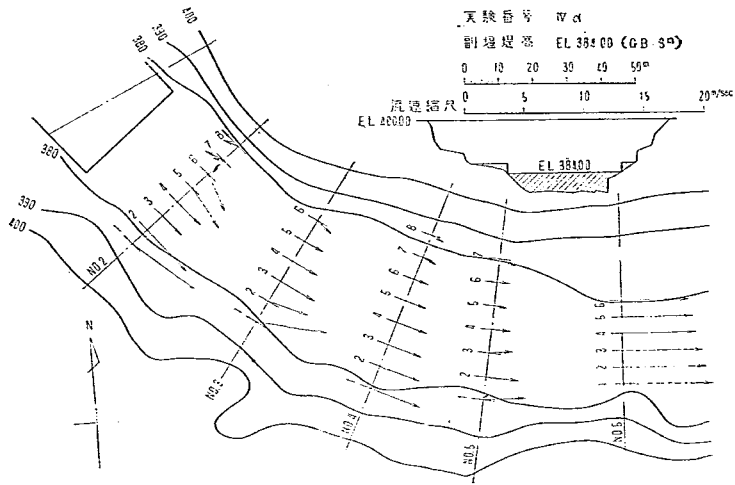
図-19 下流断面流速比較図
