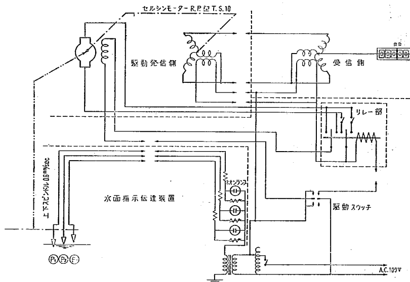
図-1. 水面追従器系統図
