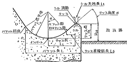
図一 一般的バケット形状説明図
