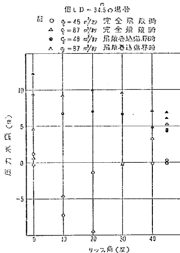
図-10 シル頂面圧力
