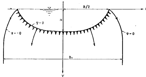
図-6 地下水位の深い場合の溝からの滲透
