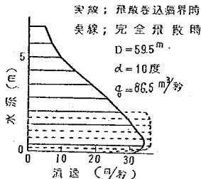
図—22 飛散時と飛散巻込臨界時とのリップ断面流速分布比較
