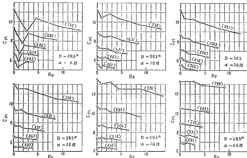
図-21 Re と飛散巻込臨界水深係数の関係
