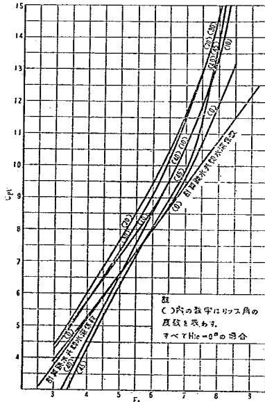
図-18 フルード数、飛散巻込臨界水深係数関係曲線
