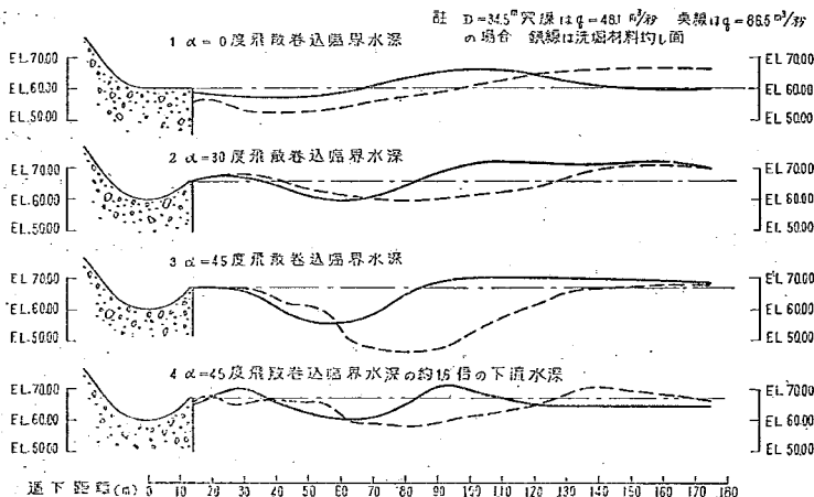
図-23 バケット型水叩における洗掘状態の例
