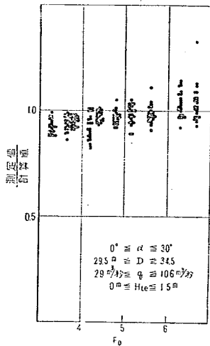
図一五 飛散巻込臨界水深計算値 測定値比較-2
