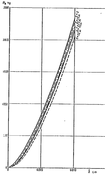
(1) 接触球数の変化、すなわち負荷分布の変化 図一5
