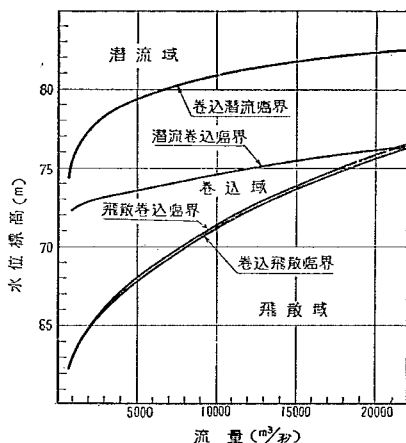
図-3 各種臨界水位の相互関係 (Bugs Island Dam の例)
