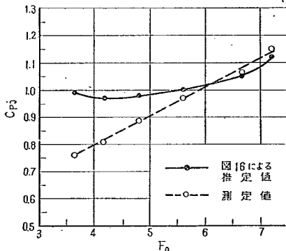
図-17 C_{pf} 推定値と測定値の比較
