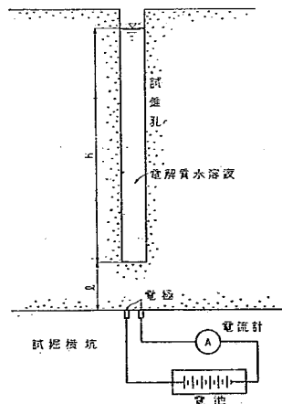
図一5 試錐孔による透水係数測定法
