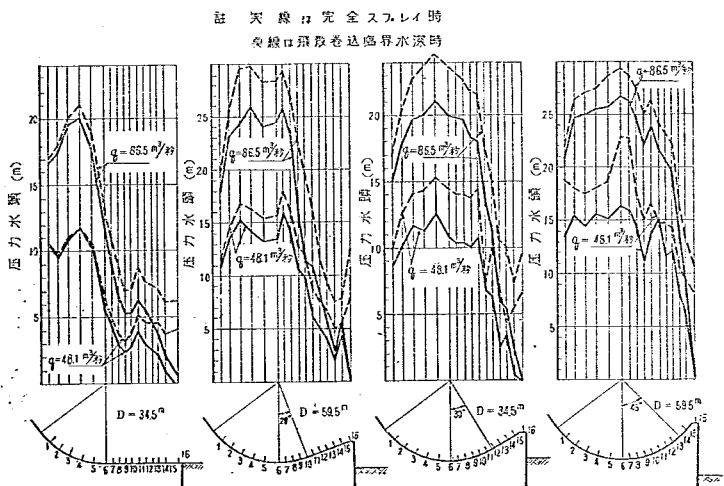
図-6 バケット面圧力分布実験例
