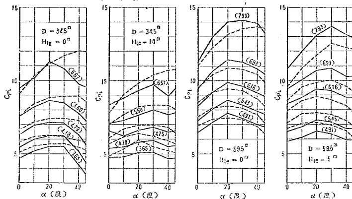
図-20 リップ角と飛散巻込臨界水深係数の関係
