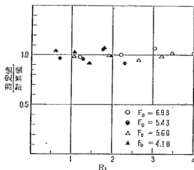
図-8 巻込直前時におけるバケツ面全 圧力水平成分計算値実験値比較
