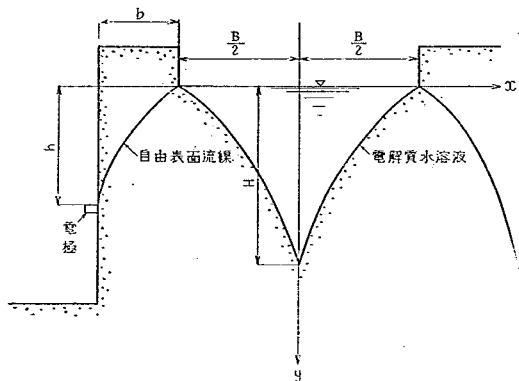
図一7 試験溝による透水係数測定法
