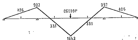
B 桁 曲 げ モーメント図
