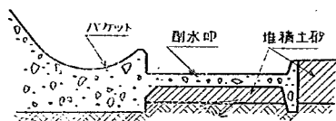
図—24 Buggs Island Dam のバケット縦断形状
