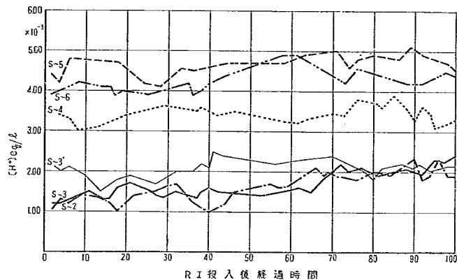
図-7 メチルオレンジ酸度の時間的变化
