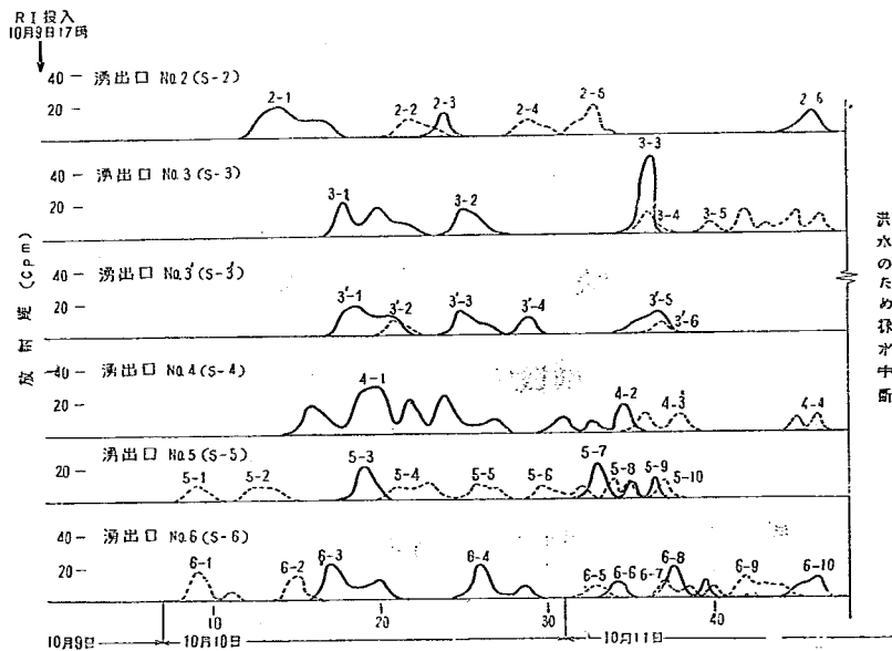
RI投入後の経過時間 図-10 第2回実験RI流出状況 (1956年10月9日~13日)
