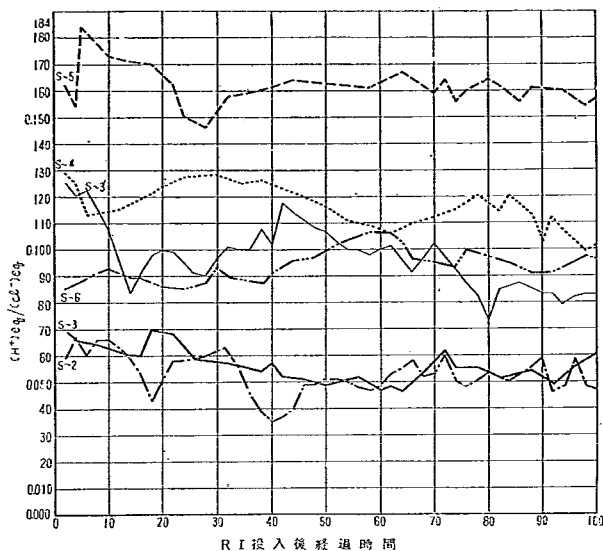
図-9 湧出水における塩素イオン対水素イオン濃度化
