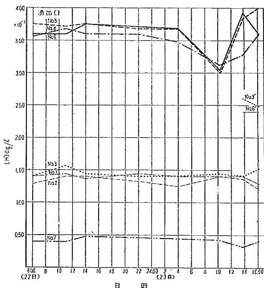
図—2 メチルオレンジ酸度の時間的変化
