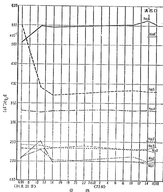
図-3 塩素イオン濃度の時間的变化
