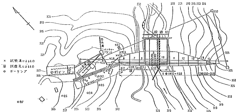
図一8 透水試験測定箇所及びボーリング箇所
