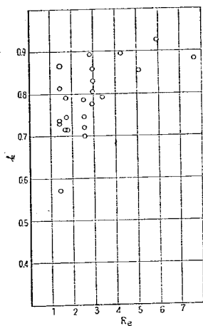
図-9 巻込直前時におけるシル垂直 面圧力水頭と下流水深との比較
