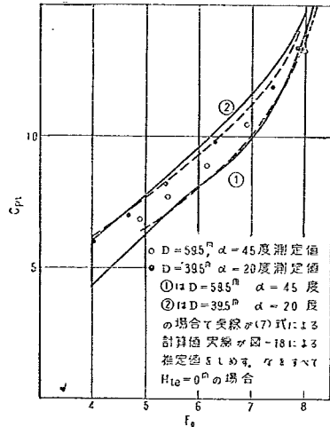
図-19 C_{pi} 推定値と測定値の比較
