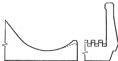
図—25 副水叩を有するバケットの縦断形状
