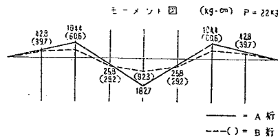
図-22 A, B 桁の荷重, モーメント図, 撓み図
