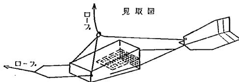
図-2 掃流砂採取器
