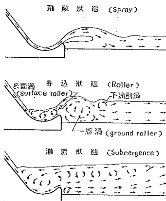
図二 飛散, 巻込, 潜流各流況説明図
