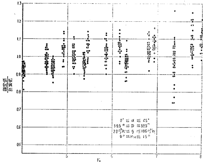
図一四 飛散巻込臨界水深計算値測定値比較
