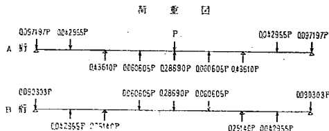
図-22 A, B 桁の荷重, モーメント図, 撓み図
