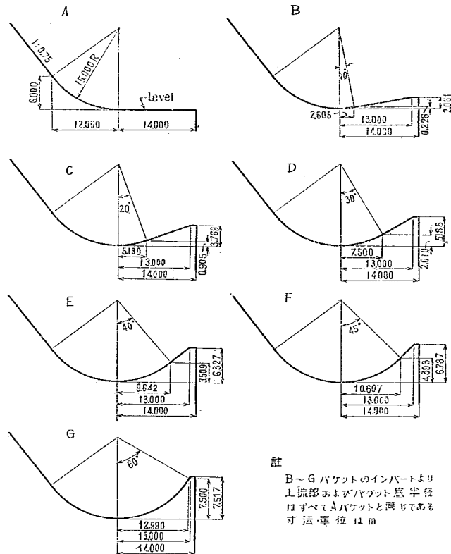
図-5 秋葉ダム水理模型実験で使用されたパケット模型縦断形状
