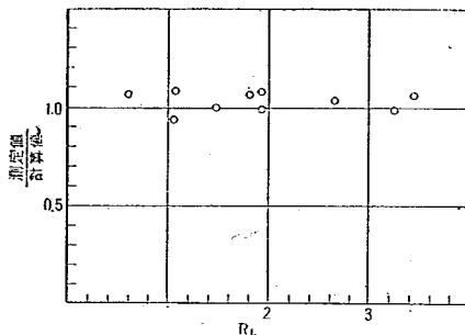
図-7 バケツ面全圧力水平成分計算値 実験値比較
