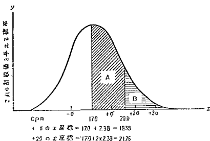
図-4 バックグラウンドの計数値分布曲線
