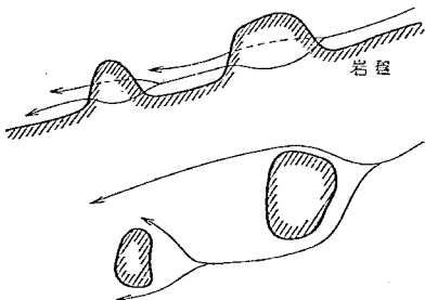
図-13 岩塊突起によるフィンガリング現象模型図
