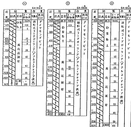
図-4-1 左岸地質柱状図
