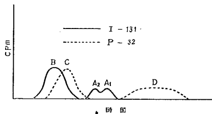
図—12 R I流出の推定図
