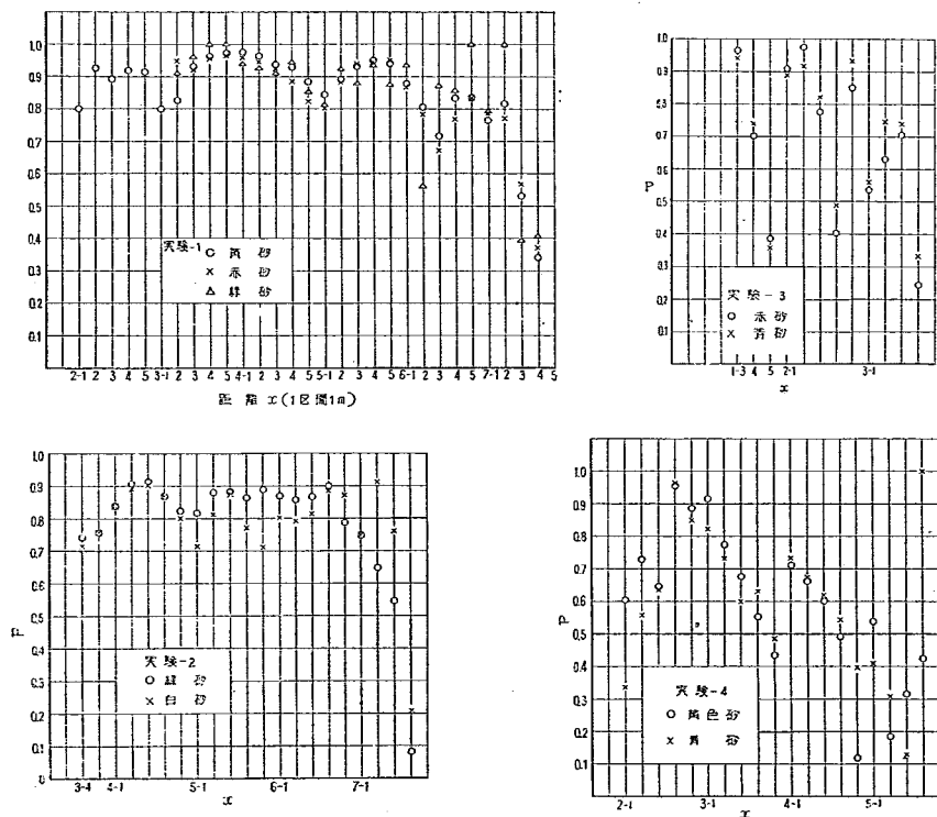
図-4 染色砂の移動確率
