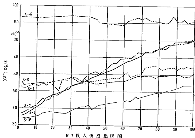
図-8 塩素イオン濃度の時間的变化
