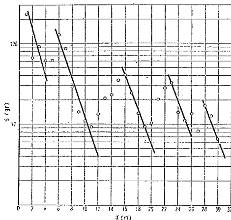
図-3 染色砂の分布の一例
