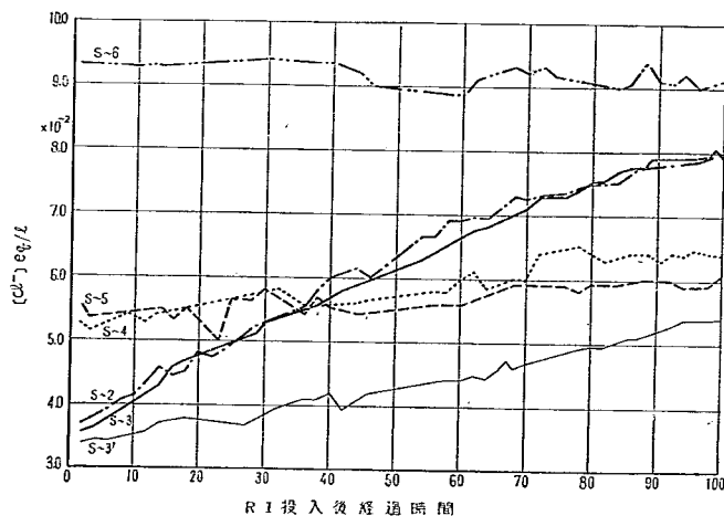
図-8 塩素イオン濃度の時間的变化
