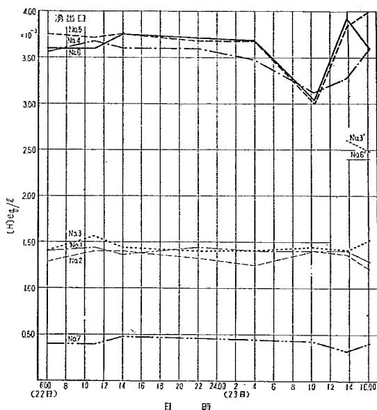
図—2 メチルオレンジ酸度の時間的变化
