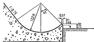
図-26 櫛型バケツトの形状
