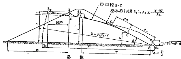
図-9 浸透線図
