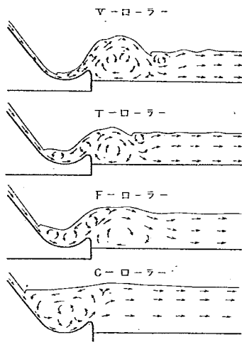
図-4 巻込流況の諸相説明図
