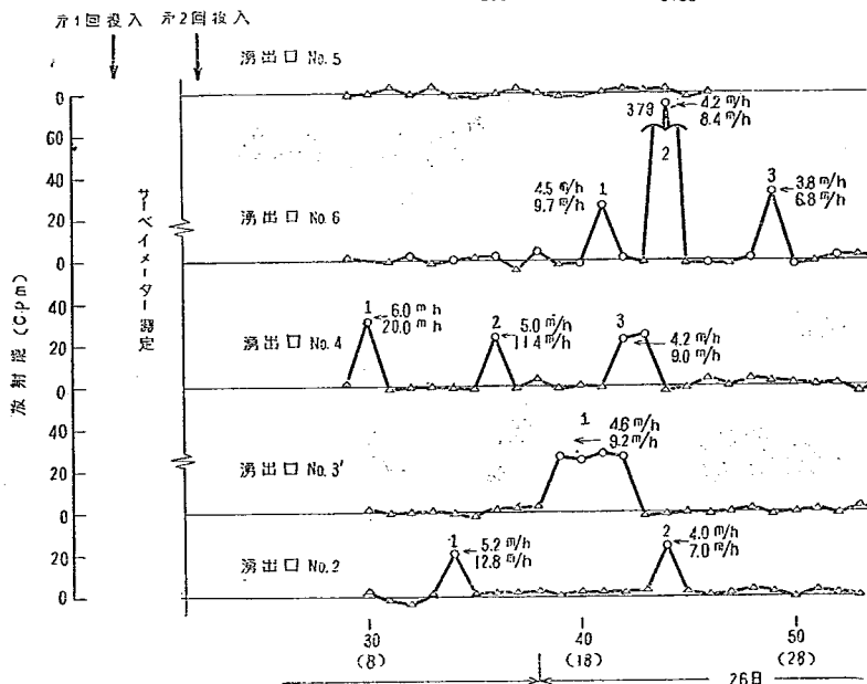
図—6 第1回実験R I流出状況 (1956年3月)
