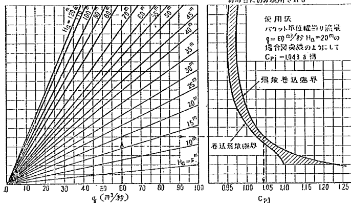
図-16 J. A. Tiffanyにより与えられた C_{pf} 計算図
