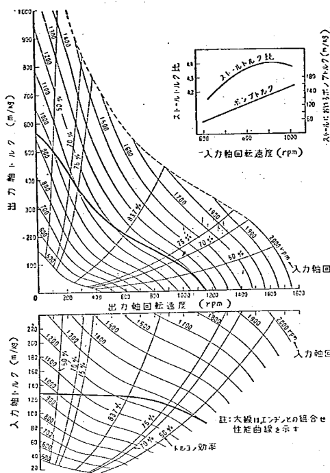
図-8 トルクコンバータ (138-M, 300) 性能曲線
