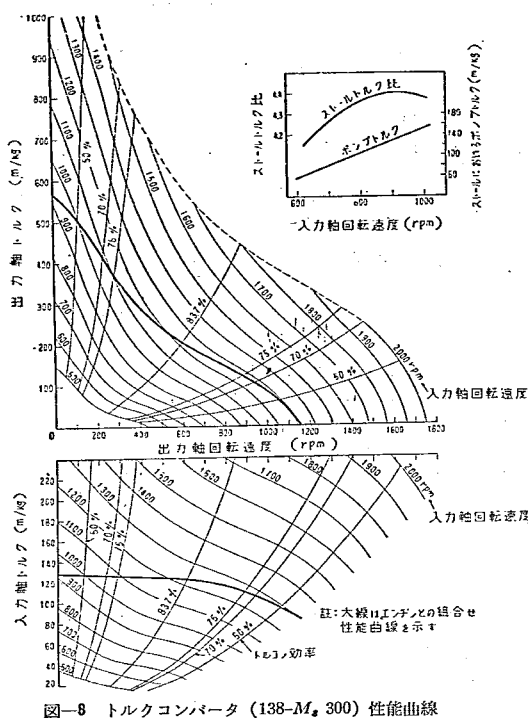
図-8 トルクコンバータ (138-M, 300) 性能曲線
