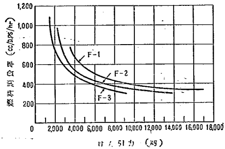
図-14 燃 焼 消 費 率
