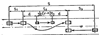
図-18 追越視距
