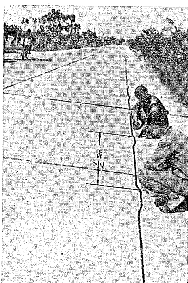
写真-3 1/2 sec 作動の走行軌跡 表-1 走行残跡装置のジェットの特性
