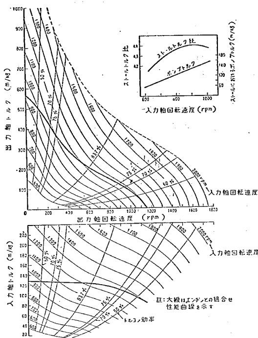
図-8 トルクコンバータ (138-M, 300) 性能曲線
