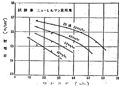
図-14 異なる初速度と増加加速度に対する加速度の関係
