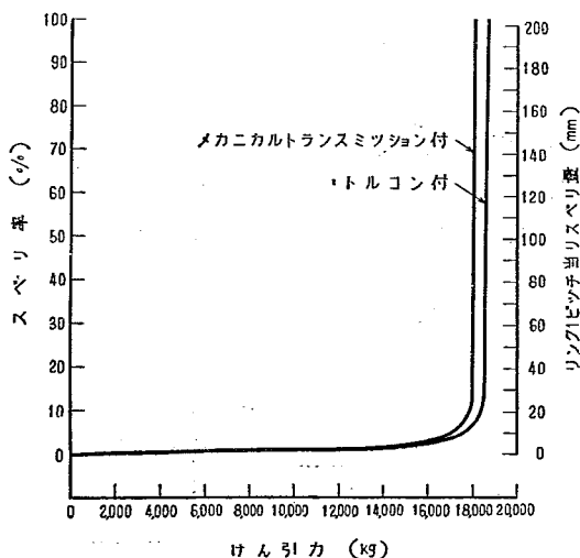
図-9 けん引力と滑り率
