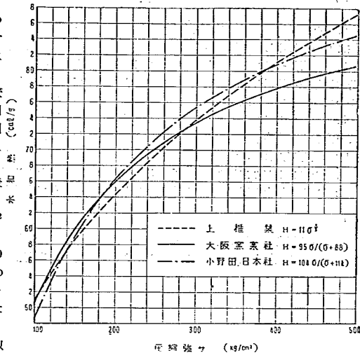
図-8 圧縮強さと水和熱の関係
