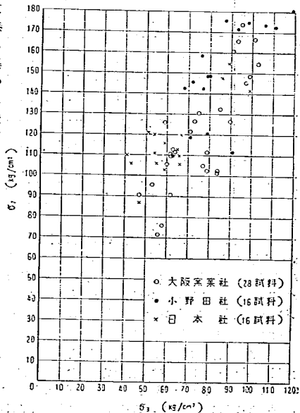
図-4 圧縮強サ ( \sigma_3 , \sigma_7 ) 間の関係
