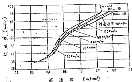
図-15 速度と減速度の関係
