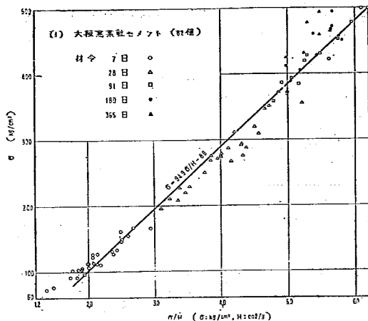
図-7 (1) \sigma - \sigma/H の関係
