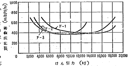
図-15 燃焼消費率 (トルコン付)
