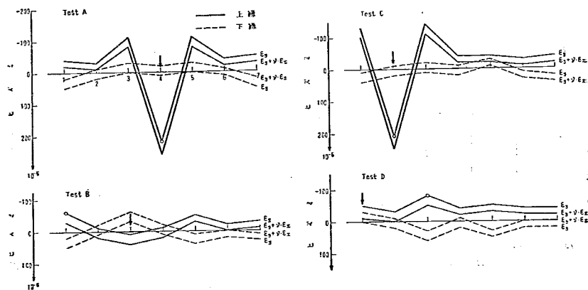
図-8 断面内における横方向ヒズミ ( \epsilon_y ) の分布
