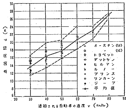
図-9 追越される自動車の速度と車頭間隔の関係
