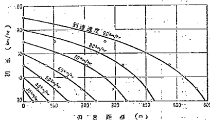
図-5 速度と加速距離
