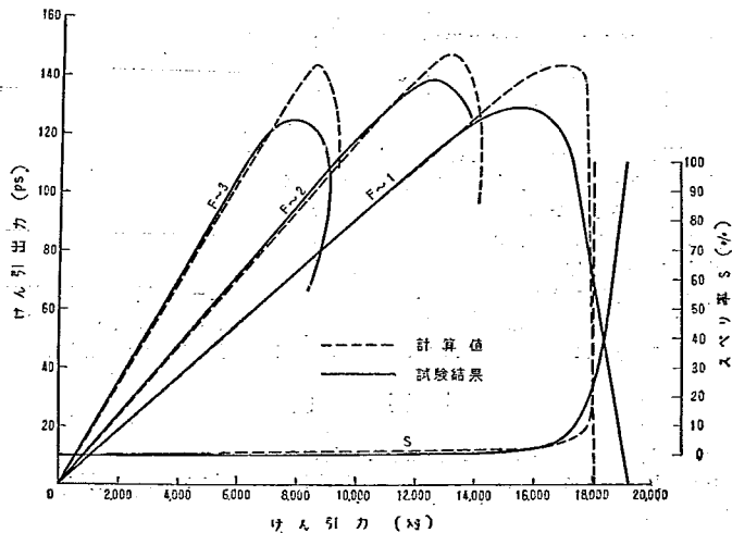
図-16 けん引出力の比較 (メカニカルトランスミッション付)
