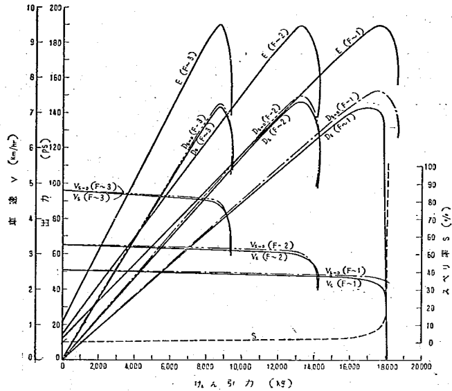
図-10 けん引特性図 (メカニカルトランスミッション付)
