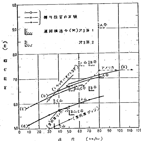
図-22 速度と追越所要車員の関係
