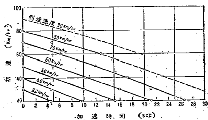
図-6 速度と加速時間
