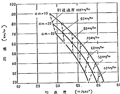
図—12 速度と加速度の関係
