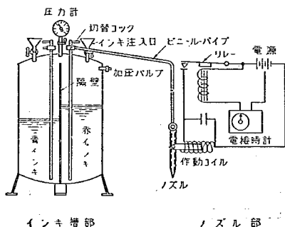
図-3 走行残跡装置
