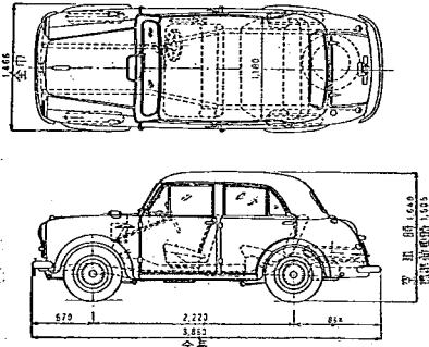
図-2.d ダツサン
