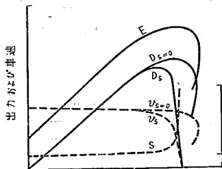
図-1 けん引特性図 (メカニカルトランスミッション付)
