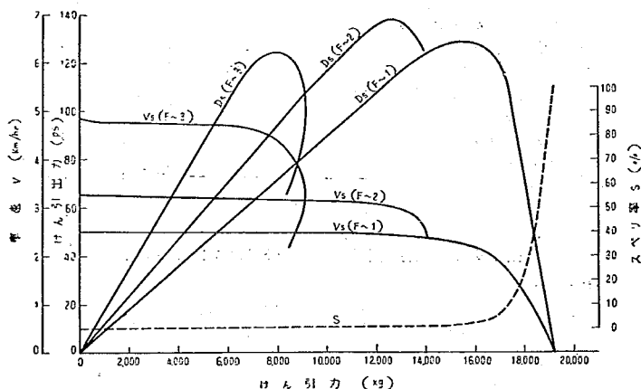
図-12 けん引試験特性図 (メカニカルトランスミッション付)
