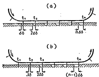
図—5 履板列の接地状況
