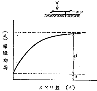
図-3 履板の粘着特性図
