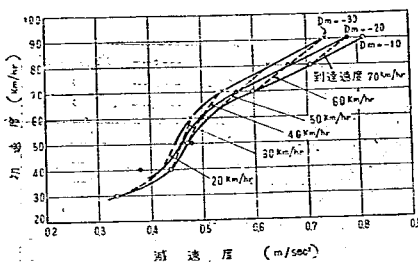
図-15 速度と減速度の関係
