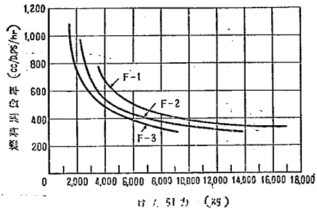
図-14 燃焼消費率 (メカニカルトランスミッション付)
