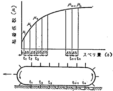
図-4 車輻の粘着特性図
