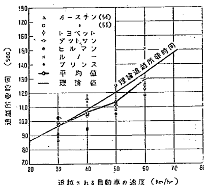
図—11 追越される自動車の速度と追越 所要時間の関係
