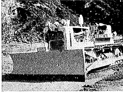
写真-1 D-120 アングルドーザ
