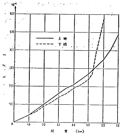
図一16 荷重とヒズミの関係
