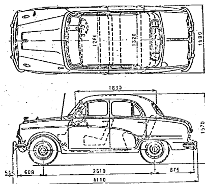
図-2.e オーステン・イングランド
