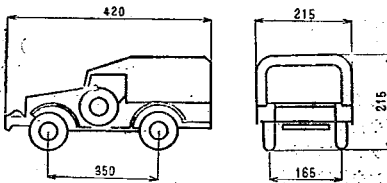
図-2.a ウェアポン・キャリア
