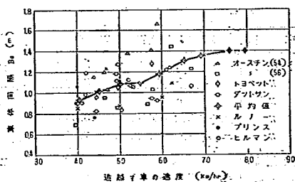
図-20 追越す車の速度と車体間隔の関係
