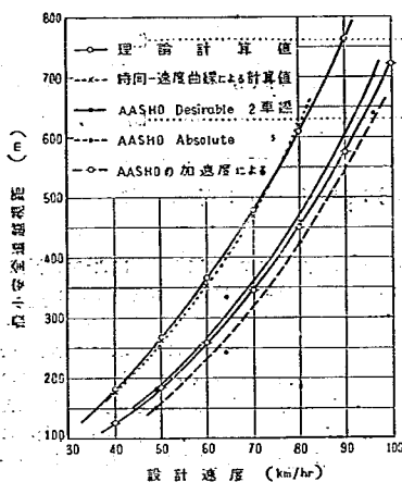
図-19 設計速度に対する最小安全追越視距 追越実験による方法について以下に記す。
