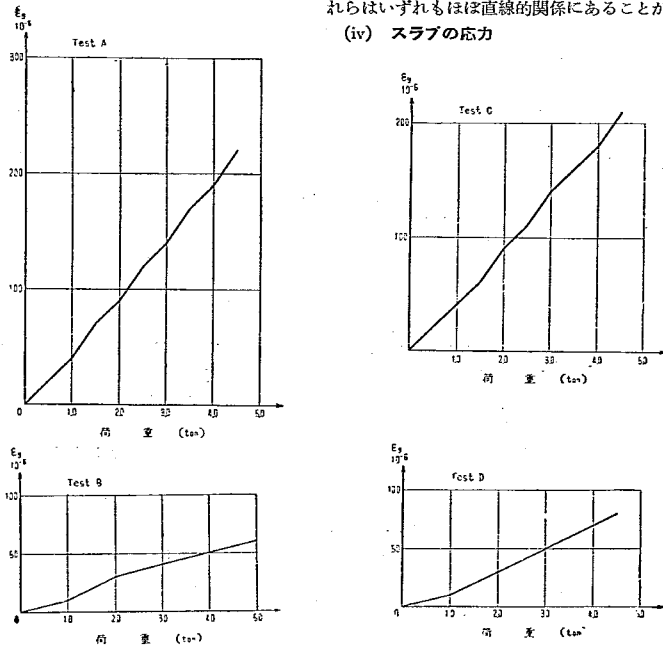
図-9 横方向のヒズミと荷重との関係
