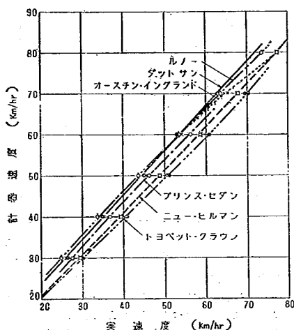
図-4 実速度と計器速度の関係
