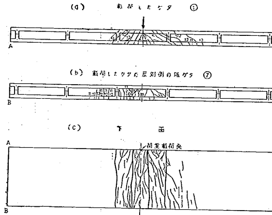
図-22 ひびわれの状況
