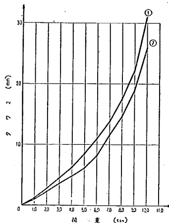
図-19 タワミと荷重との関係 (Test D 3 )
