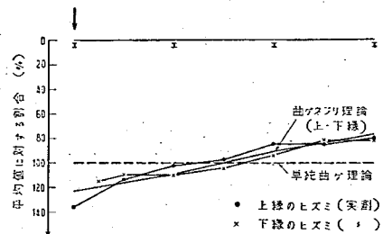
図-12 l/2 断面内における橋軸方向の応力の分布
