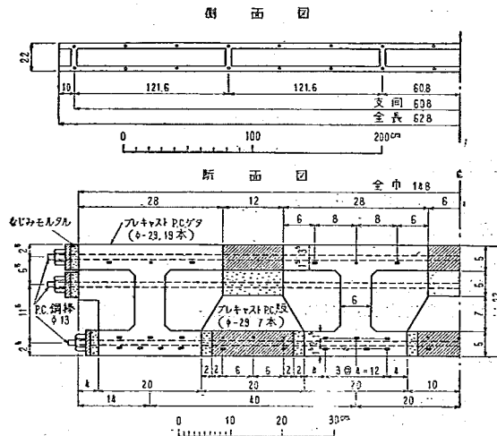
図-2 実験ゲタの断面寸法
