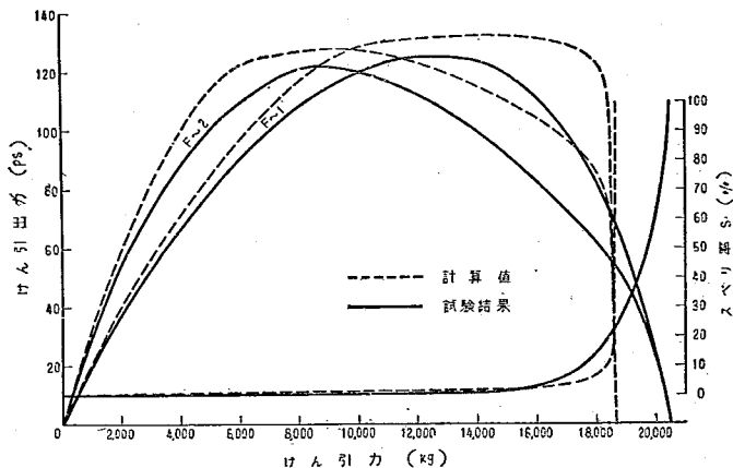
図-17 けん引出力の比較 (トルコン付)
