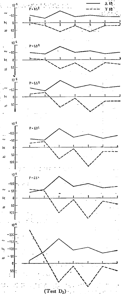
図一17 1/2断面内の横方向のヒズミの分布
