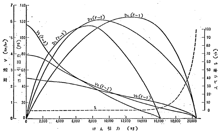
図-13 けん引試験特性図 (トルコン付)
