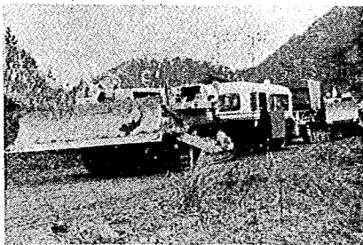
写真-2 けん引試験の状況
