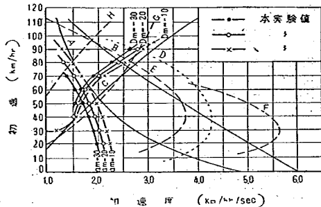
図-13 初速度と加速度の関係
