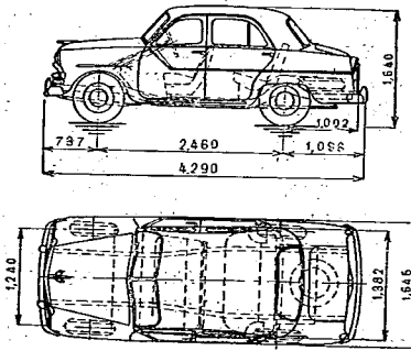
図-2.c プリンス・セダン
