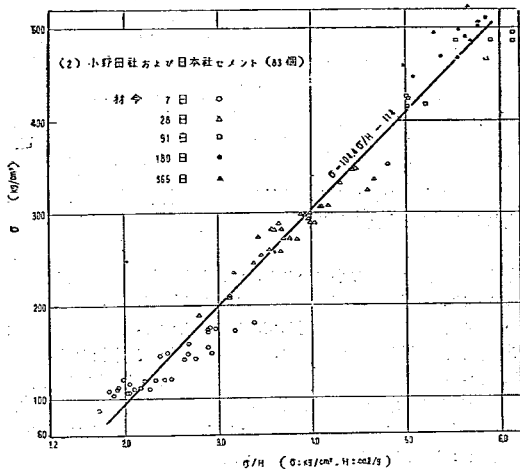
図-7 (2) \sigma - \sigma/H の関係
