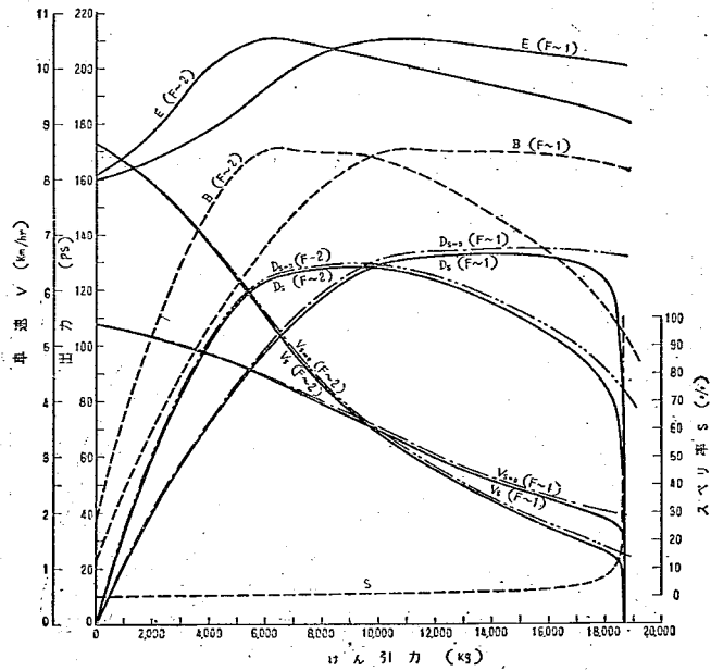
図-11 けん引特性図 (トルコン付)
