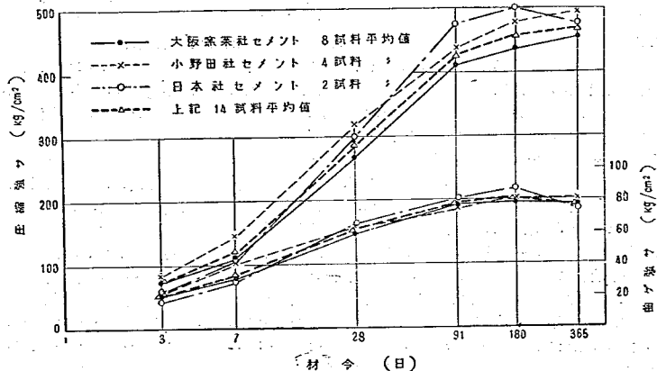
図-1 材令1年までの曲ゲおよび圧縮強さ
