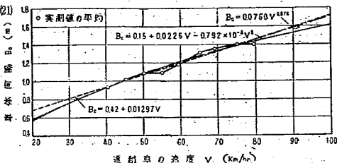
図-21 追越車の速度に対する車体間隔の曲線の当て嵌め
