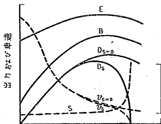
図-2 けん引特性図 (トルクコンバータ付)
