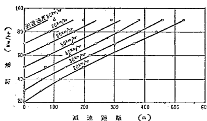
図-7 速度と減速距離
