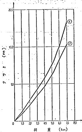
図-14 タワミと荷重の関係 (Test D 2 )
