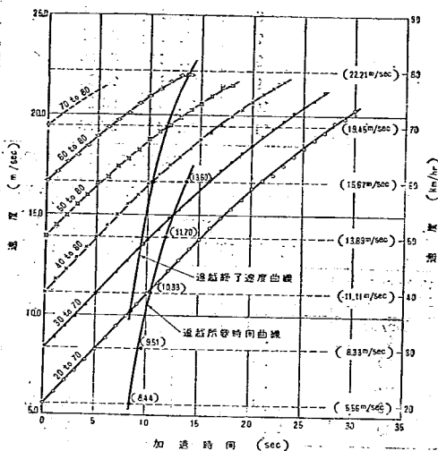
図-17 加速時間と速度との関係
