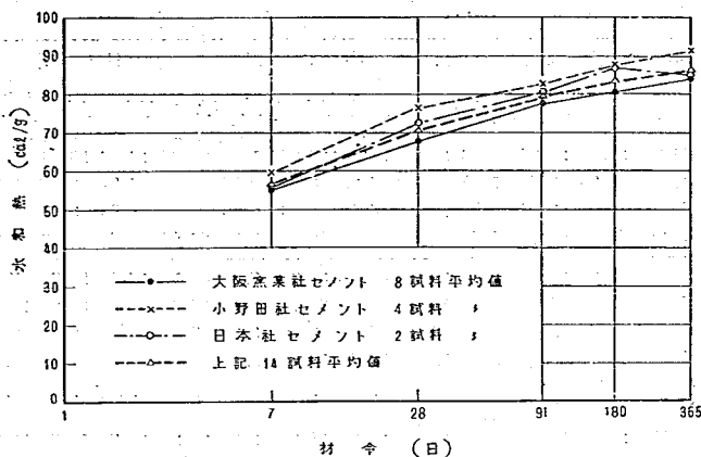
図-2 材令 1 年までの水和熱
