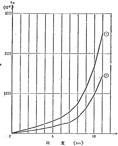
図-21 橋軸方向のヒズミと荷重との関係 (Test D 3 )
