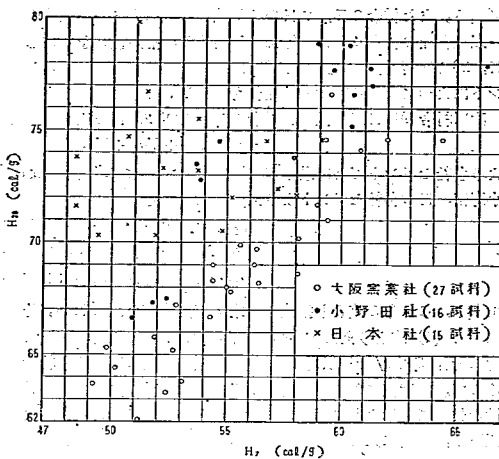
図-6 水和熱 ( H_7 , H_{28} ) 間の関係
