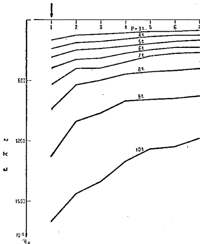
図-20 1/2断面内における橋軸方向のヒズミの分布 (Test D 3 )
