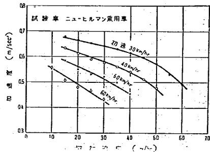
図-14 異なる初速度と増加加速度に対する加速度の関係
