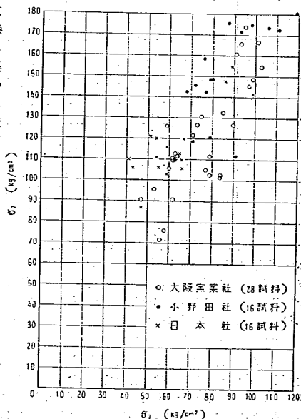
図-4 圧縮強サ ( \sigma_3 , \sigma_7 ) 間との関係
