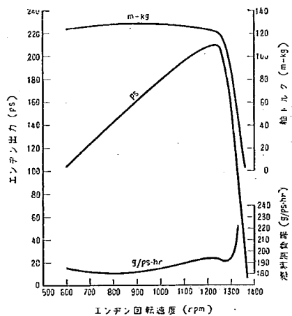
図—7 DE 型エンジン性能曲線 (トルコン付 D-120 登載)
