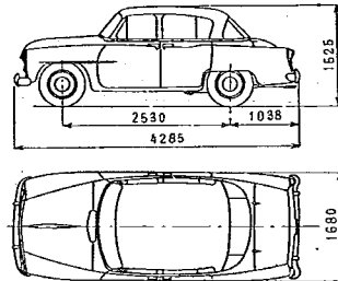
図-2.b トヨベツト・クラウン
