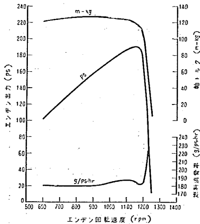
図—6 DE 型エンジン性能曲線 (メカニカルトランスミッション付 D-120 登載)
