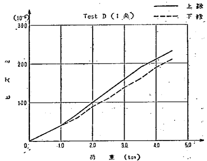
図-7 荷重載荷点の橋軸方向のヒズミ ( \epsilon_x ) と荷重の関係
