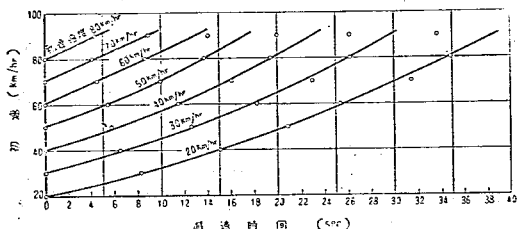
図-8 速度と減速時間
