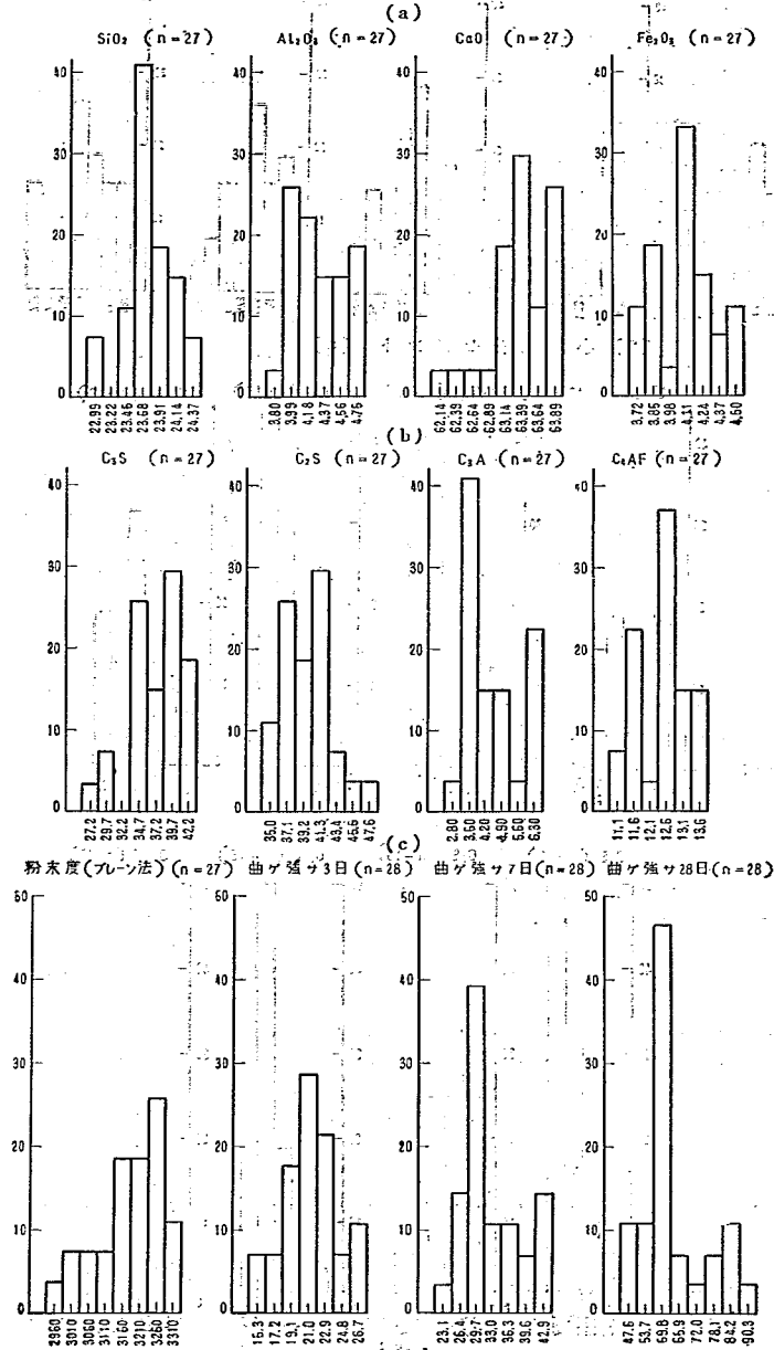
図-3 セメント諸性質のヒストグラム
