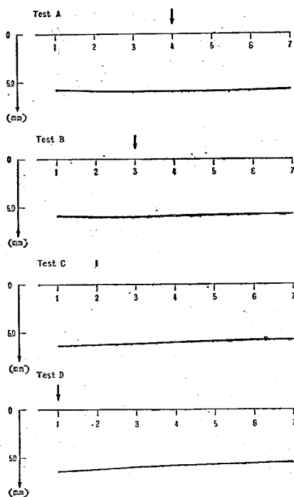
図—4 1/2 断面内のタワミ (Test A, B, C, D)
