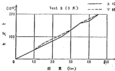
図-7 荷重載荷点の橋軸方向のヒズミ ( \epsilon_x ) と荷重の関係
