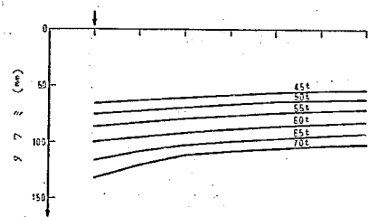
図-13 l/2 断面内のタワミ分布 (Test D_2 )
