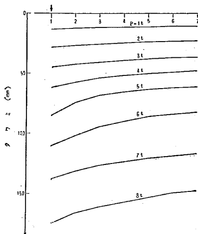
図-18 l/2 断面内におけるタワミの分布 (Test D 3 )
