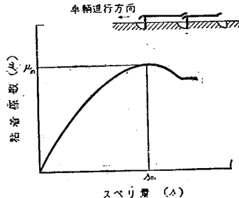
図-18 履板の粘着特性図
