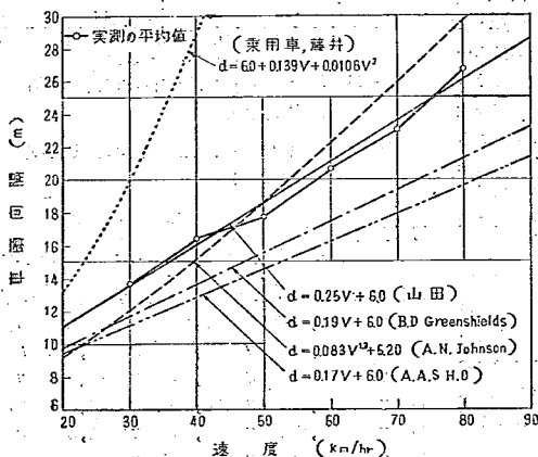
図-16 速度と車頭間隔の関係
