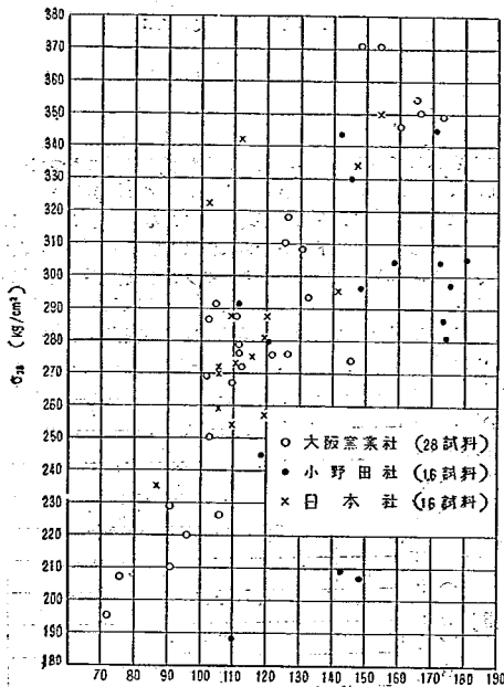
図-5 圧縮強サ ( \sigma_7 , \sigma_{28} ) 間の関係
