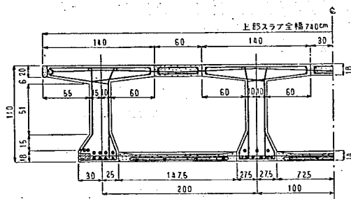
図-1 実橋の断面図 (1/2 断面)
