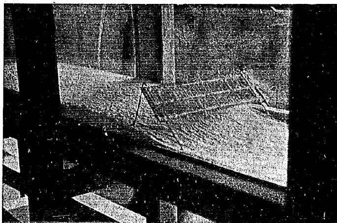
写真—3.2 45 型吹払い櫓の防雪効果, 風洞模型実験, 向つて右が風下側
