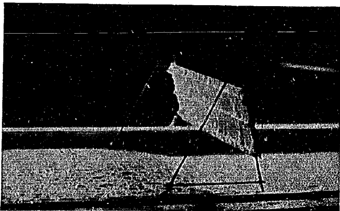
写真—3.5 75 型吹払い柵の防雪効果，風洞模型実験，向つて右が風下側
