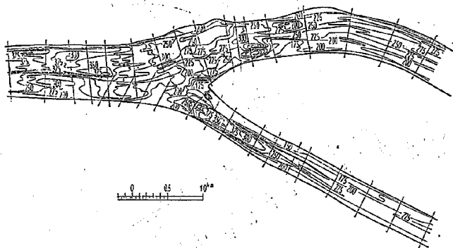
図-15 A-III 14,000 m³/s 流速分布
