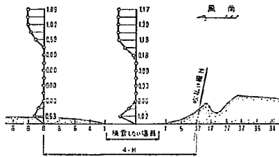
図-3.11 傾斜角度 80° の効果, 基準平均風速 6 m/sec
