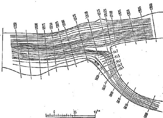
図—8・1 現況—14,000 m³/s 流況
