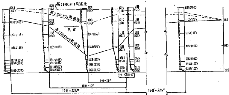
図—2.13 HS—150 型透過柵の防风効果，現地実験，10分間平均風速比分布
