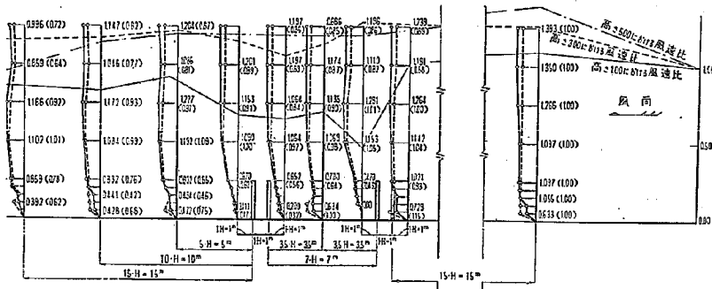
図—2.18 HS—100 2列2段型透過柵の防風効果，現地実験，5分間平均風速比分布
