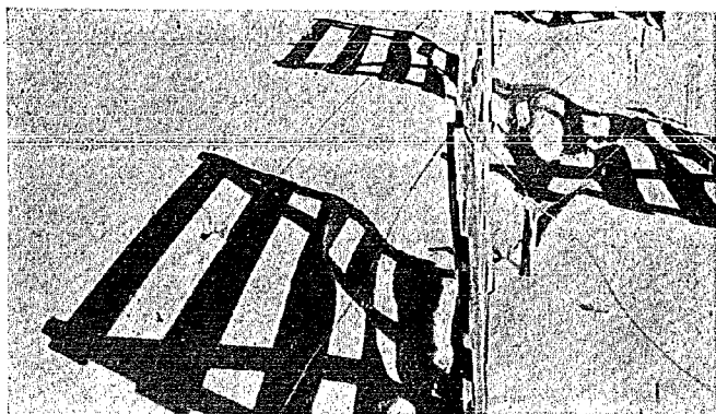
写真—2.14 HS-100 2列型 (HS-100 千鳥型) 透過櫓の防雪効果, 現地実験, 向つて左が風上側, 櫓の風上側に接近してできる吹溜り
