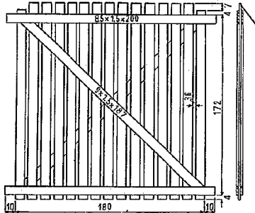
図-2.3 VS-180 型防雪柵透過率 28.5 %
