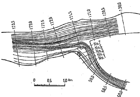
図-10-1 改修中間段階 14,000 \text{m}^3/\text{s} 流線
