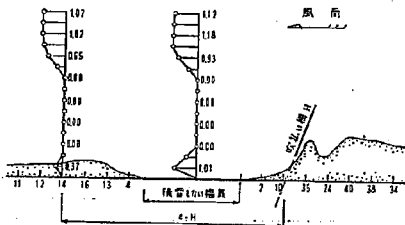
図—3.10 傾斜角度 70^\circ の効果，基準平均風速 6 m/sec
