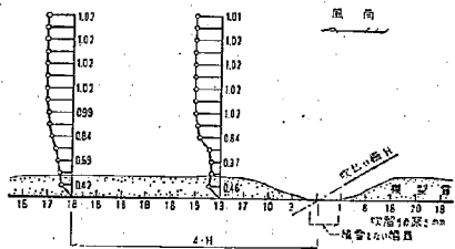
図—3.7 傾斜角度 30^\circ の効果，基準平均風速 6 m/sec
