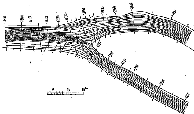
図-16 A-II 14,000 m³/s 流線
