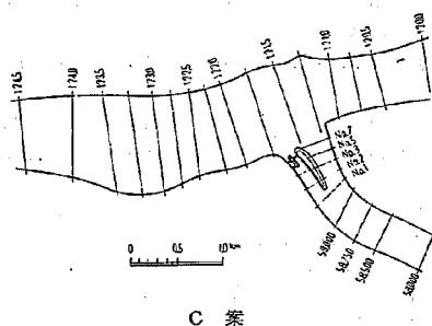
图一-11 各案平面图
