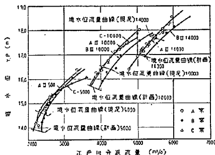
圖一12 A, B, C 3 案水位分派量相關圖
