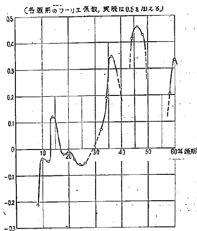
図—8. 京城最高月雨量の週期性傾向
