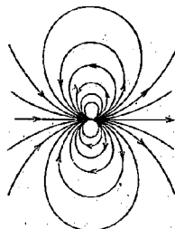
図4(b) 3次元2重わき出し
