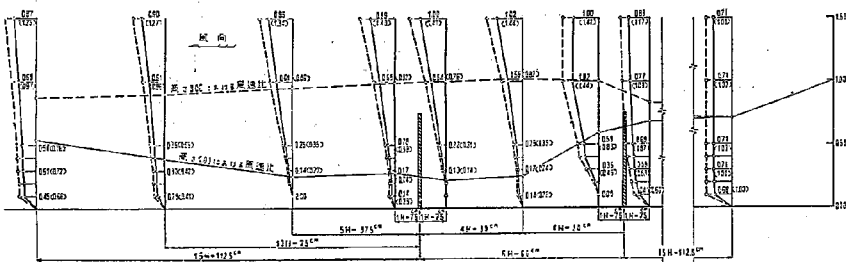
図—2.10 HS—150 2段型防風柵の防風効果風洞模型実験基準平均風速 8 m/sec
