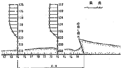
図-3.14 傾斜角度 110° の効果, 基準平均風速 6 m/sec
