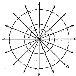
図4(a) 3次元のわき出し
