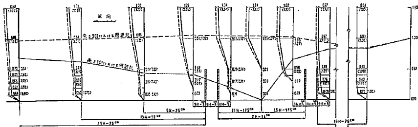
図-2.12 HS-100 2列2段型防雪柵の防風効果, 風洞模型実験, 基準平均風速 8 m/sec
