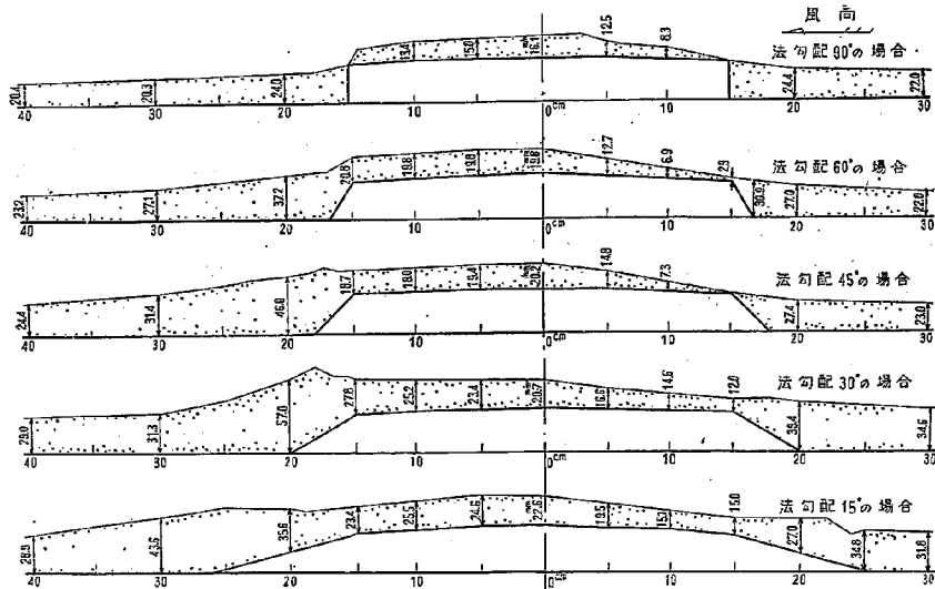
図-5.1 盛土路面形状の防除雪効果
