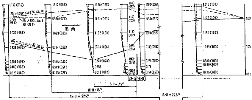
図-2.14 RHS-150 型透過柵の防風効果, 現地実験, 10 分間平均風速比分布
