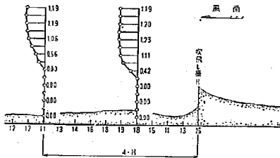
図-3.13 傾斜角度 90° の効果, 基準平均風速 6 m/sec
