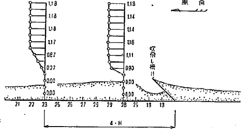
図-3.16 傾斜角度 135° の効果, 基準平均風速 6 m/sec
