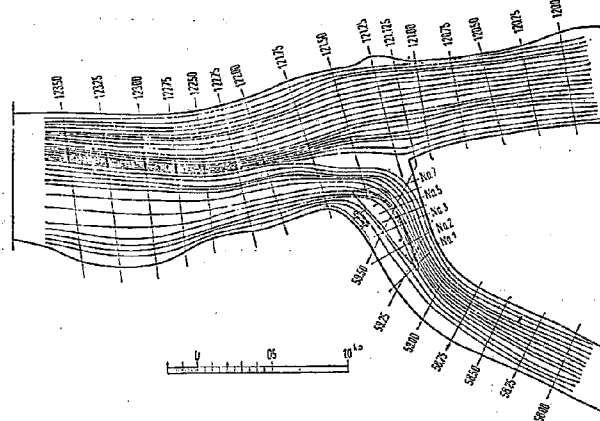
図-20 決定案 14,000 流域
