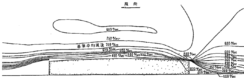
図-5.2 法勾配 90° の場合の風速分布
